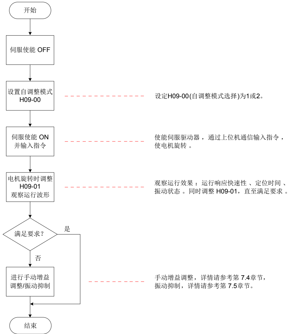
图 6-5 自动增益调整步骤
