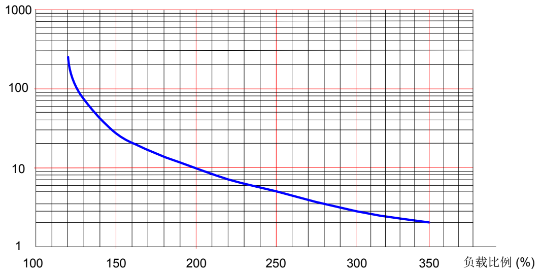
图 1-5 电机过载曲线
