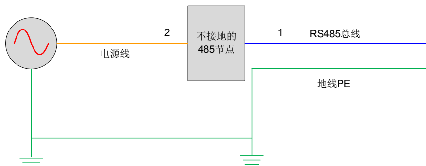
图 9-13 抑制外部干扰示意图
