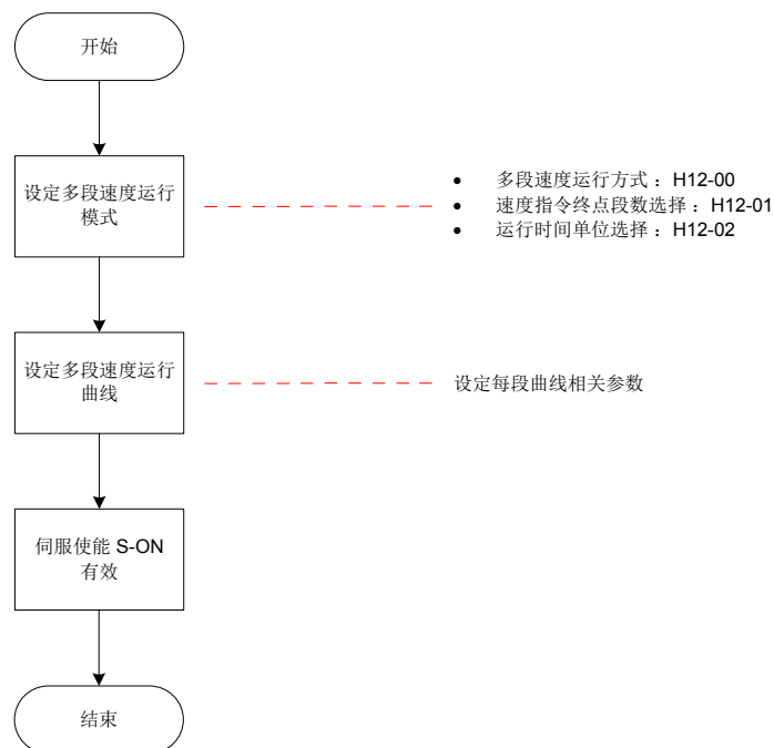
图 5-67 多段速度设置流程图
