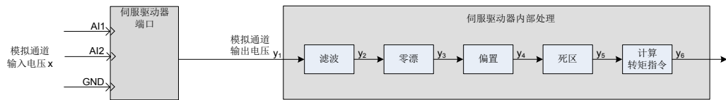
图 5-82 伺服驱动器 AI 处理流程
