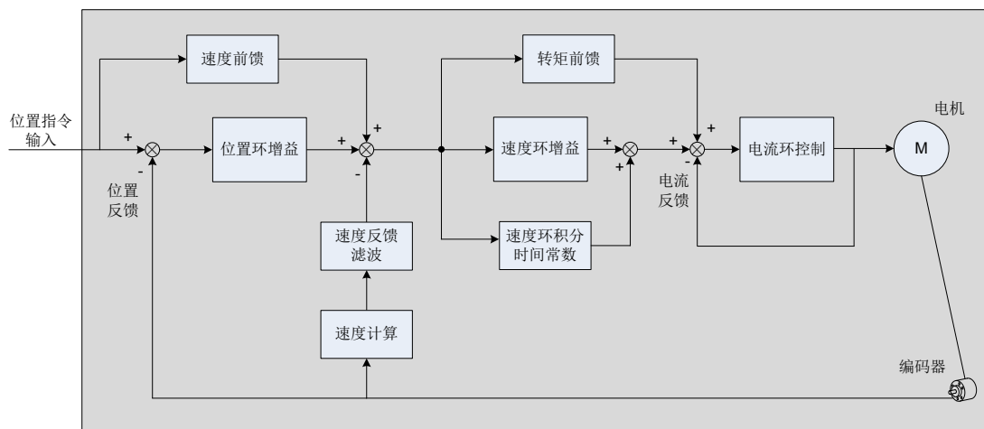
图 6-6 手动增益基本说明框图
