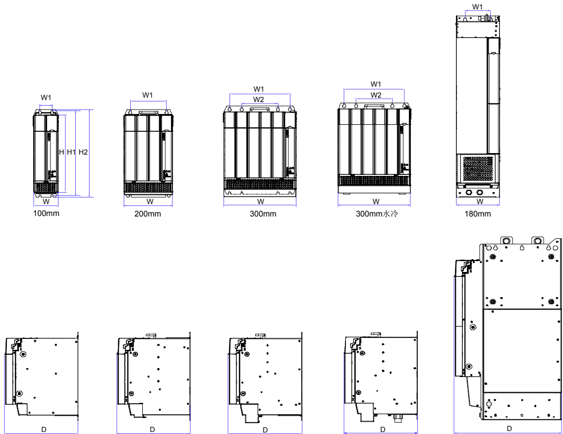
图 2-2 MD810-20M4T**G*** 外型尺寸示意图
