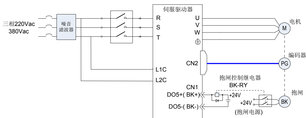
图 5-4 抱闸配线图
