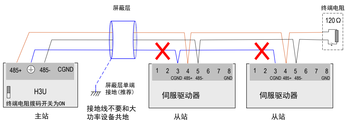
图 3-29 错误的 485 连接方法
