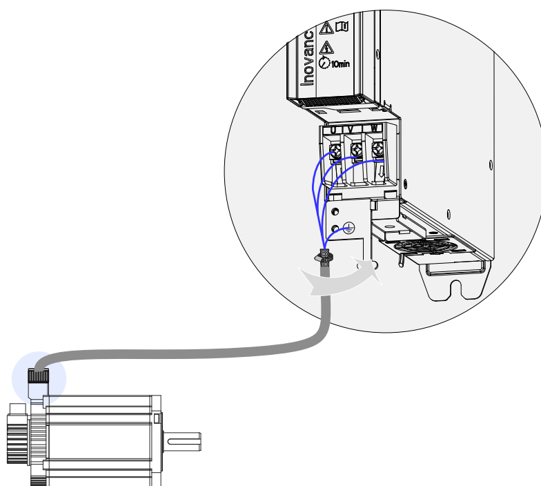
图 3-6 伺服驱动器输出与伺服电机连接举例
