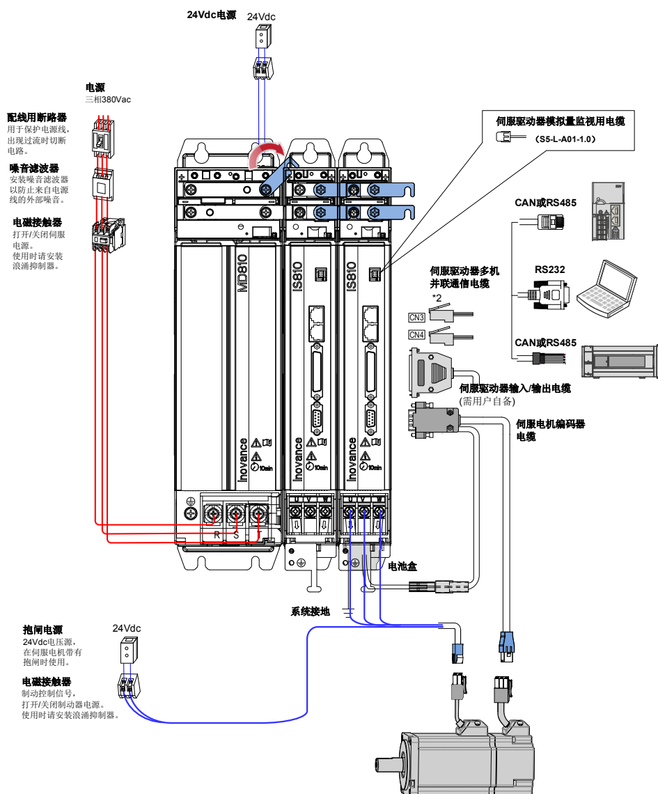
图 1-8 三相 380V 系统配线图举例
