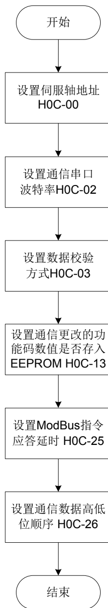
图 9-9 通信参数设定流程
