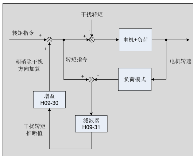
图 6-12 扰动观测功能框图
