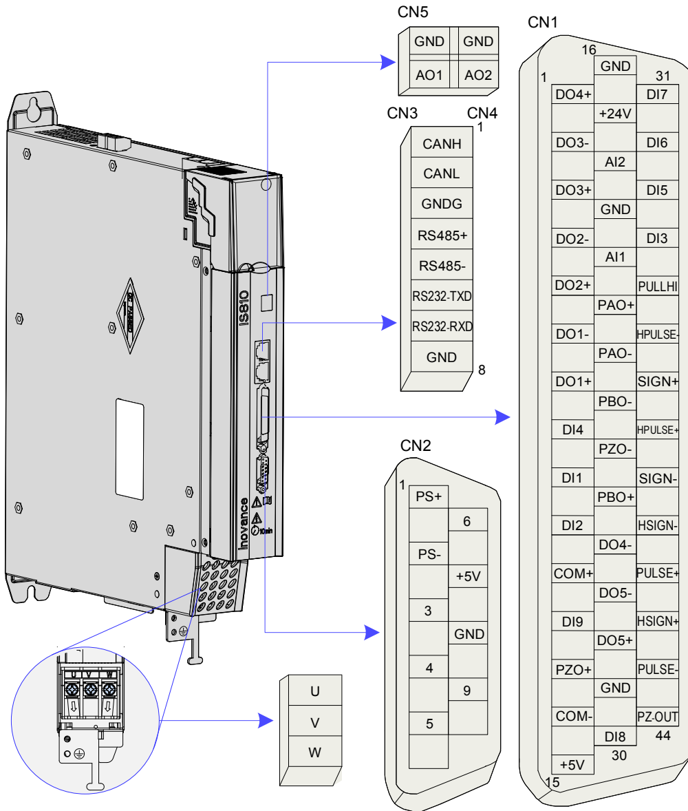
图 3-1 逆变单元端子引脚分布图
