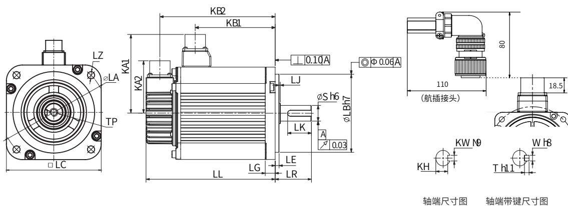
轴端尺寸图 轴端带键尺寸图
