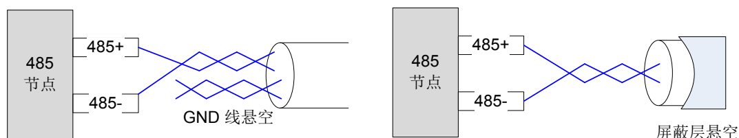
图 9-11 无 GND 时的接线示意图
