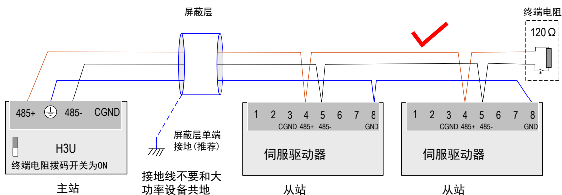
图 3-28 正确的 485 连接方法
