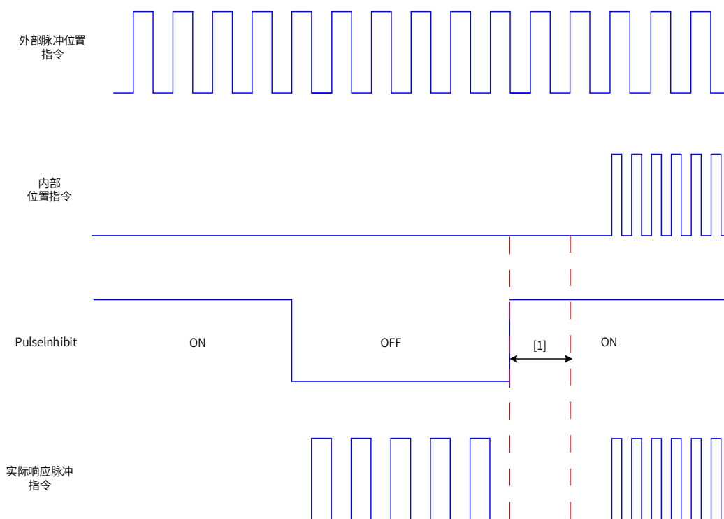
图 5-28 脉冲指令禁止功能波形举例
