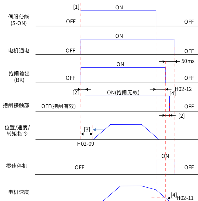
图 5-6 电机旋转时抱闸时序图
