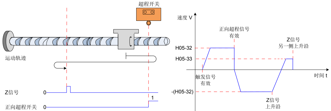
图 5-45 模式 2 原点回零电机运行曲线③与转速说明
