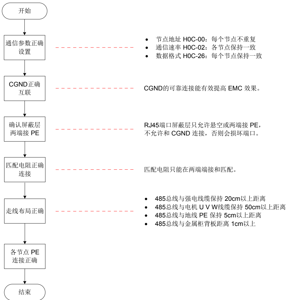
图 9-15 485 通信现场问题定位流程图
