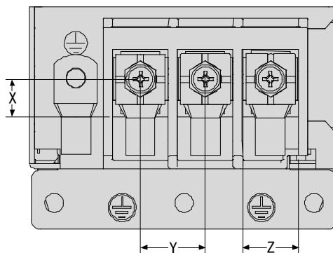
图 3-2 端子台示意图
