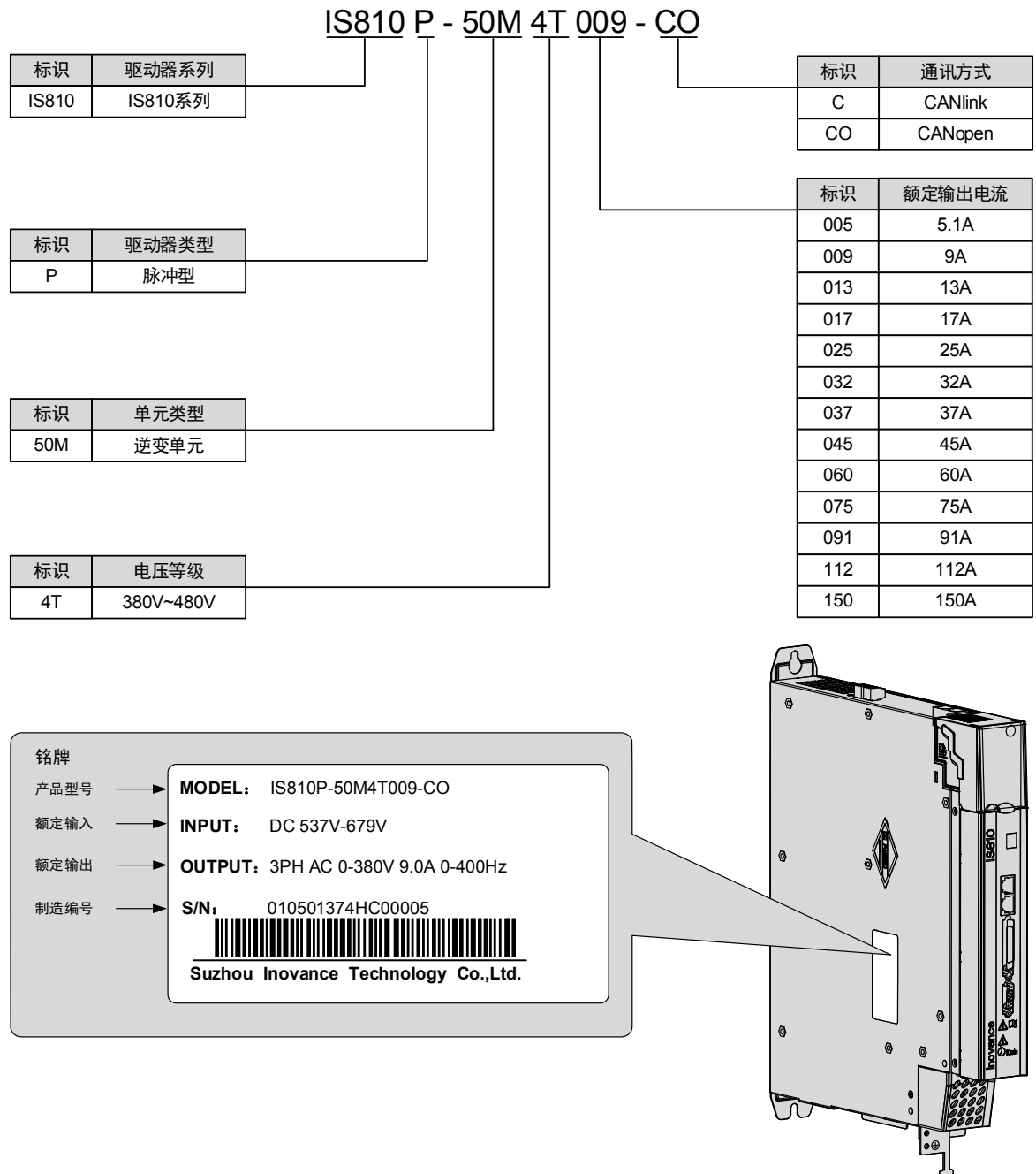
图 1-1 逆变单元型号与铭牌说明
