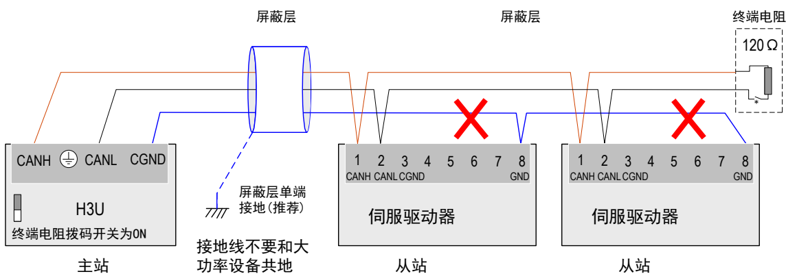
图 3-25 错误的 CAN 连接方法
