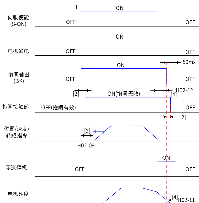
图 3-20 电机旋转时抱闸时序图
