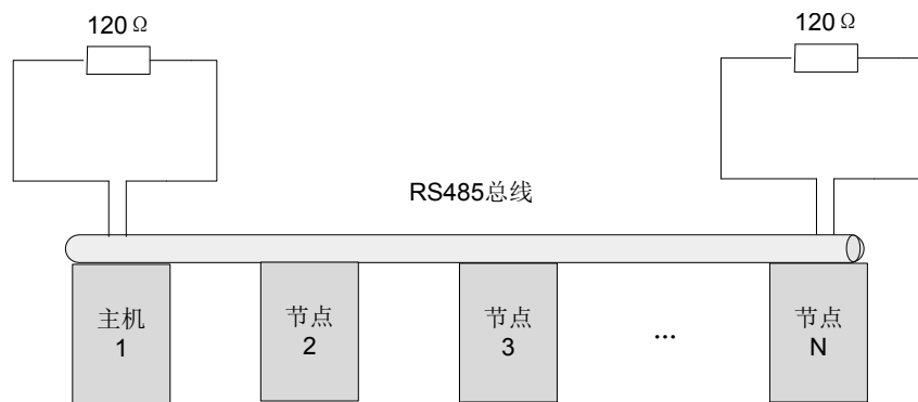
图 9-10 终端电阻接入方式示意图
