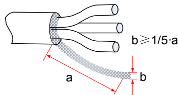
图 3-12 电机电缆屏蔽层引出示意图
