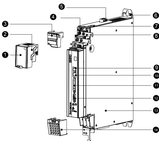
图 1-3 逆变单元组成说明
