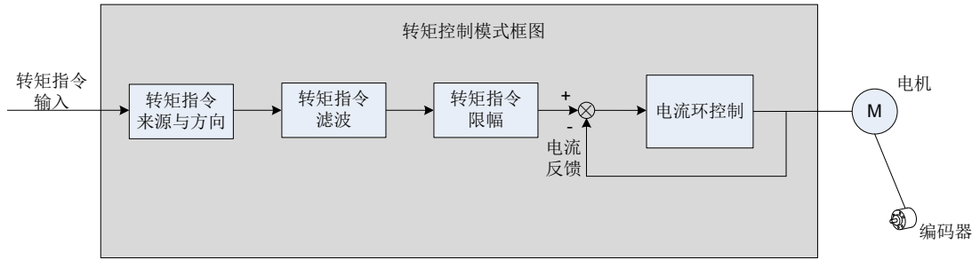
图 5-77 转矩控制框图
