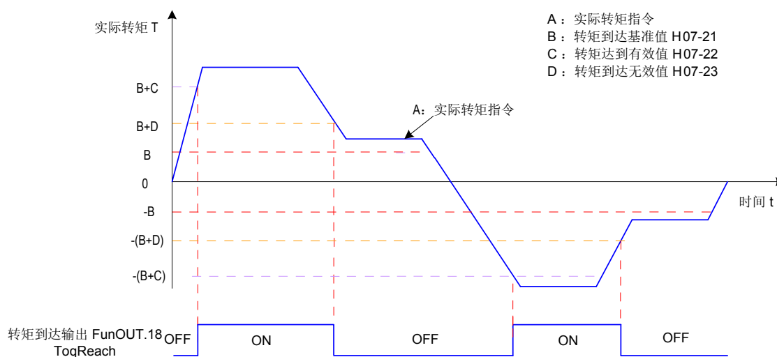
图 5-98 转矩到达输出波形举例
