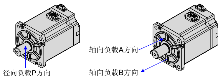
图 1-6 电机径向及轴向负载示意图
