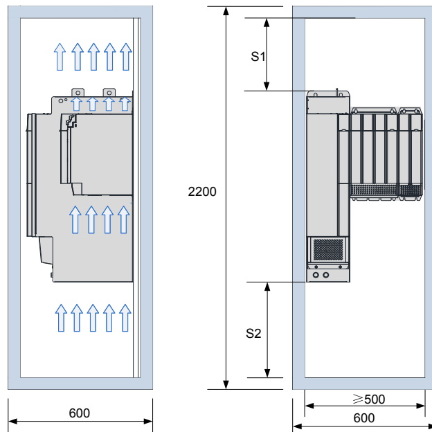
图 2-7 立式整流单元双层安装空间
