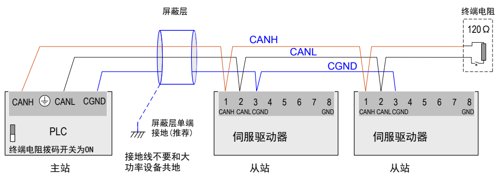
图 9-16 CANlink 接线示意图
