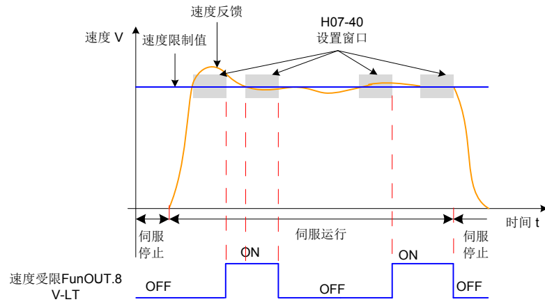
图 5-97 速度限制 DO 输出波形举例
