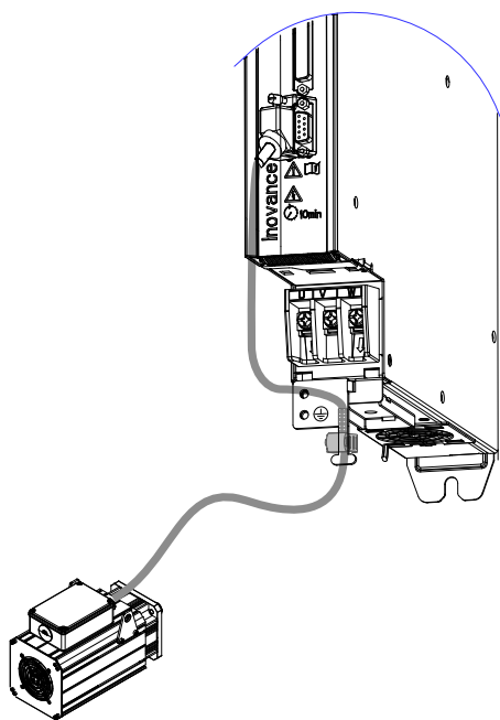
图 3-13 编码器信号接线示例图
