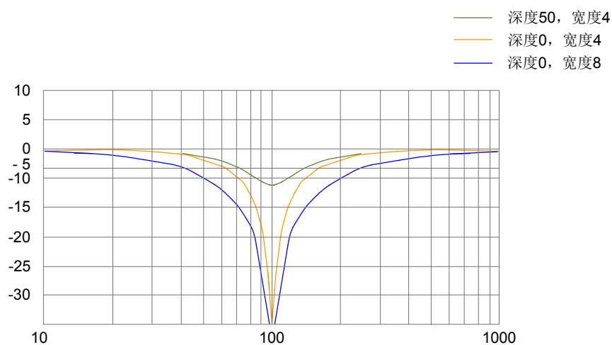
图 6-15 陷波器频率特性
