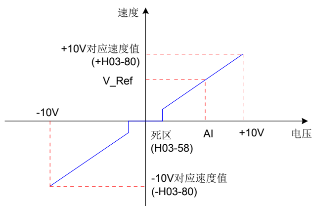
图 5-64 无偏置 AI 示意图
