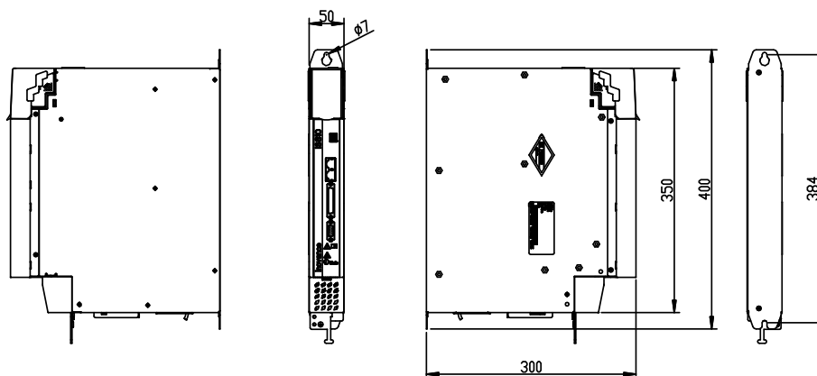
图 2-3 IS810P50M4T***** (SIZE 1) 外形尺寸图
