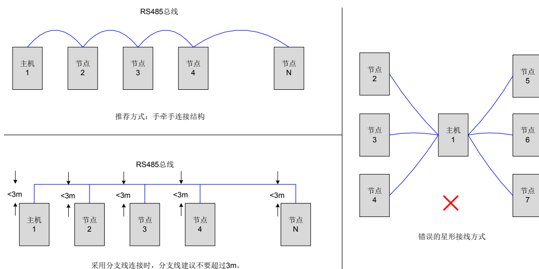
图 9-12 三种多节点连接方式示意图
