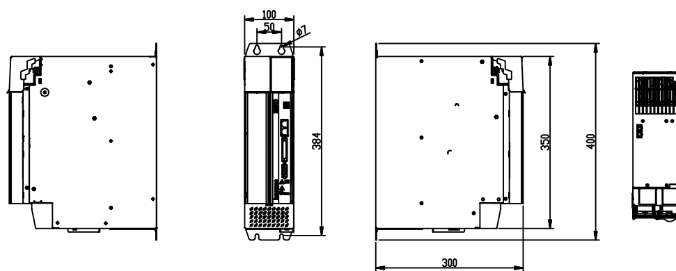
图 2-4 IS810P50M4T***** (SIZE 2) 外形尺寸图
