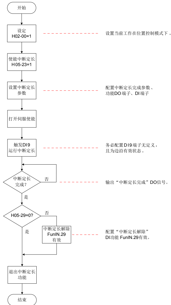
图 5-38 中断定长功能信号流程图
