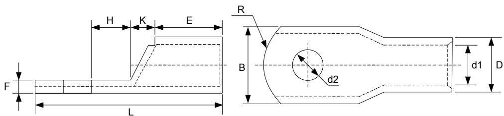
图 3-4 GTNR 系列线耳尺寸图
