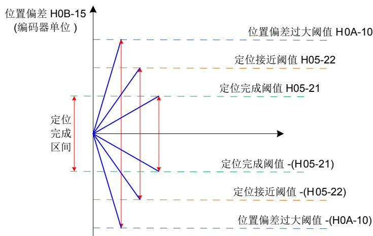
图 5-36 位置偏差相关信号
