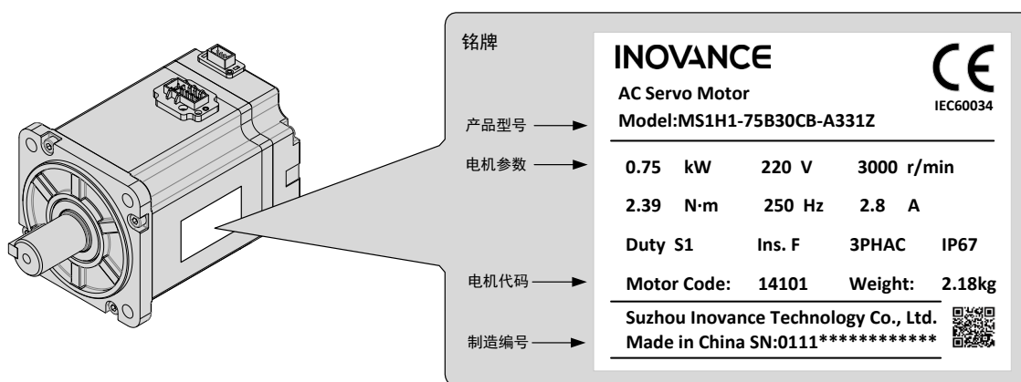
图 1-4 伺服电机型号与铭牌说明
