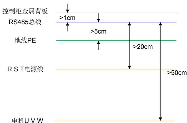
图 9-8 线缆布置示意图
