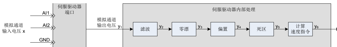
图 5-62 伺服驱动器 AI 处理流程
