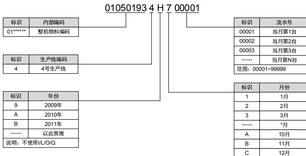
图 1-2 逆变单元生产序列号说明
