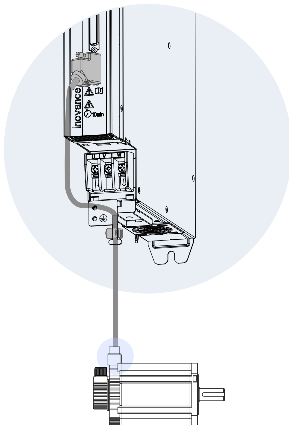
图 3-7 编码器信号接线示例图
