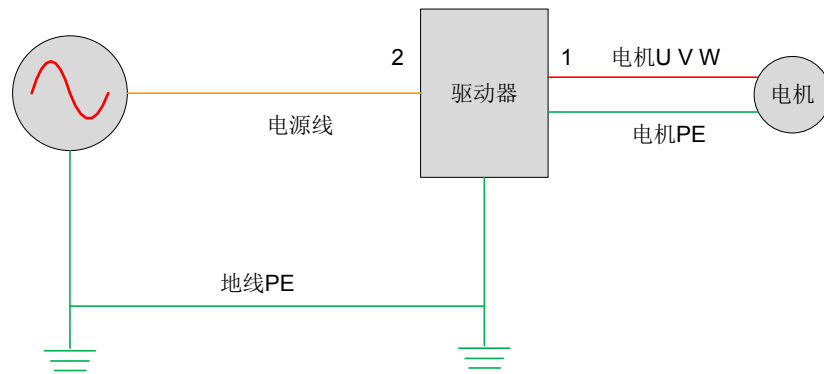
图 9-14 驱动器干扰抑制示意图
