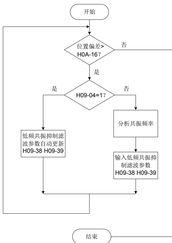
图 6-17 低频共振抑制滤波器使用步骤
