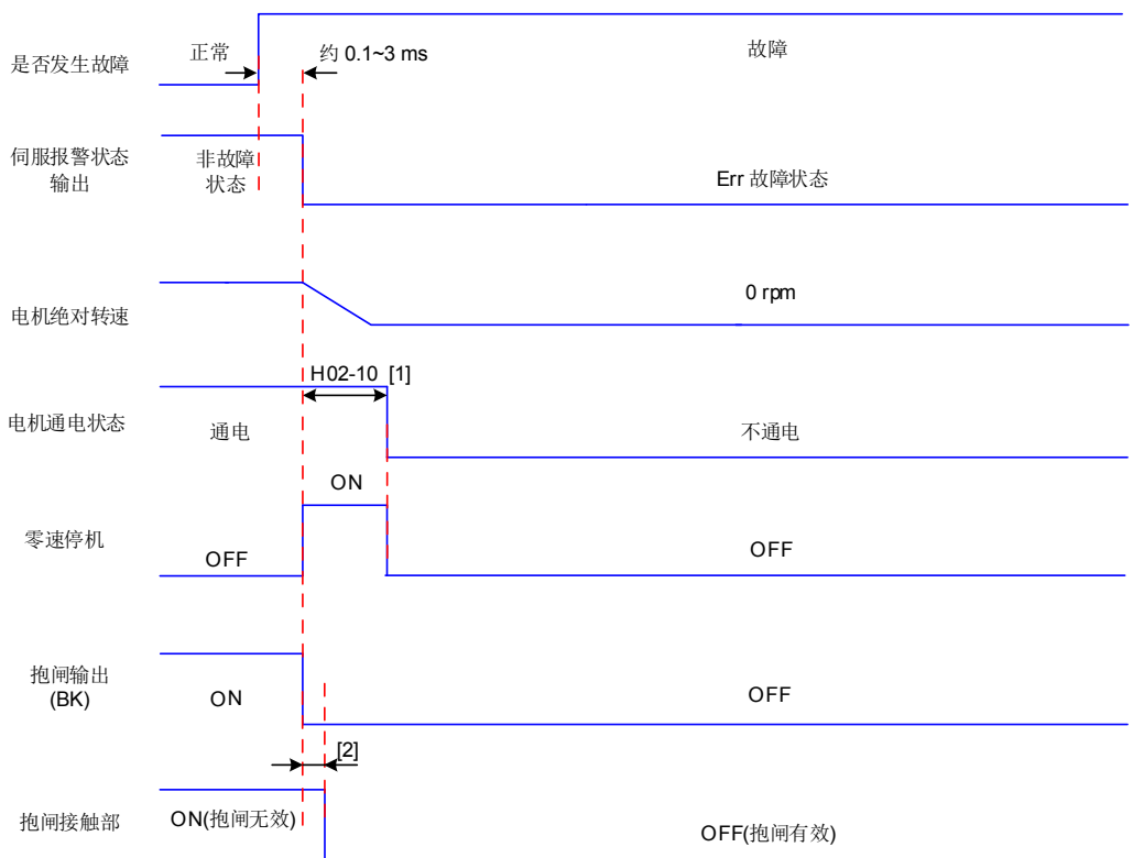
图 5-11 故障 2(带抱闸)时零速停机方式自由停机状态时序图
