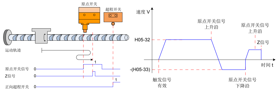
图 5-46 模式 4 原点回零电机运行曲线①与转速说明
