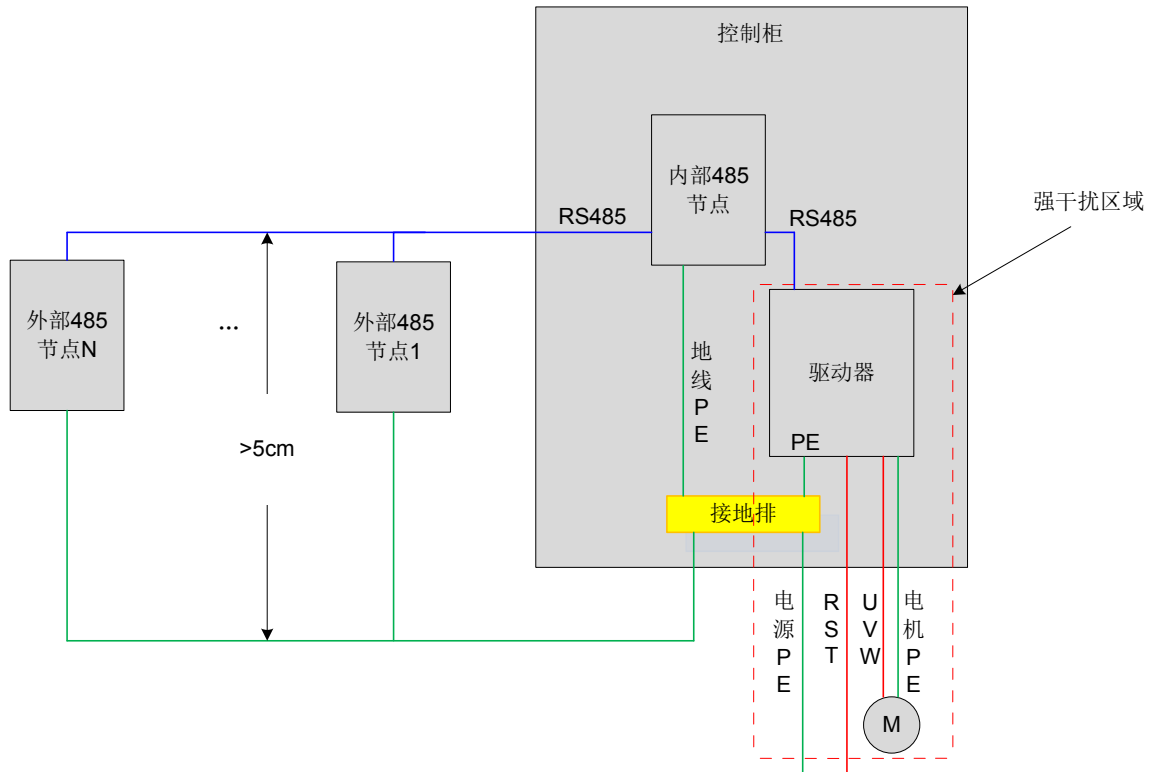
图 9-6 区域布置示意图
