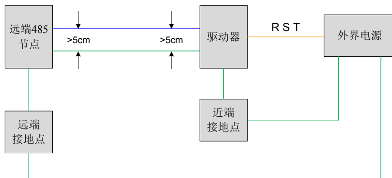
图 9-7 地线 PE 配线示意图
