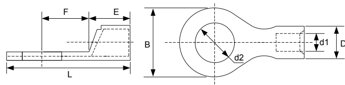
图 3-3 TNR 系列线耳尺寸图
