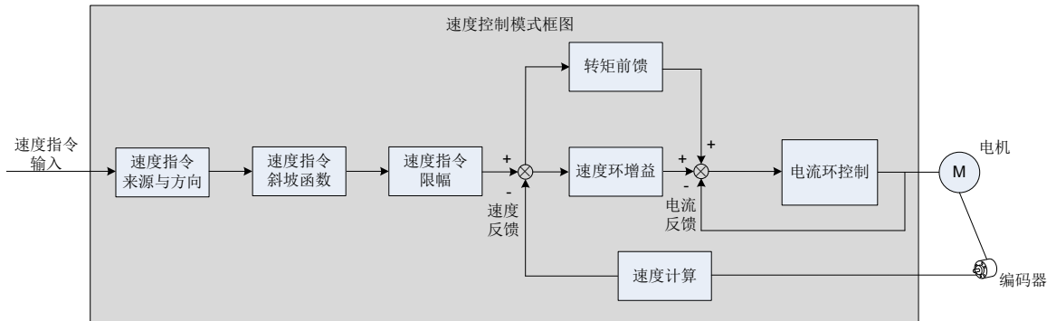
图 5-57 速度控制框图
