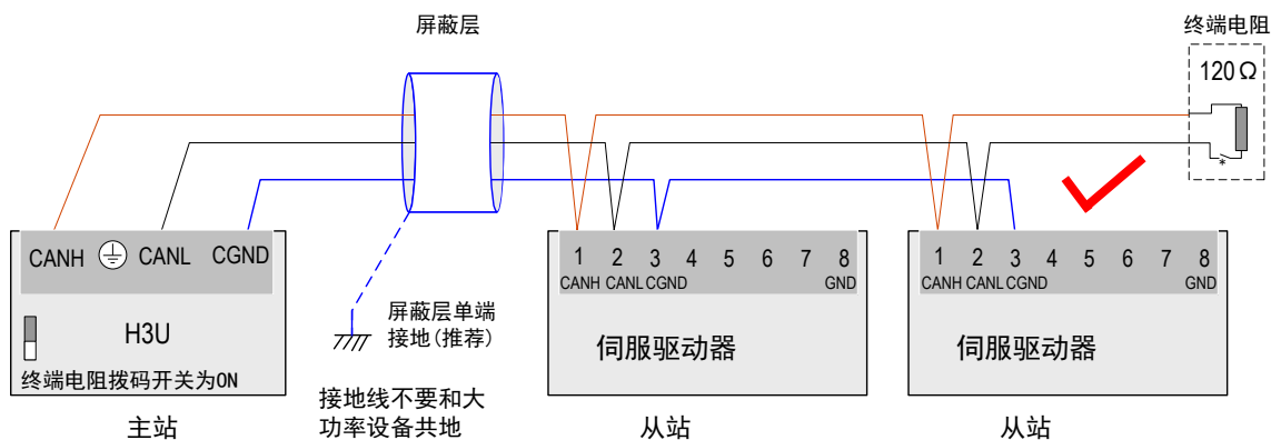
图 3-24 正确的 CAN 连接方法
