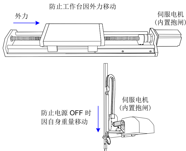
图 3-17 抱闸应用示意图
