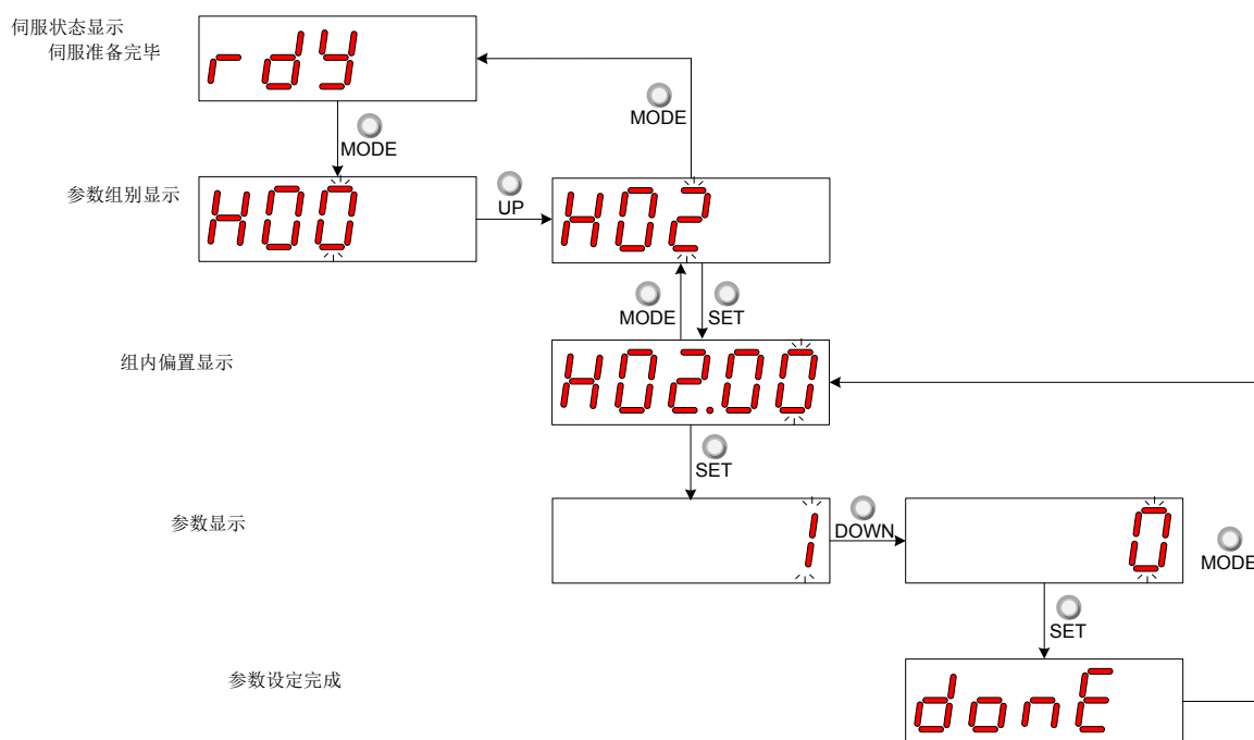
图 4-5 参数设定步骤示意图
