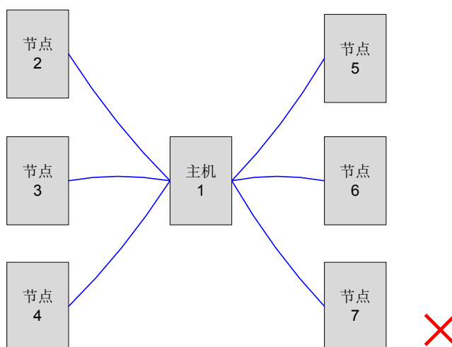
图 9-5 错误的星形接线方式
