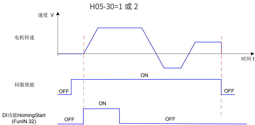
图 5-56 时序图举例
