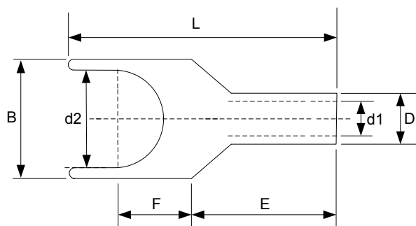
图 3-5 TNS 系列线耳尺寸图
