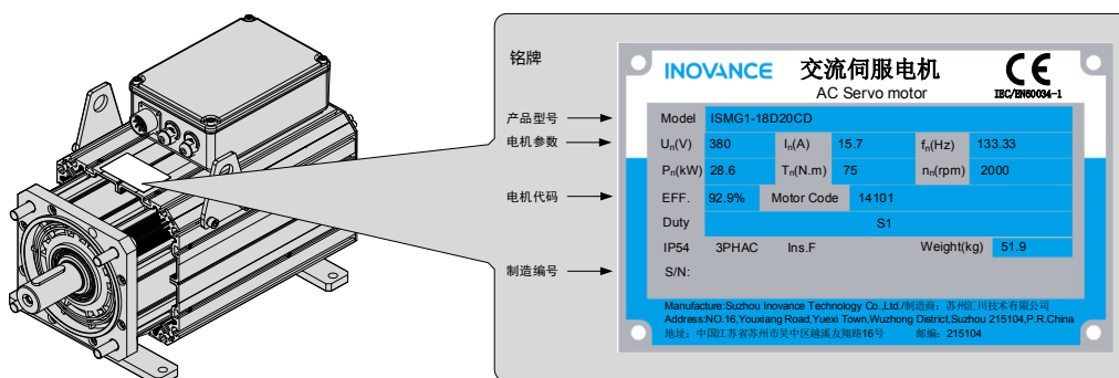
图 1-7 伺服电机型号与铭牌说明
