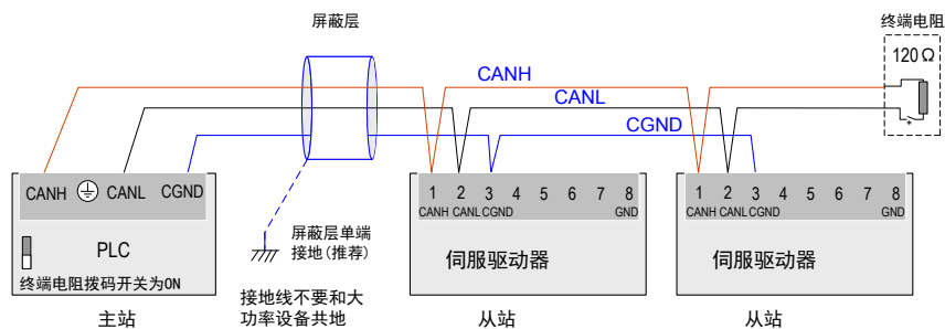
图 9-17 CANopen 连接示意图
