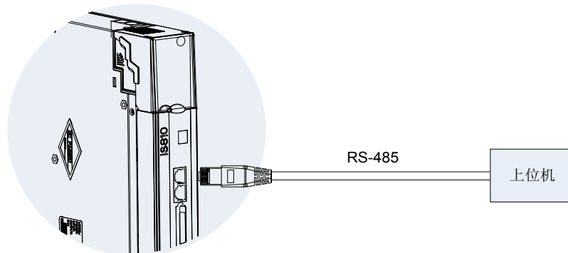
图 9-2 RS-485 连接示意图
