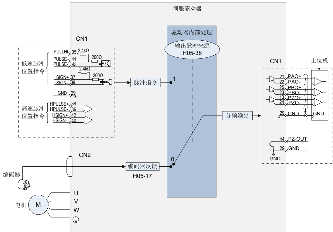
图 5-34 分频输出原理示意图
