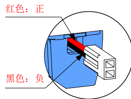
图 3-10 绝对值编码器电池外引线说明
