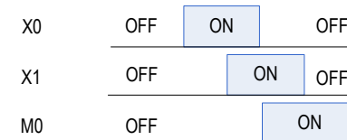
时序图
