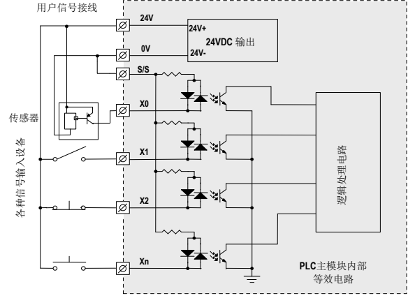
源型输入接法
