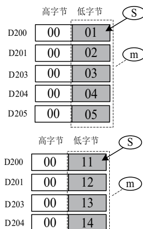
M8161=ON, 8bit 模式
