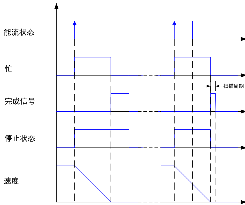
MCSTOP 时序图
