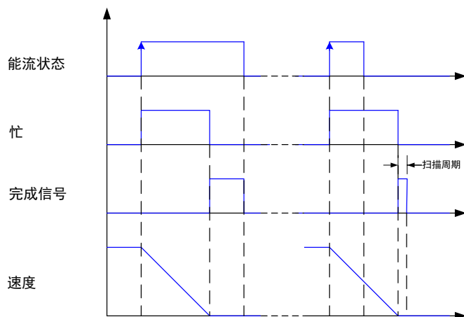
MCHALT 时序图
