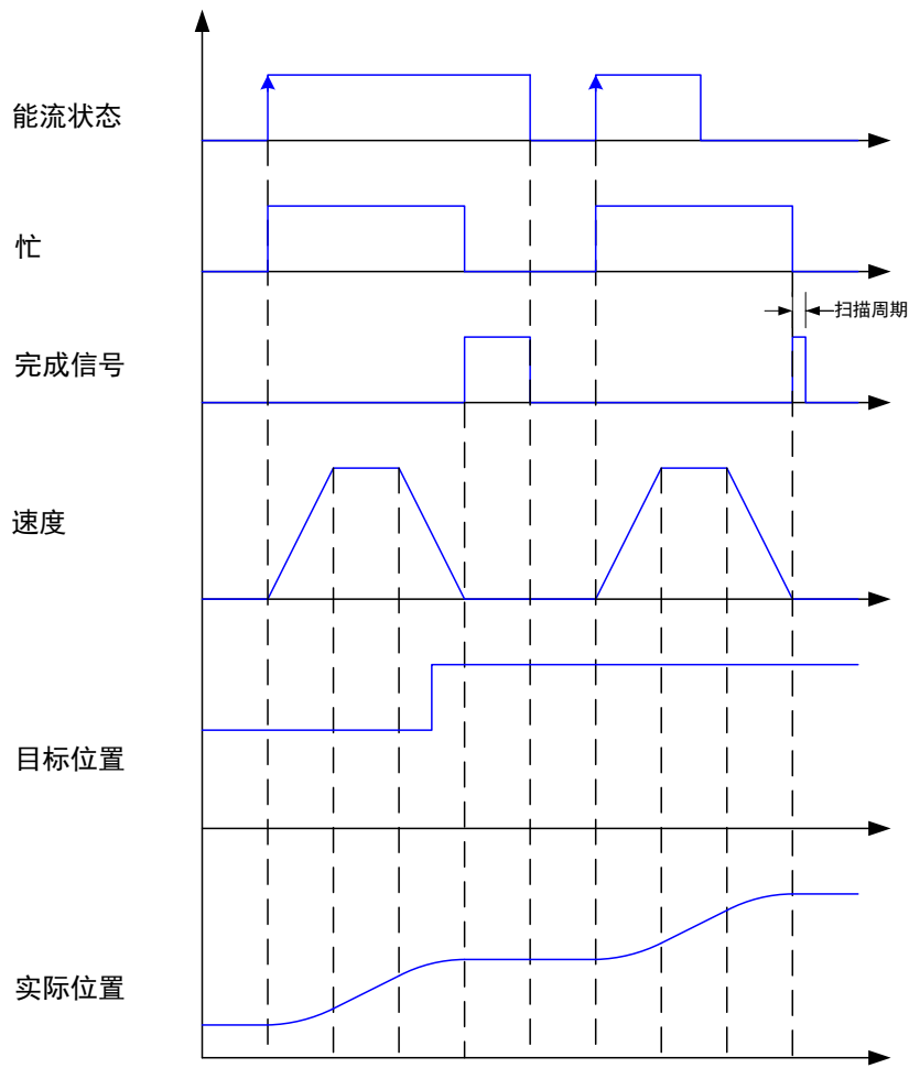
MCMOVABS 时序图
