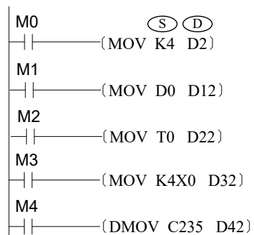
梯形图
