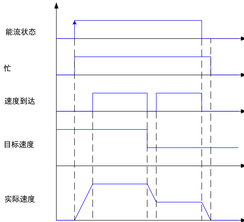
MCMOVVEL 时序图
