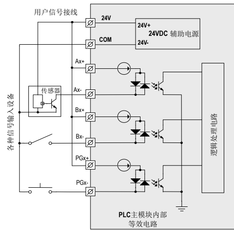
漏型输入
