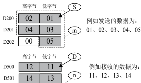
M8161=OFF, 16bit 模式
