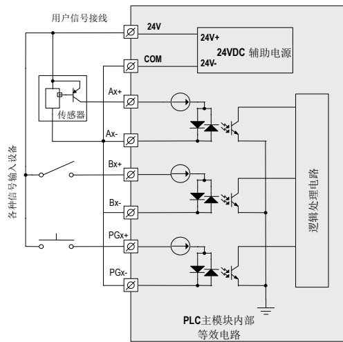
源型输入
