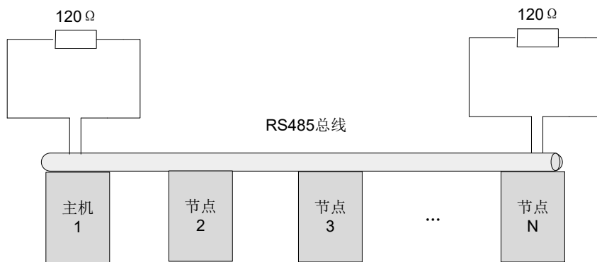
图 7-10 终端电阻接入方式示意图
