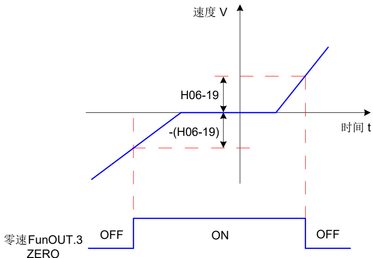
图 5-76 零速信号波形图
