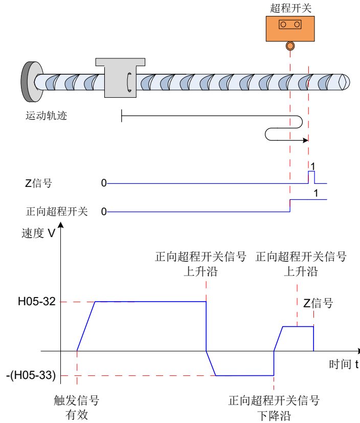
图 5-51 模式 8 原点回零电机运行曲线①与转速说明
