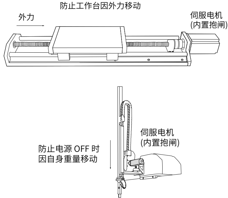
图 3-17 抱闸应用示意图
