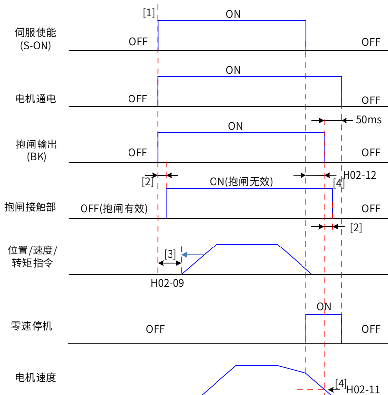
图 3-20 电机旋转时抱闸时序图
