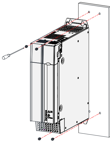
图 2-8 整流单元壁挂式安装示意图
