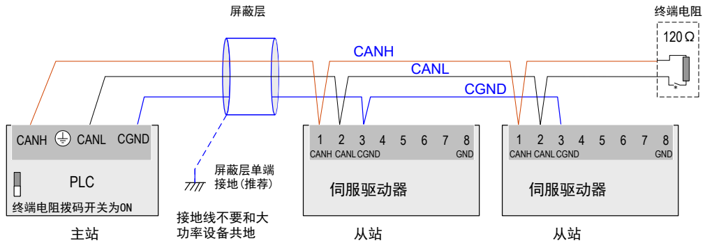
图 7-16 CANlink 接线示意图
