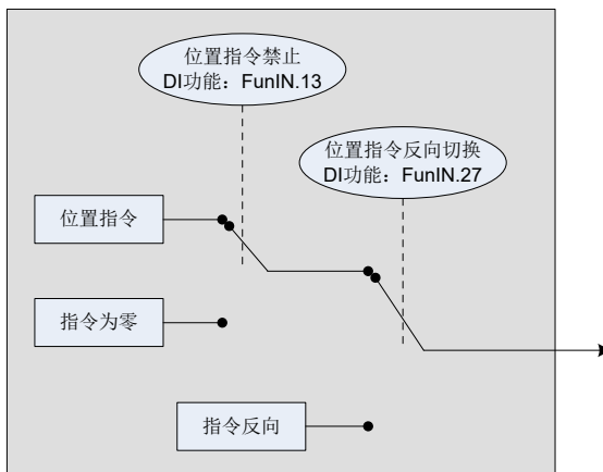
图 5-18 位置指令输入设置框图
