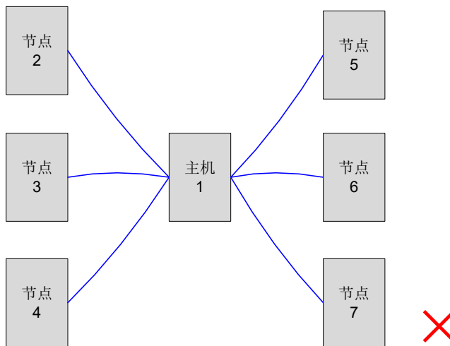
图 7-5 错误的星形接线方式
