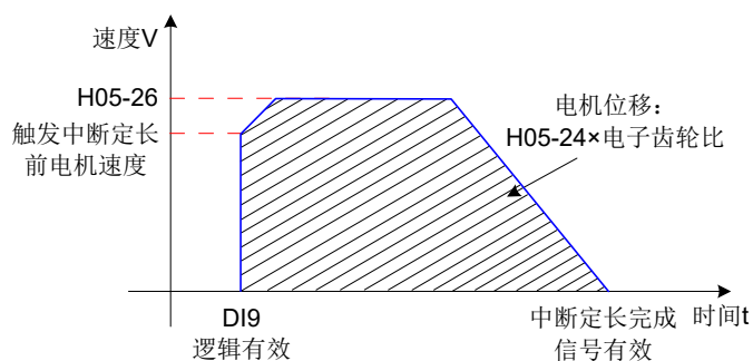
图 5-39 中断定长功能电机运行曲线
