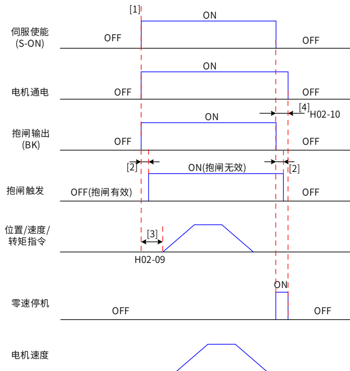
图 5-5 电机静止时抱闸时序图
