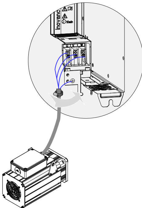
图 3-11 逆变单元输出与 ISMG 系列电机连接举例
