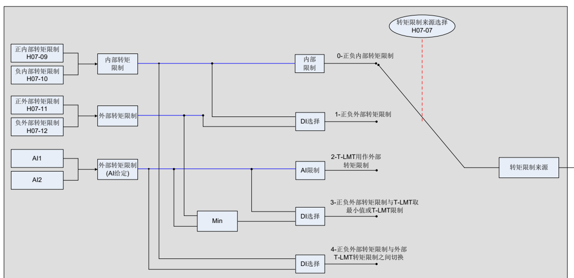
图 5-88 转矩限制来源
