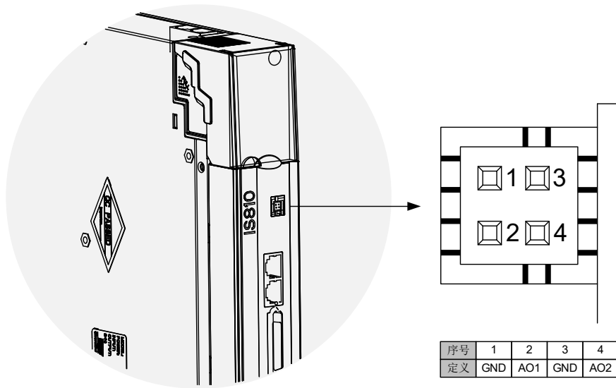
图 3-32 模拟量监视信号连接器端子
