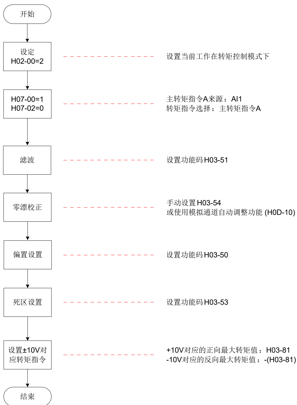
图 5-81 模拟量电压转矩指令操作流程
