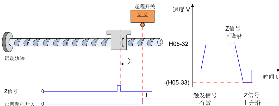
图 5-44 模式 2 原点回零电机运行曲线②与转速说明
