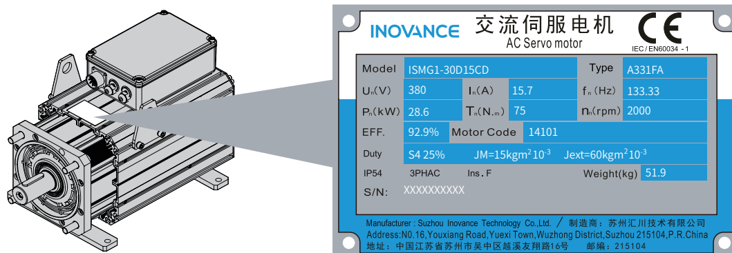
图 1-7 伺服电机型号与铭牌说明
