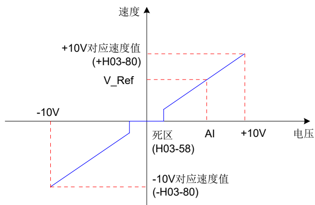
图 5-64 无偏置 AI 示意图
