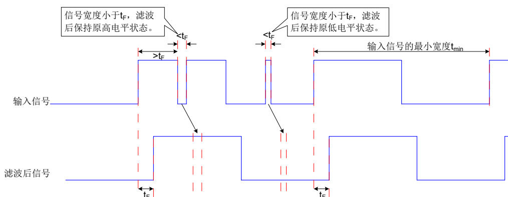
图 5-21 滤波信号波形举例
