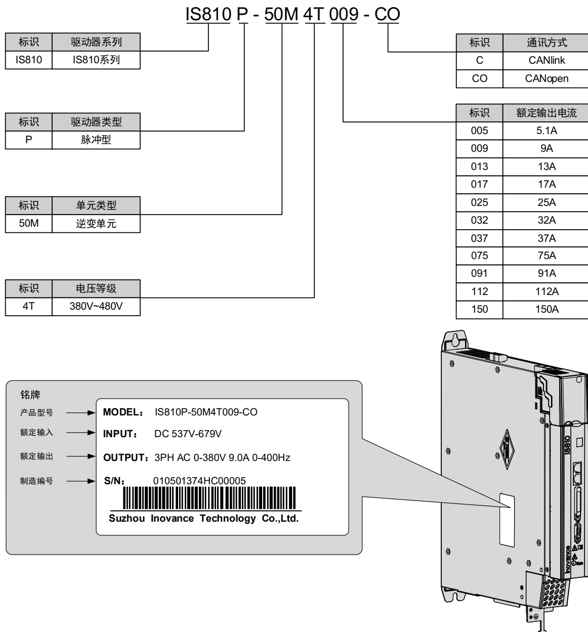
图 1-1 逆变单元型号与铭牌说明
