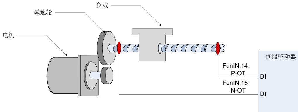
图 5-15 限位开关的安装示意图
