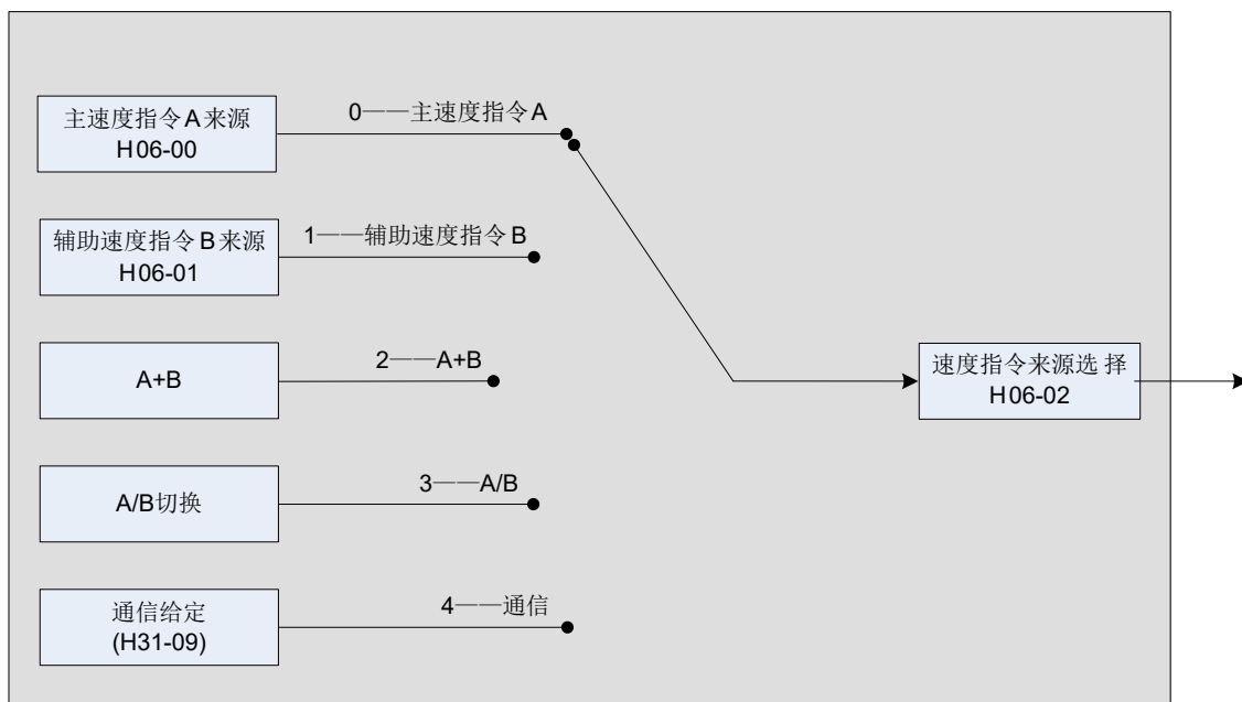
图 5-59 速度指令来源图
