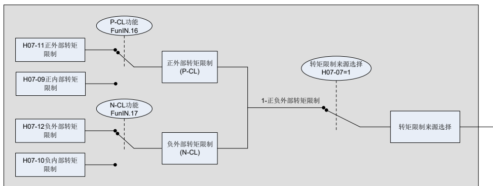
图 5-90 H07-07=1 转矩限制来源
