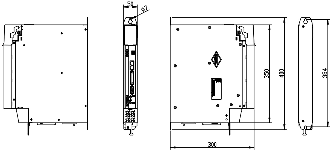
图 2-3 IS810P50M4T***** (SIZE 1) 外形尺寸图
