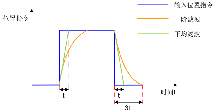
图 5-32 矩形位置指令一阶滤波与平均滤波示意图
