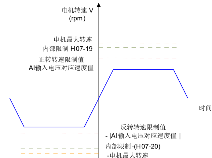
图 5-96 H07-17=1 速度限制曲线图
