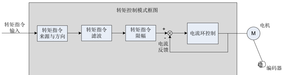
图 5-77 转矩控制框图
