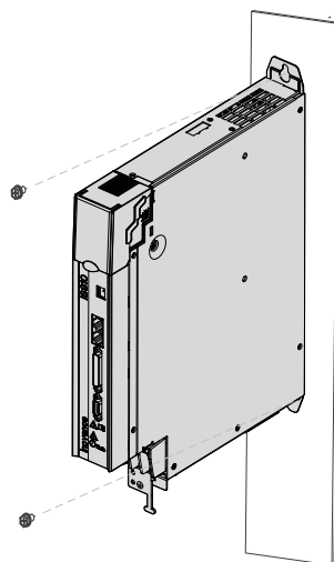
图 2-9 逆变单元壁挂式安装示意图
