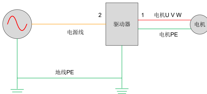
图 7-14 驱动器干扰抑制示意图
