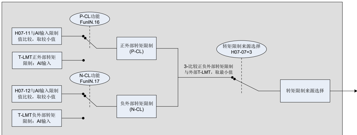
图 5-93 H7-07=3 转矩限制来源
