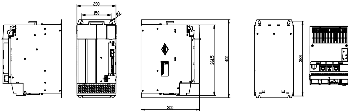
图 2-5 IS810P50M4T***** (SIZE 3) 外形尺寸图
