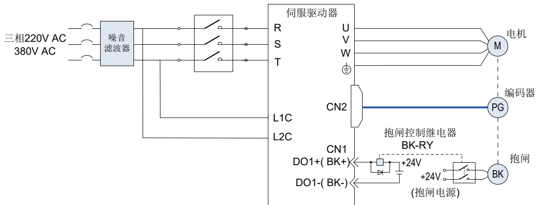
图 3-18 抱闸配线图
