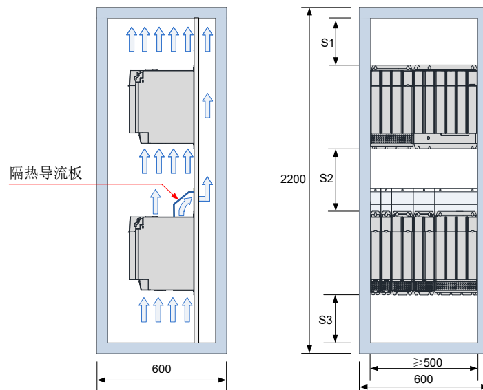
图 2-6 书本型整流单元双层安装空间
