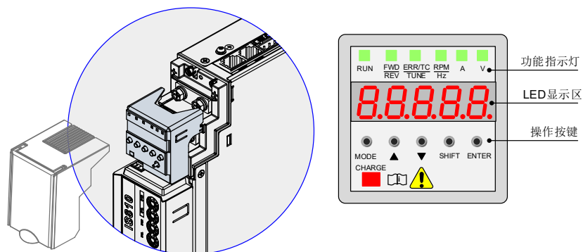
图 4-1 面板外观示意图
