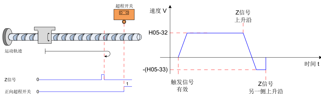
图 5-43 模式 2 原点回零电机运行曲线①与转速说明
