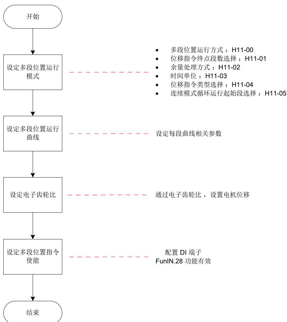
图 5-24 多段位置指令来源设置流程
