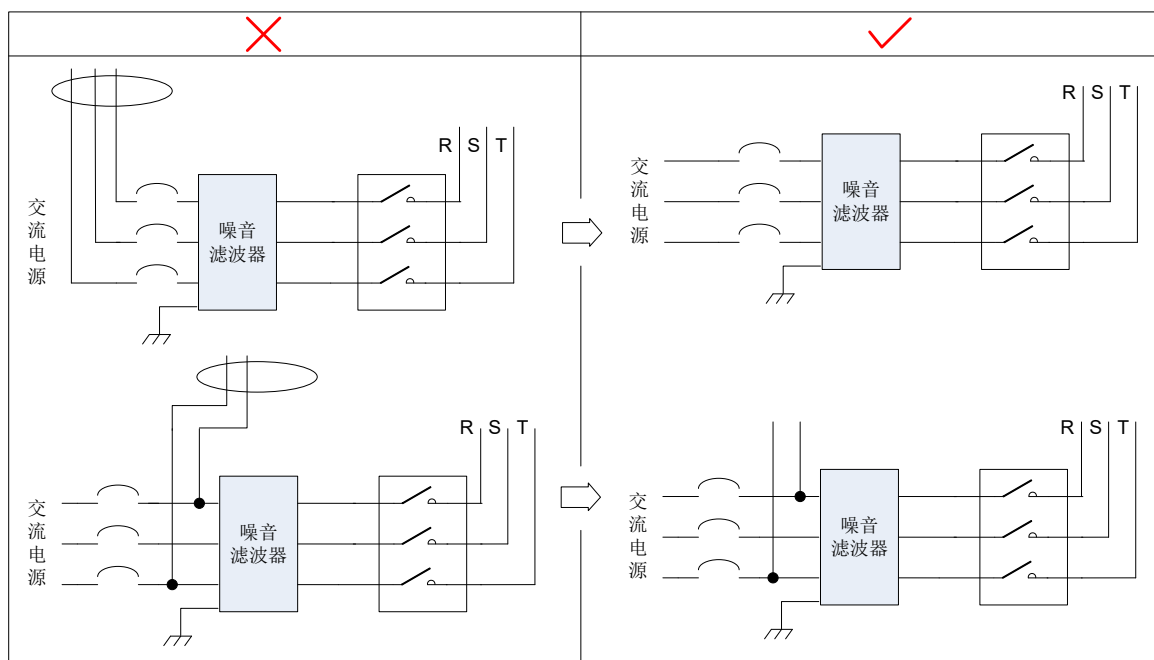
图 3-34 噪音滤波器输入与输出配线分离走线示意图
