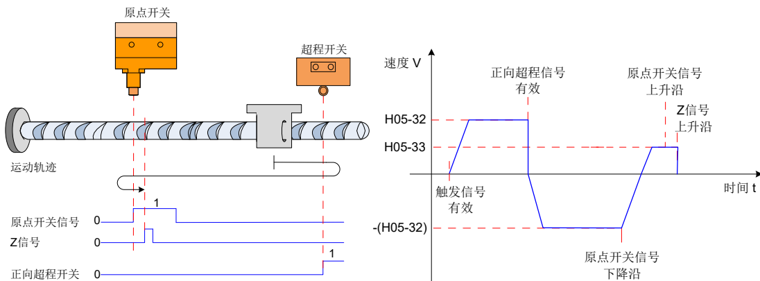
图 5-48 模式 4 原点回零电机运行曲线③与转速说明
