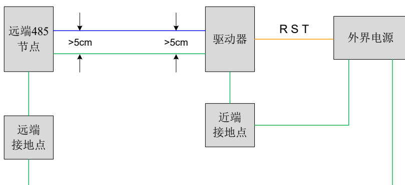
图 7-7 地线 PE 配线示意图
