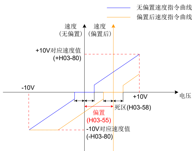
图 5-65 偏置 AI 示意图
