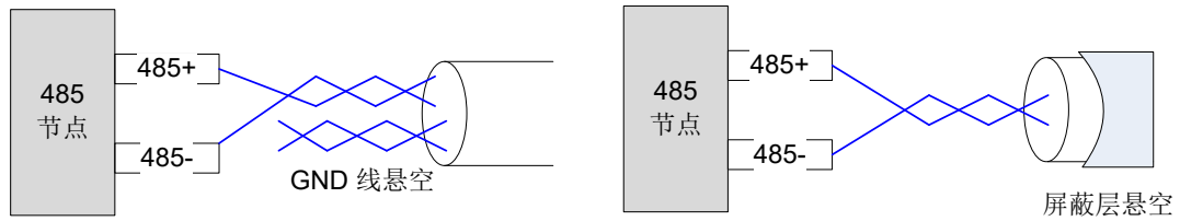
图 7-11 无 GND 时的接线示意图
