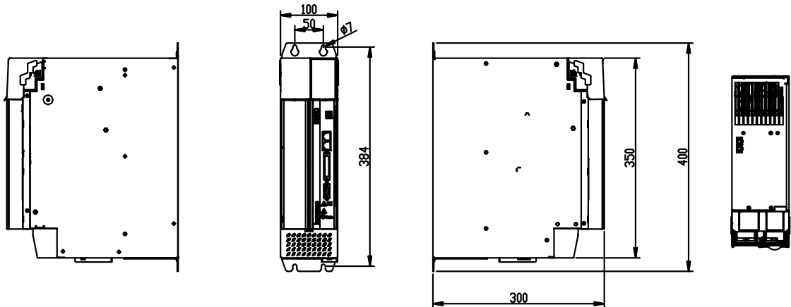
图 2-4 IS810P50M4T***** (SIZE 2) 外形尺寸图
