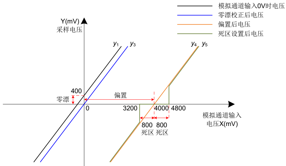
图 5-83 伺服驱动器 AI 处理对应采样电压举例
