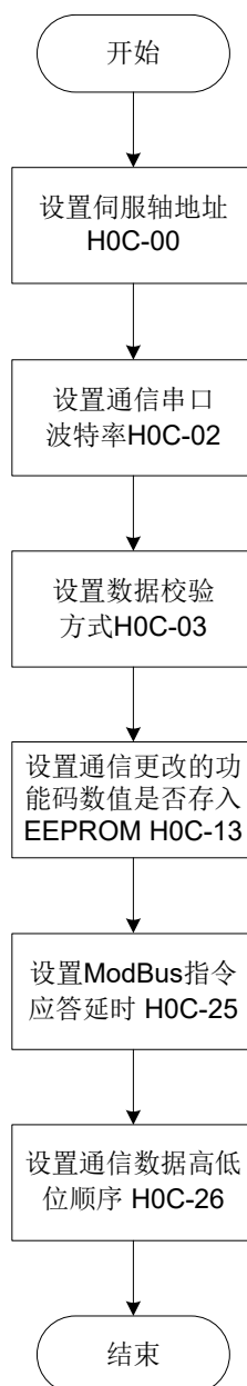
图 7-9 通信参数设定流程
