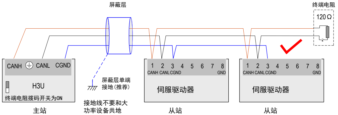
图 3-24 正确的 CAN 连接方法
