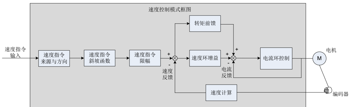
图 5-57 速度控制框图
