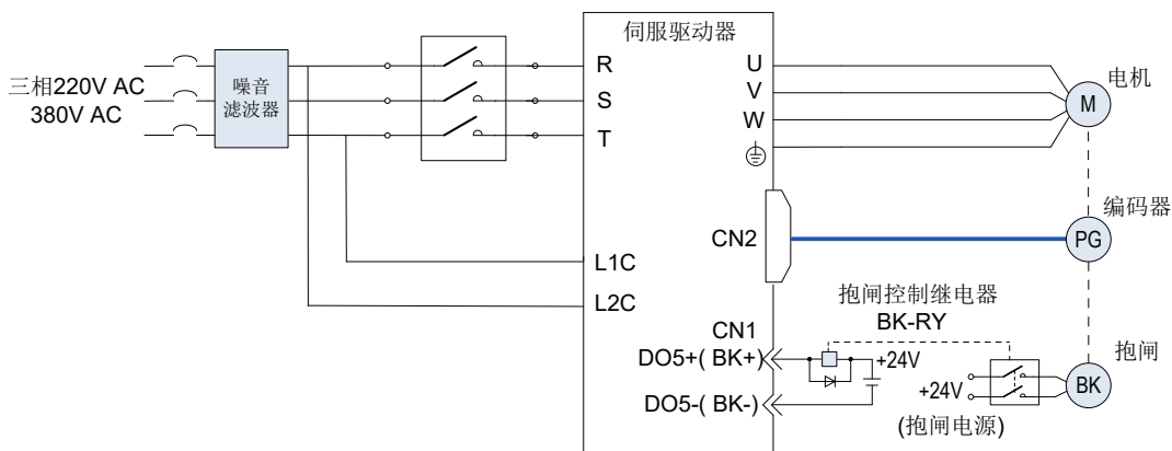
图 5-4 抱闸配线图
