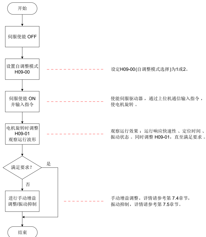
图 6-5 自动增益调整步骤
