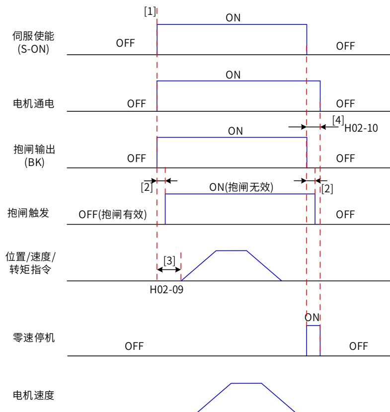
图 3-19 电机静止时抱闸时序图
