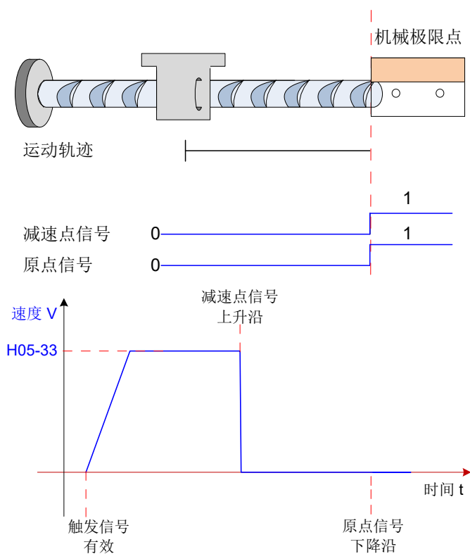
图 5-53 模式 10 原点回零电机运行曲线与转速说明
