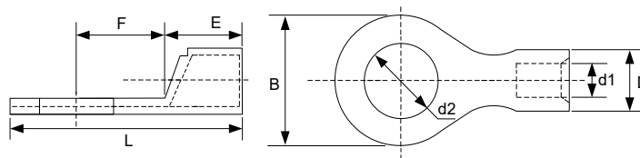
图 3-4 TNR 系列线耳尺寸图
