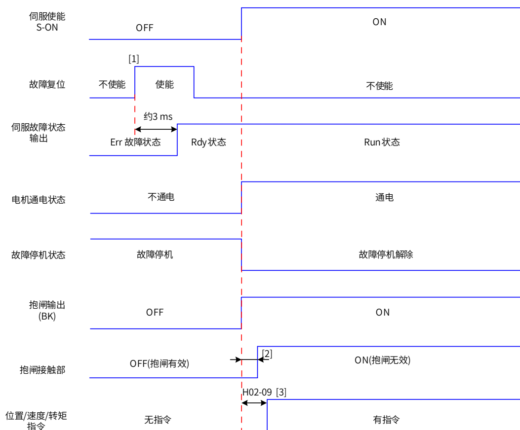
图 5-14 故障复位时序图
