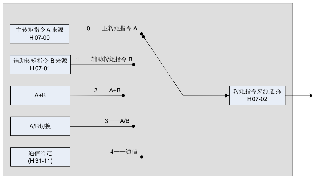
图 5-79 转矩指令来源图
