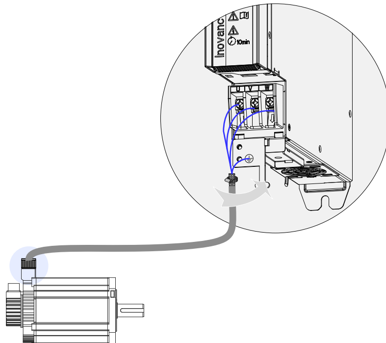
图 3-7 伺服驱动器输出与伺服电机连接举例
