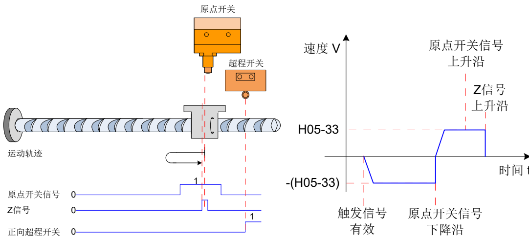
图 5-47 模式 4 原点回零电机运行曲线②与转速说明
