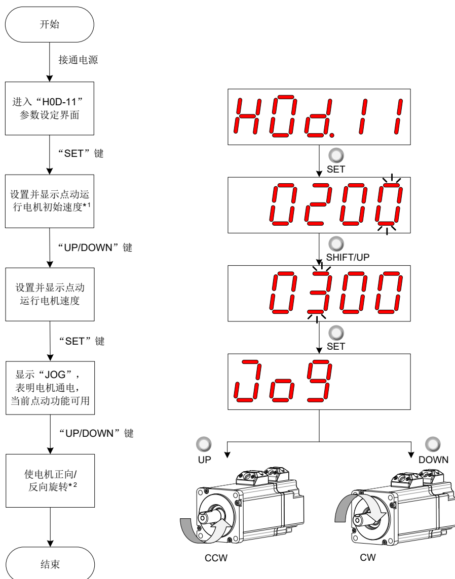
图 4-7 点动运行设定步骤示意图
