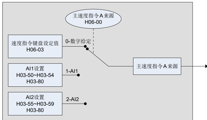
图 5-60 主速度指令 A 来源图
