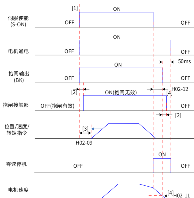
图 5-6 电机旋转时抱闸时序图
