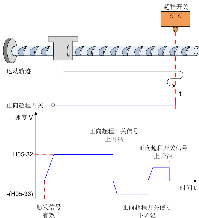
图 5-49 模式 6 原点回零电机运行曲线①与转速说明
