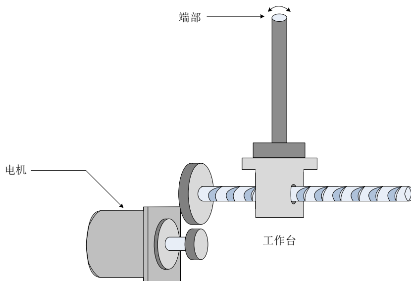
图 6-16 低频共振机械示意图
