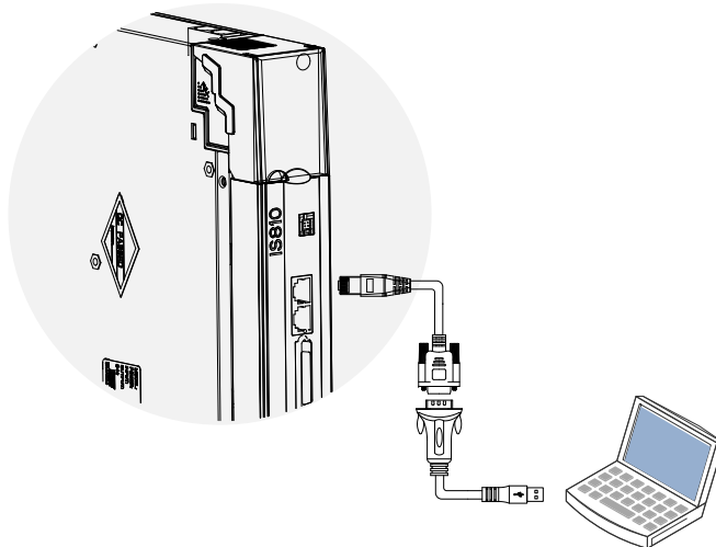
图 3-31 通讯串口转 USB 示意图
