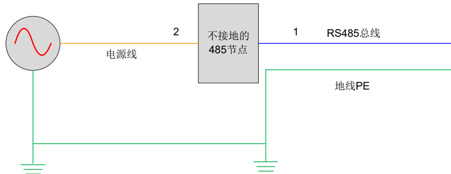
图 7-13 抑制外部干扰示意图
