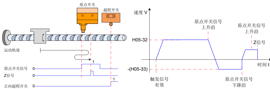
图 5-46 模式 4 原点回零电机运行曲线①与转速说明
