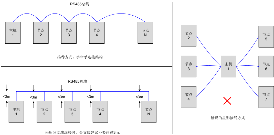
图 7-12 三种多节点连接方式示意图
