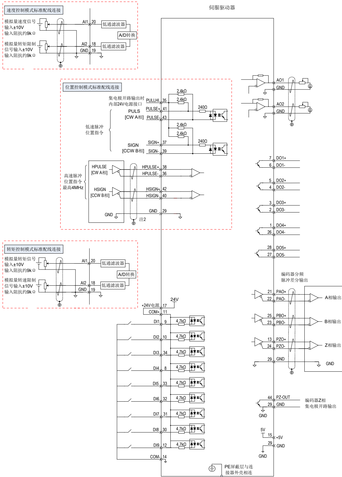
图 3-15 三种控制模式配线图举例
