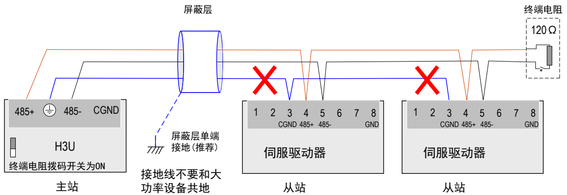
图 3-29 错误的 485 连接方法
