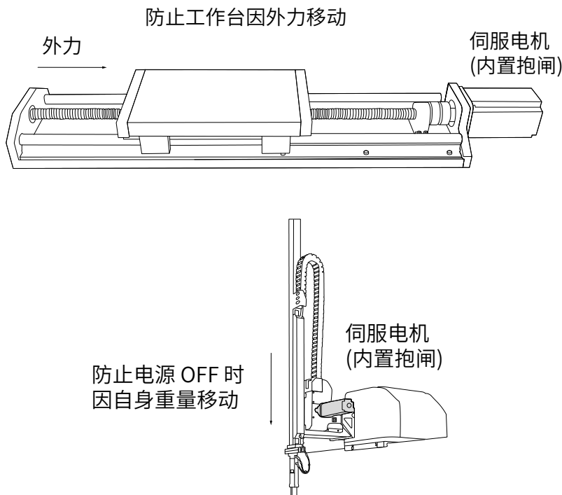
图 5-3 抱闸应用示意图
