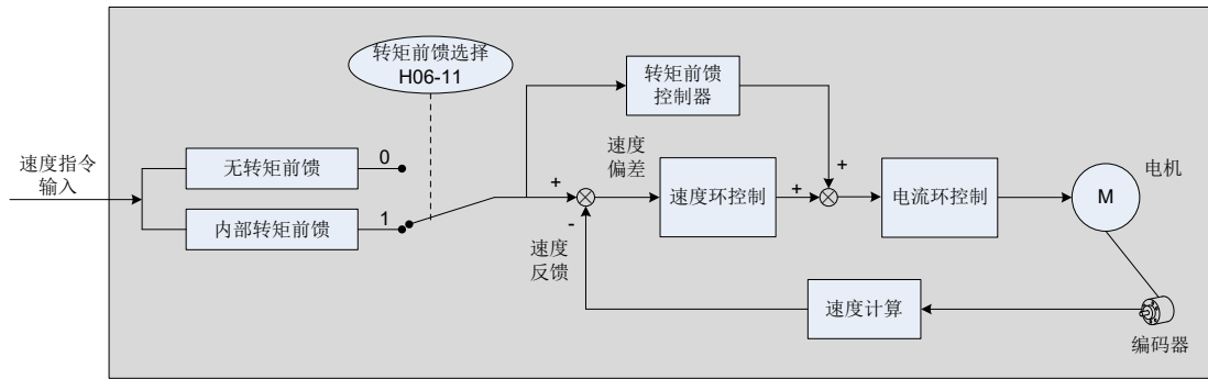
图 6-10 转矩前馈控制操作图
