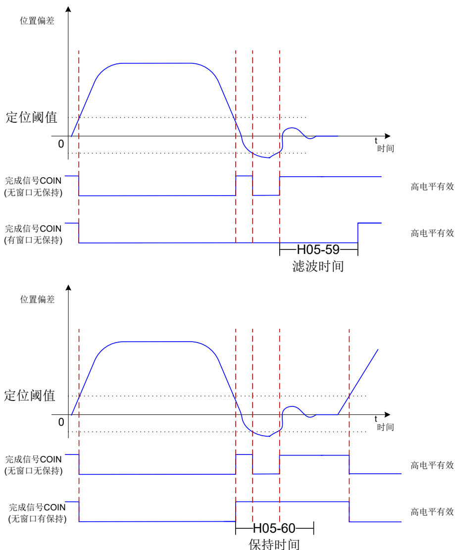
图 5-37 定位完成窗口时间和保持时间的原理图
