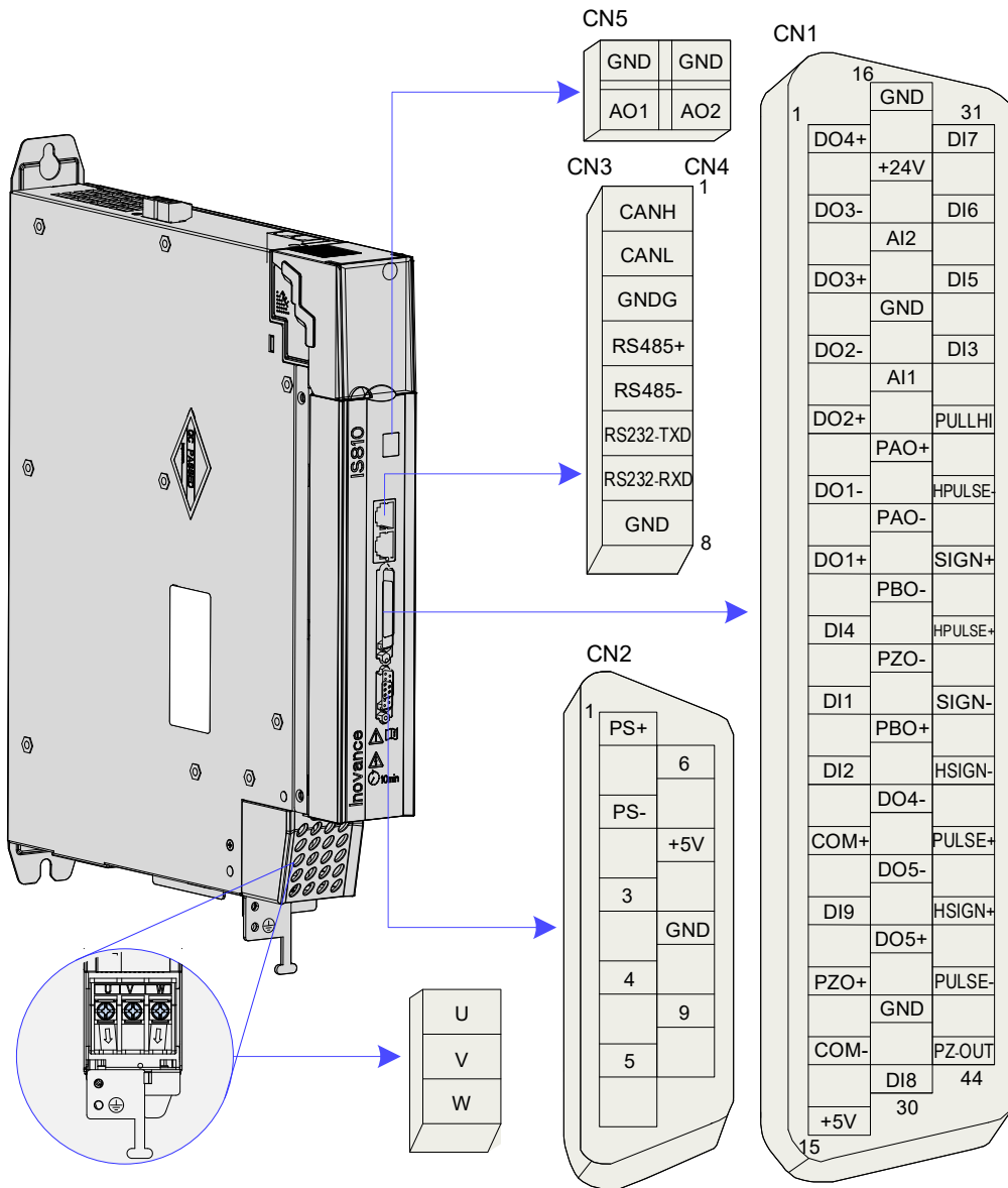
图 3-2 逆变单元端子引脚分布图
