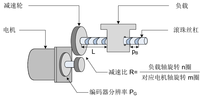
图 5-31 滚珠丝杠图示
