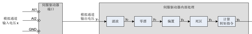
图 5-82 伺服驱动器 AI 处理流程
