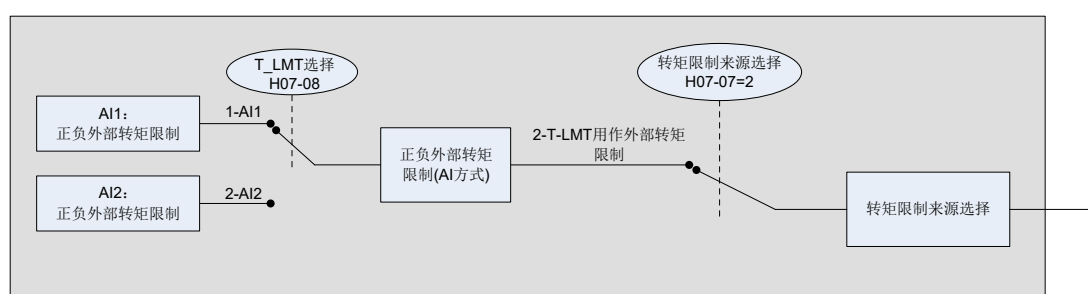
图 5-91 H7-07=2 转矩限制来源
