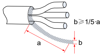
图 3-12 机电缆屏蔽层引出示意图
