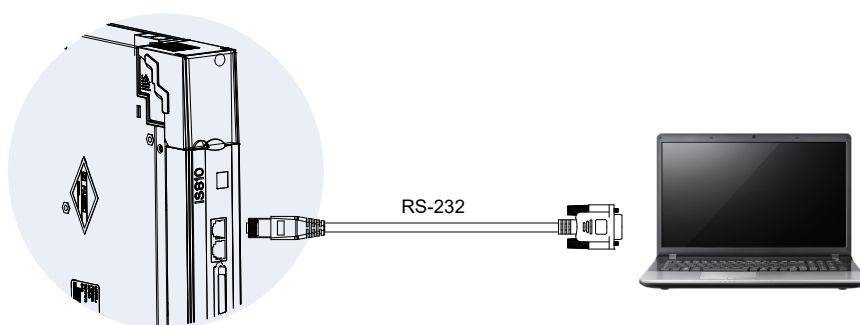
图 7-1 RS-232 连接示意图
