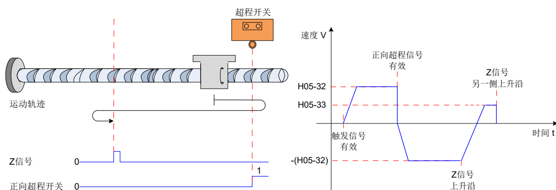
图 5-45 模式 2 原点回零电机运行曲线③与转速说明
