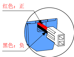
图 3-10 绝对值编码器电池外引线说明
