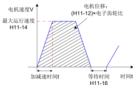
图 5-26 第 1 段电机运行曲线
