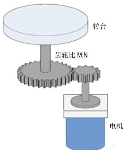
图 5-101 旋转负载示意图
