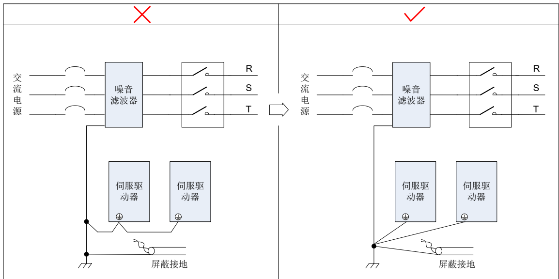
图 3-36 单点接地示意图
