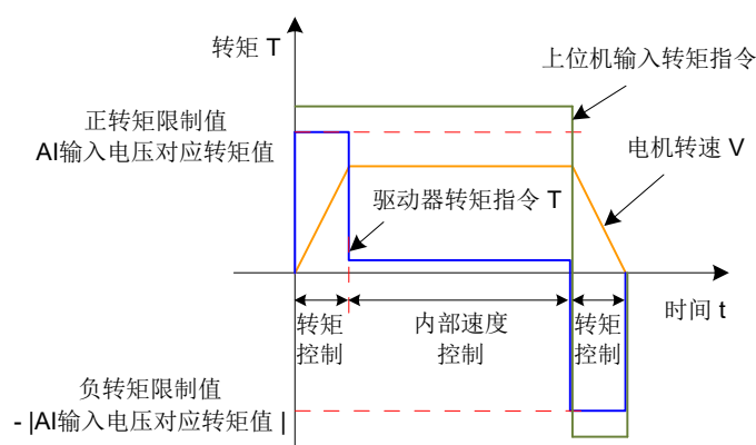
图 5-92 H07-07=2 转矩限制曲线图
