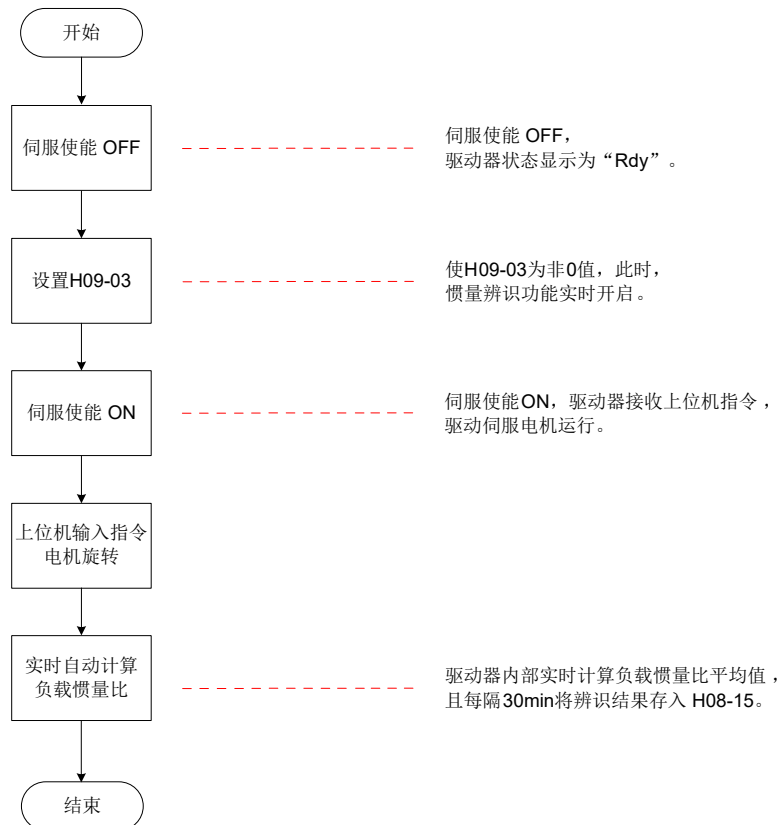
图 6-4 在线惯量辨识操作流程
