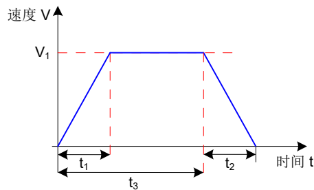
图 5-69 多段速度曲线举例
