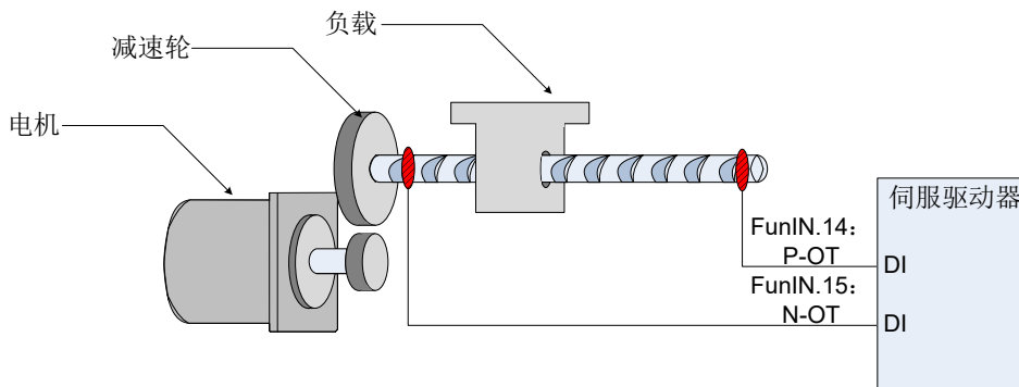
图 5-104 限位开关的安装示意图
