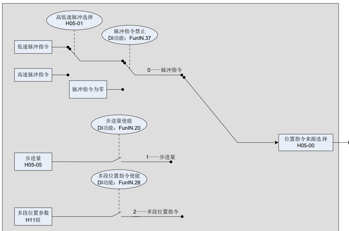
图 5-19 位置指令来源设置
