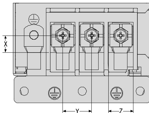
图 3-3 端子台示意图
