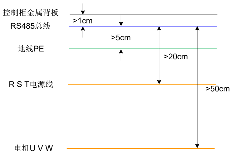
图 7-8 线缆布置示意图
