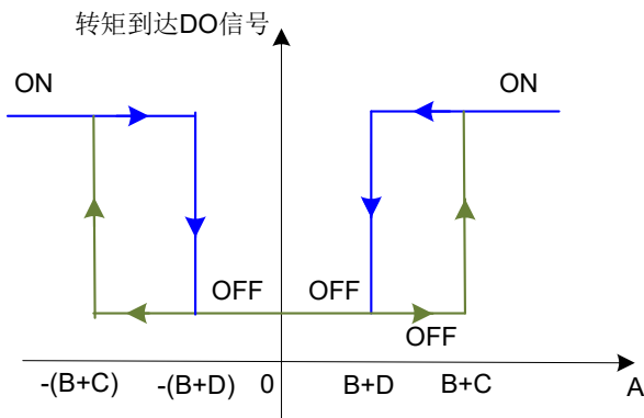
图 5-99 转矩到达输出有效说明
