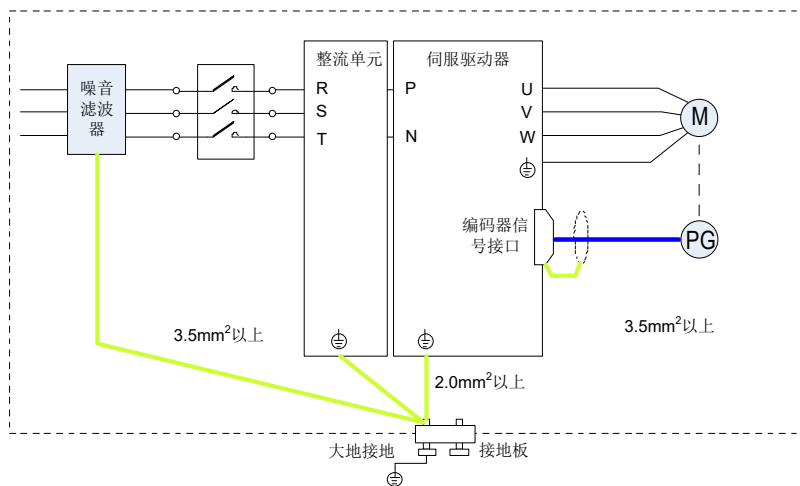
图 3-33 抗干扰配线实例
