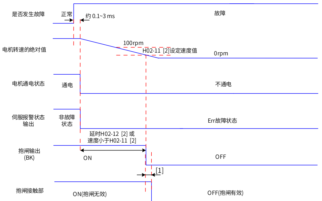
图 5-8 故障 1 时自由停机保持自由运行状态时序图
