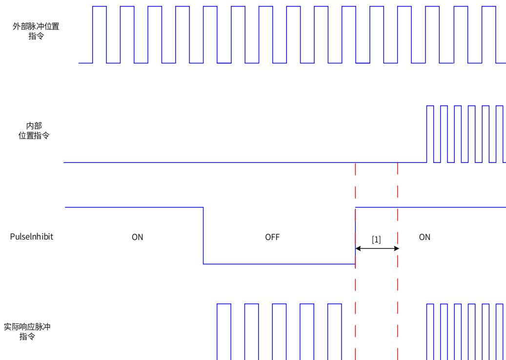
图 5-28 脉冲指令禁止功能波形举例
