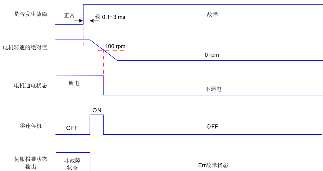
图 5-10 故障 2(非抱闸)时零速停机保持自由运行状态时序图
