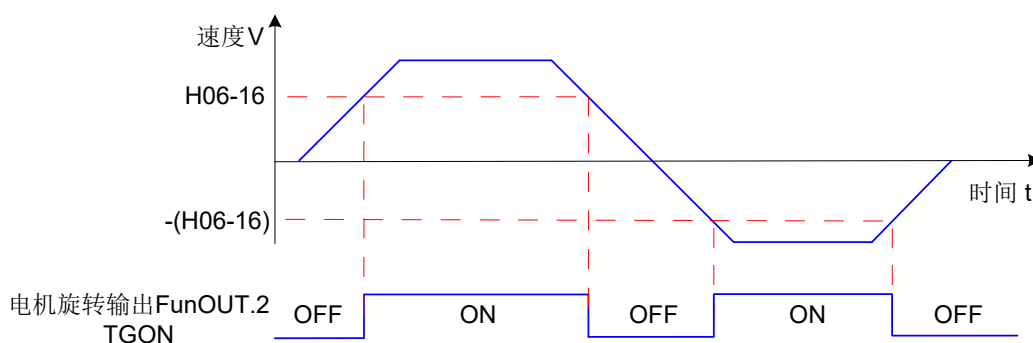
图 5-73 电机旋转信号波形图
