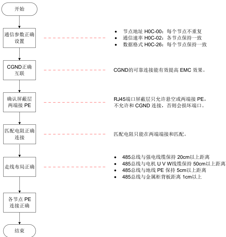
图 7-15 485 通信现场问题定位流程图
