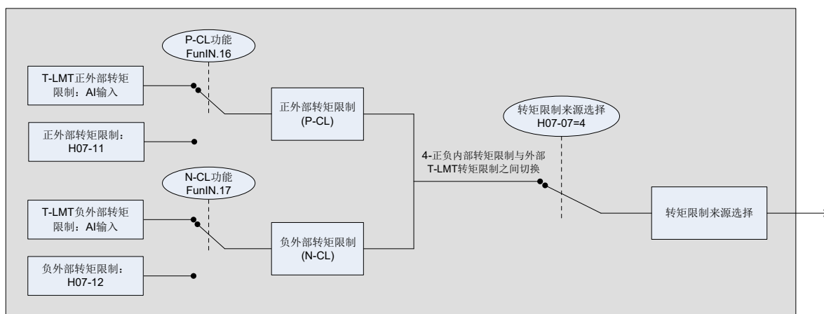
图 5-94 H7-07=4 转矩限制来源
