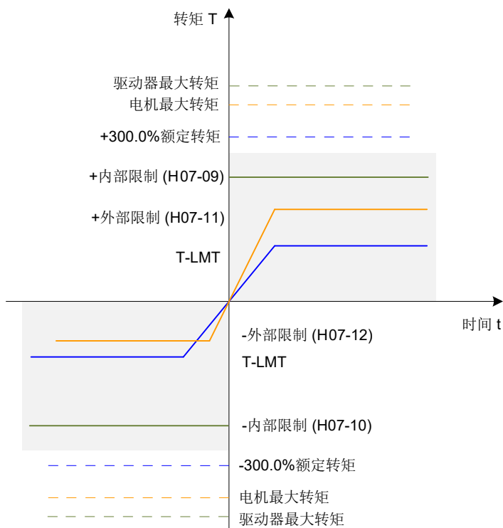
图 5-87 转矩限制举例
