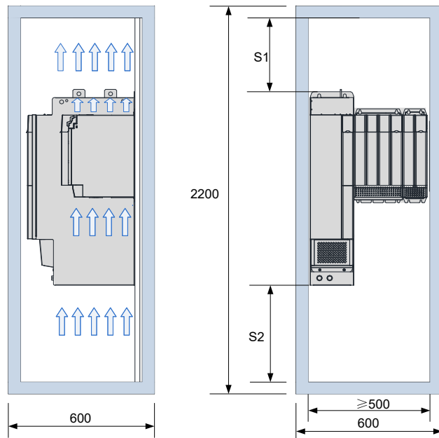
图 2-7 立式整流单元双层安装空间
