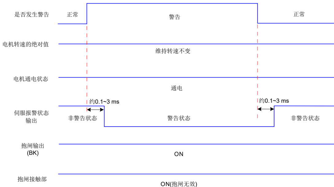
图 5-13 非停机警告时序图
