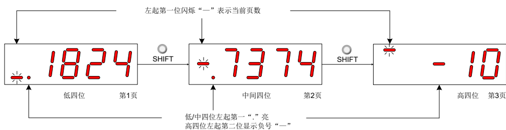
图 4-3 -1073741824 显示操作示意图
