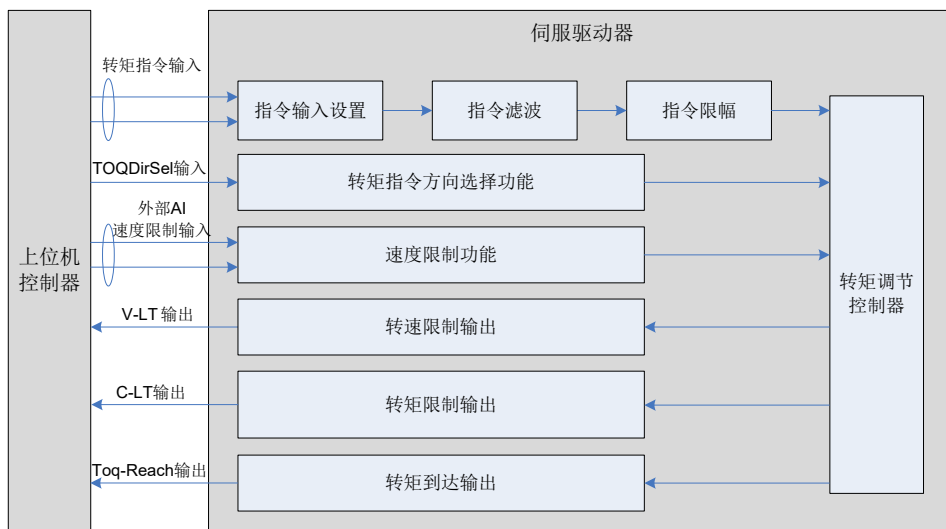
图 5-78 伺服驱动器与上位机信号交互图
