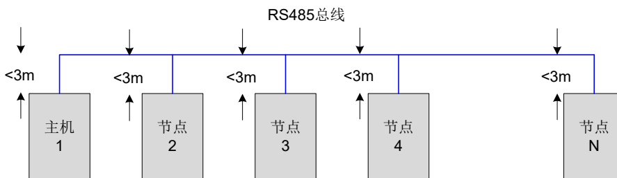
图 7-4 分支线连接结构示意图
