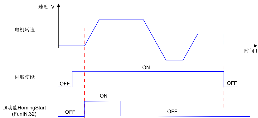
图 5-56 时序图举例
