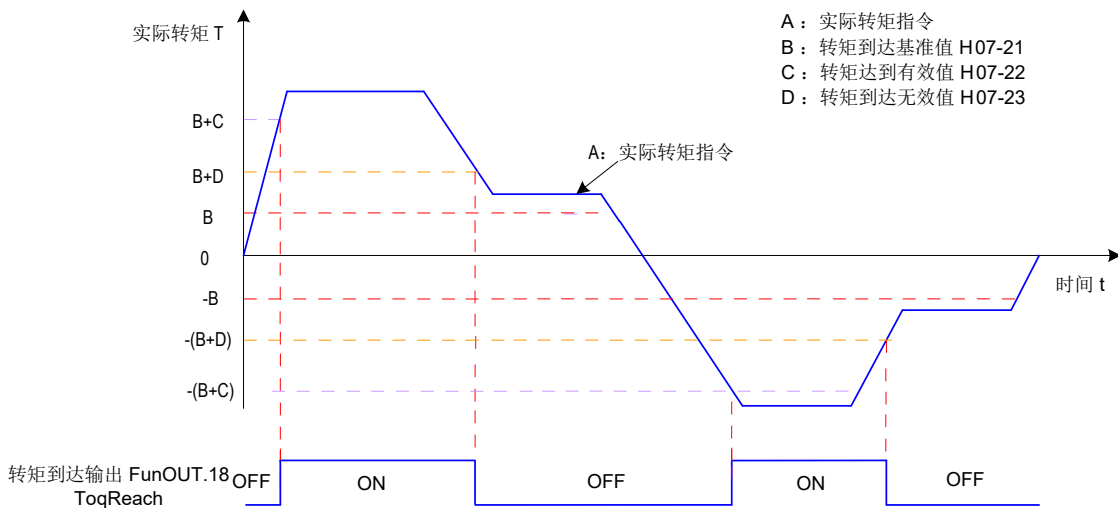
图 5-98 转矩到达输出波形举例
