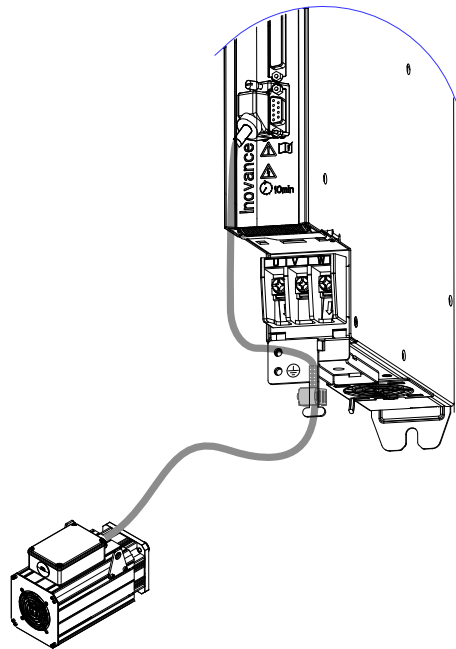
图 3-13 编码器信号接线示例图
