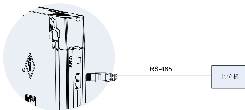
图 7-2 RS-485 连接示意图
