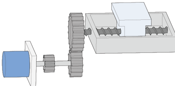
图 5-100 滚珠丝杠传动机构示意图
