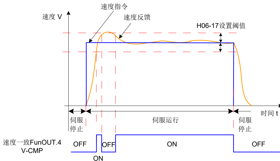
图 5-74 速度一致信号波形图
