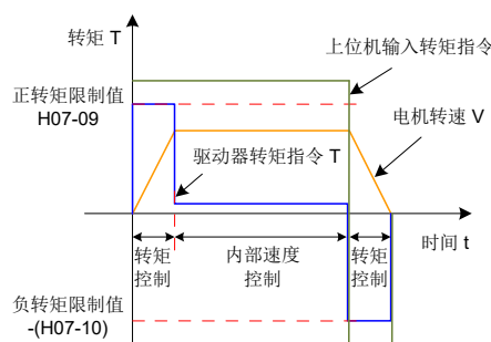
图 5-89 H07-07=0 转矩限制曲线图
