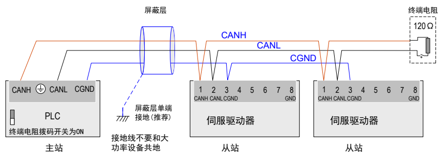
图 7-17 CANopen 连接示意图
