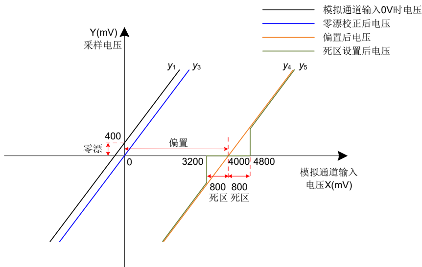
图 5-63 伺服驱动器 AI 处理对应采样电压举例
