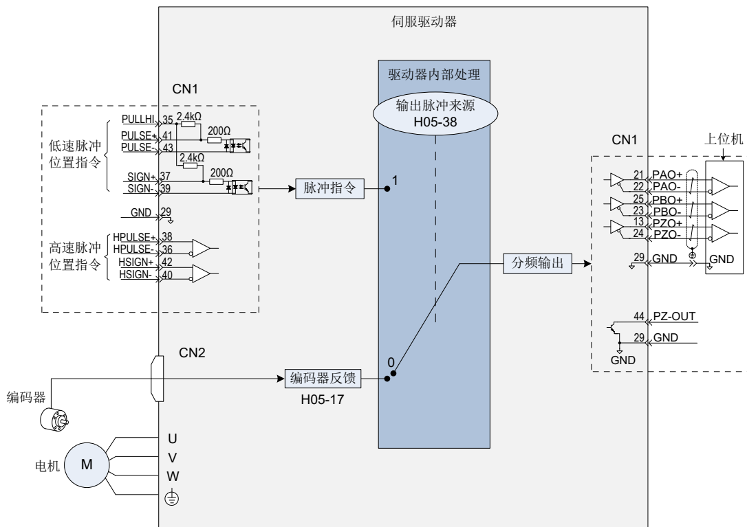
图 5-34 分频输出原理示意图
