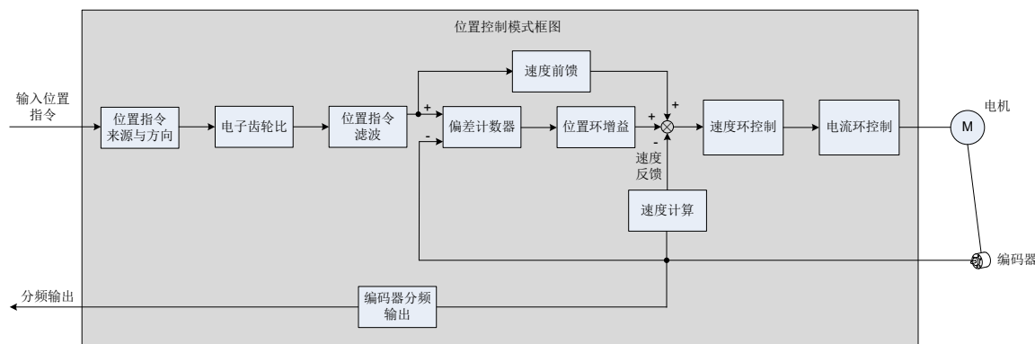
图 5-16 位置控制框图
