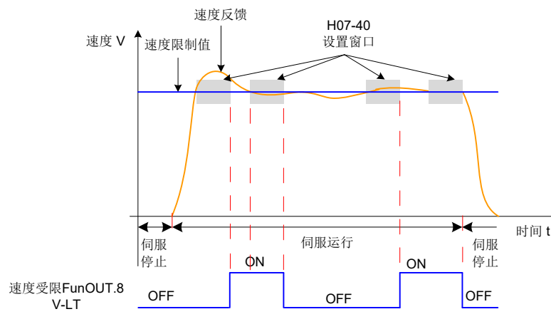
图 5-97 速度限制 DO 输出波形举例
