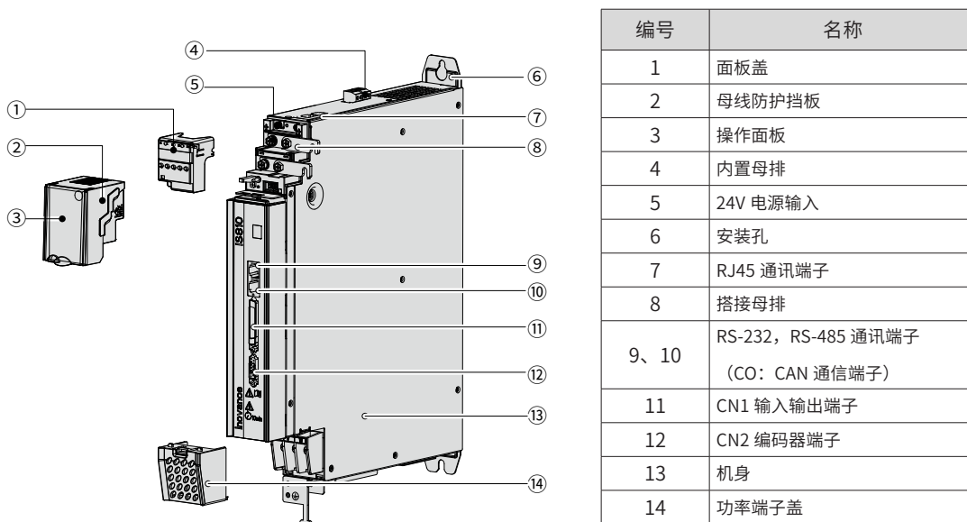
图 1-3 逆变单元组成说明
