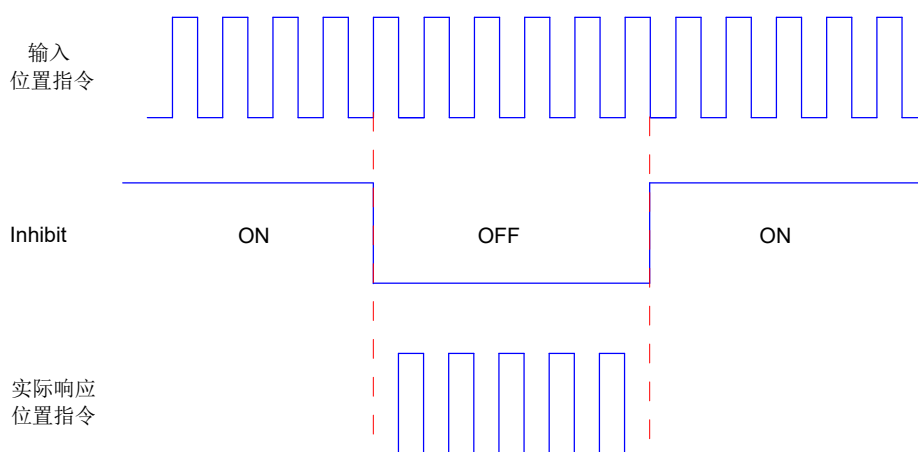
图 5-27 位置指令禁止功能波形举例
