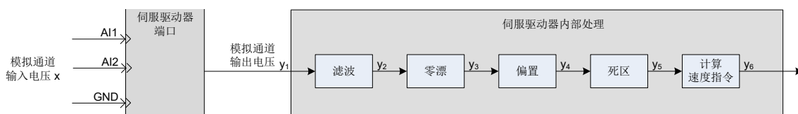
图 5-62 伺服驱动器 AI 处理流程
