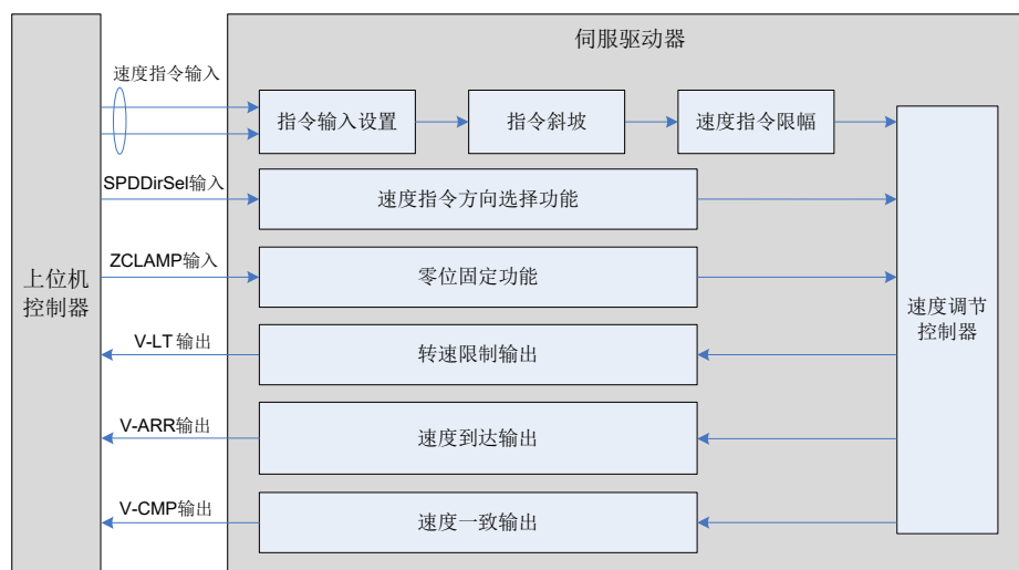
图 5-58 伺服驱动器与上位机信号交互图
