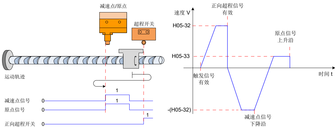
图 5-42 模式 0 原点回零电机运行曲线③与转速说明
