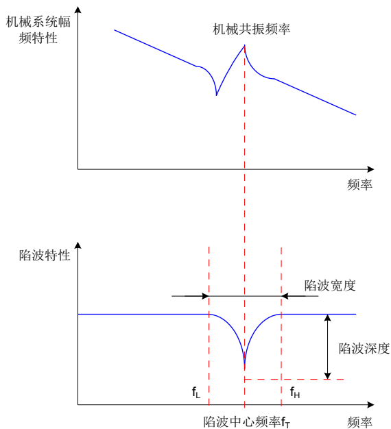
图 6-13 陷波器的抑制原理
