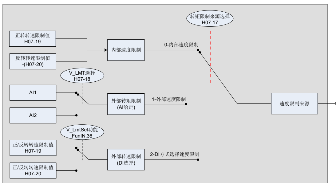
图 5-95 速度限制来源
