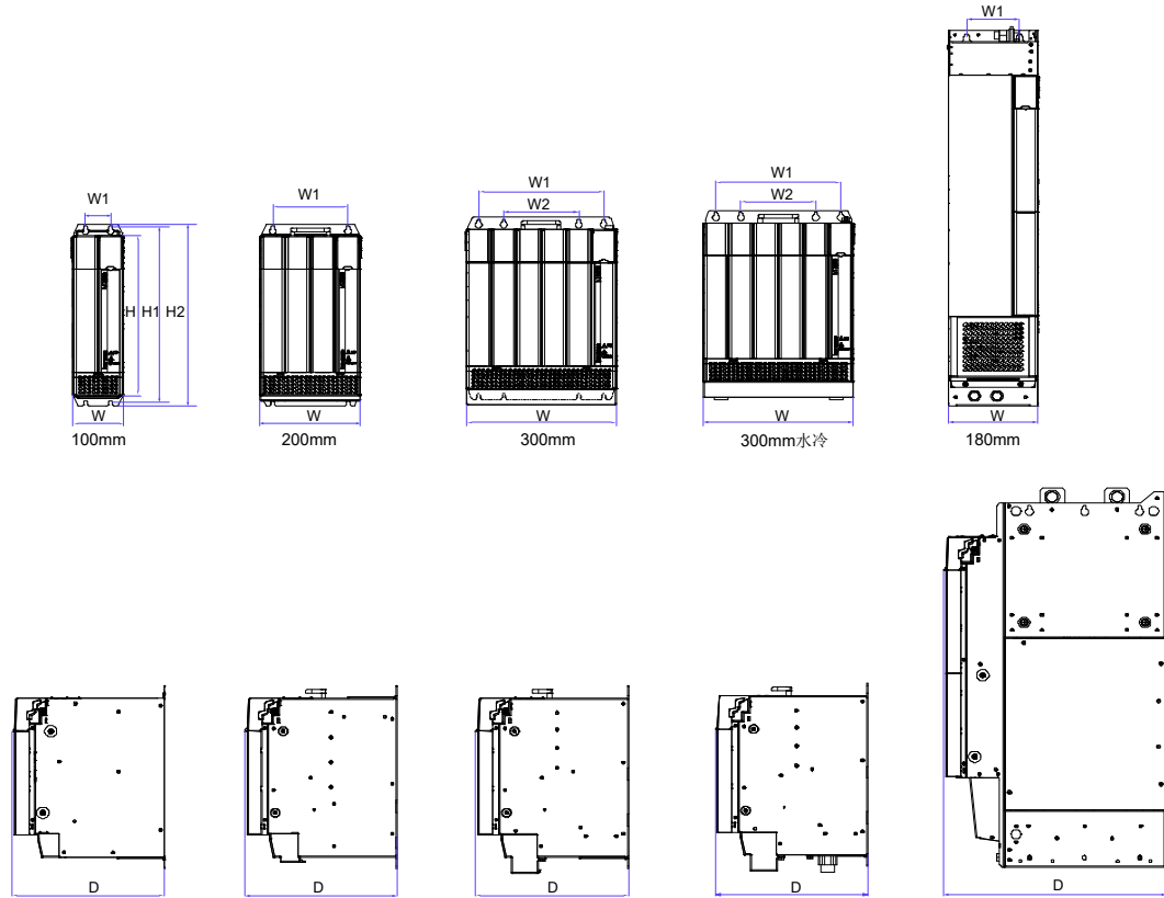
图 2-2 MD810-20M4T**G*** 外型尺寸示意图
