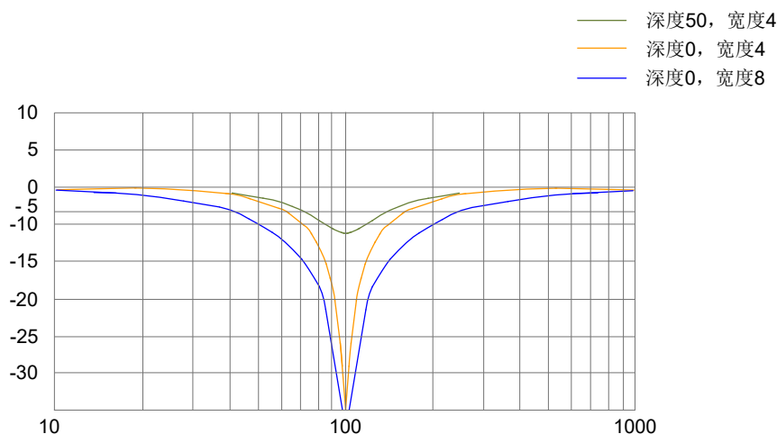
图 6-15 陷波器频率特性
