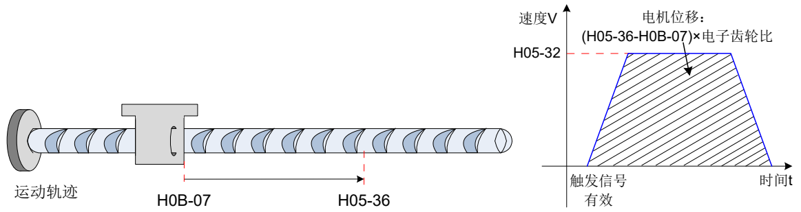
图 5-55 电气回零电机运行曲线与转速说明
