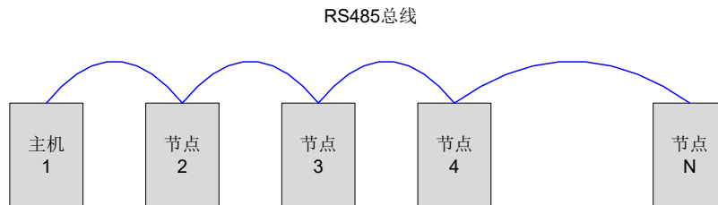
图 7-3 推荐手牵手连接结构示意图
