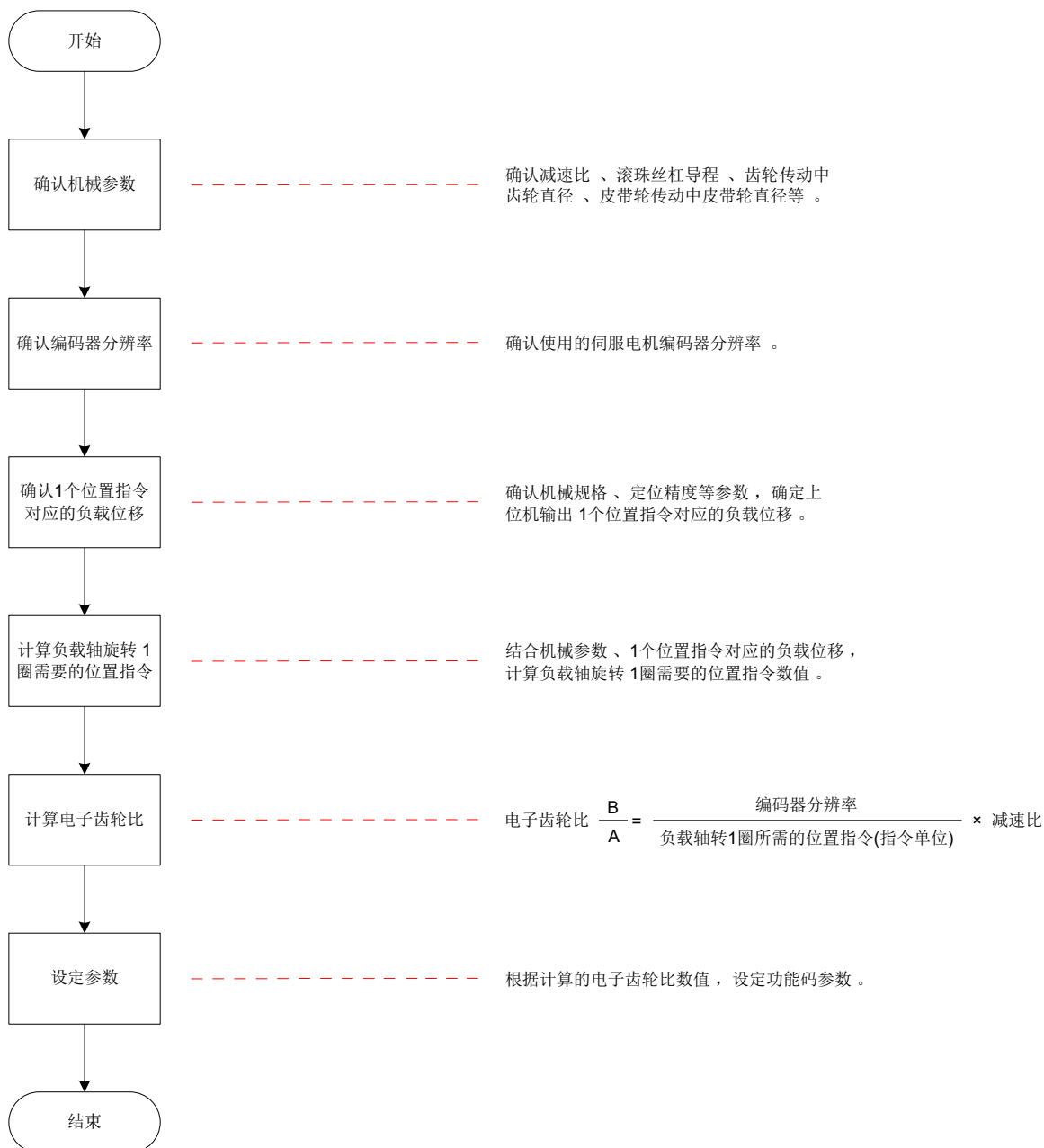
图 5-29 电子齿轮比设定步骤
