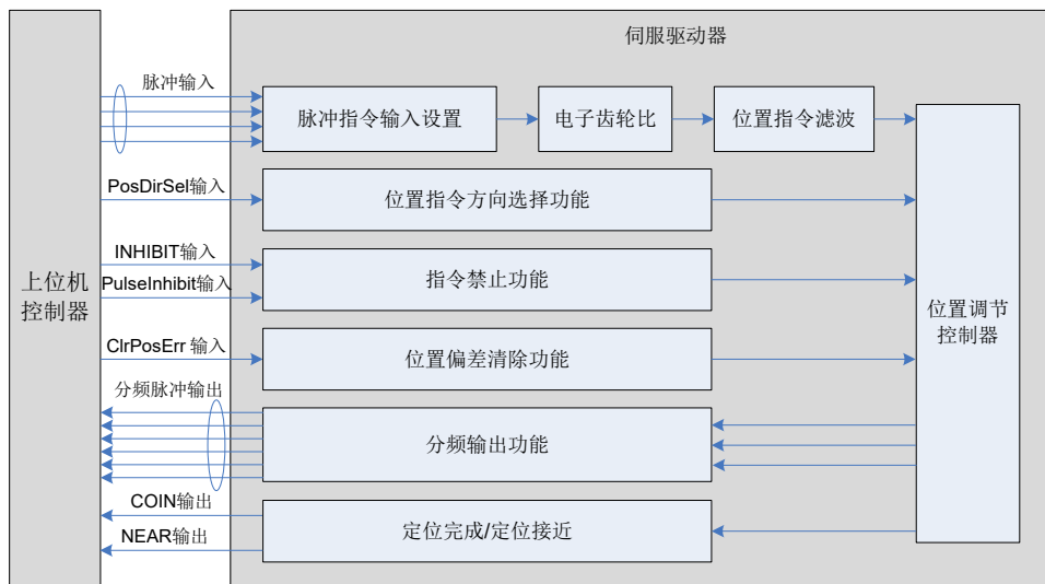
图 5-17 伺服驱动器与上位机信号交互图
