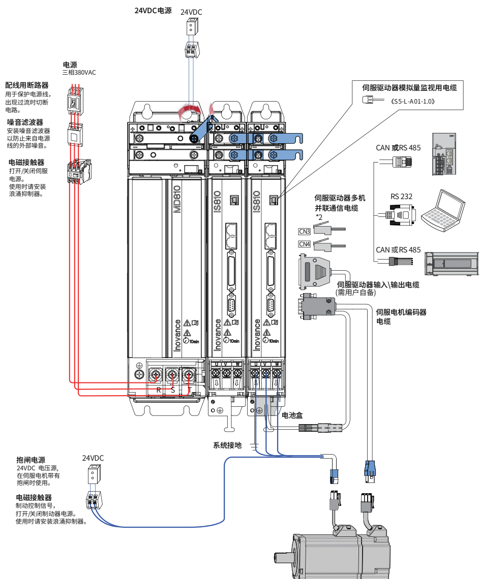
图 3-1 三相 380V 系统配线图举例
