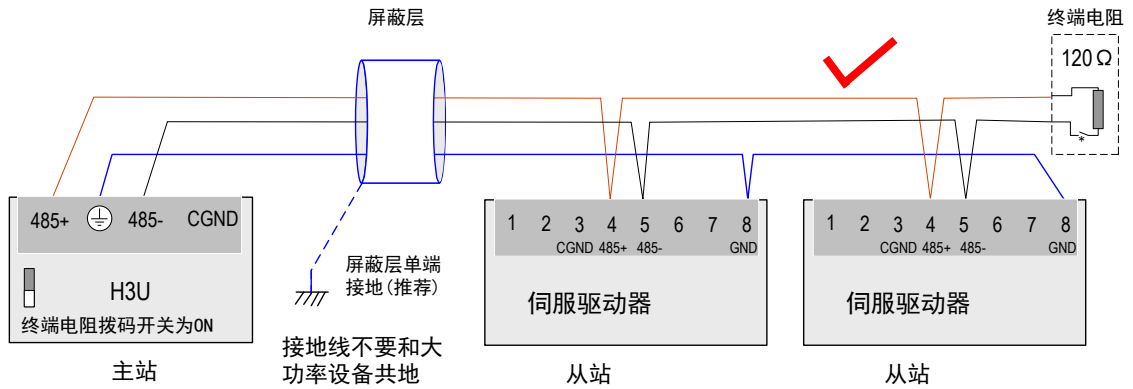
图 3-28 正确的 485 连接方法
