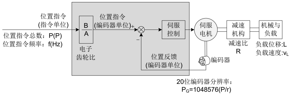
图 5-30 位置指令 (指令单位)、负载位移与电子齿轮比之间的关系
