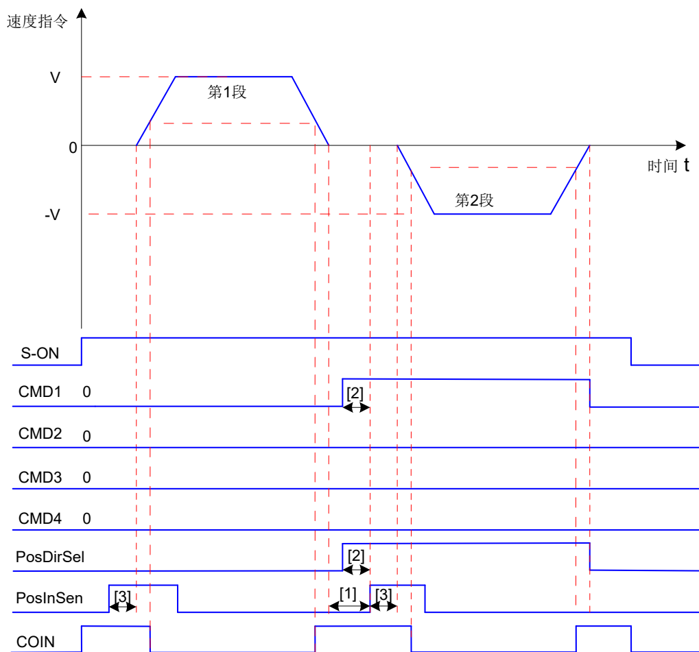
图 5-25 多段位置时序图
