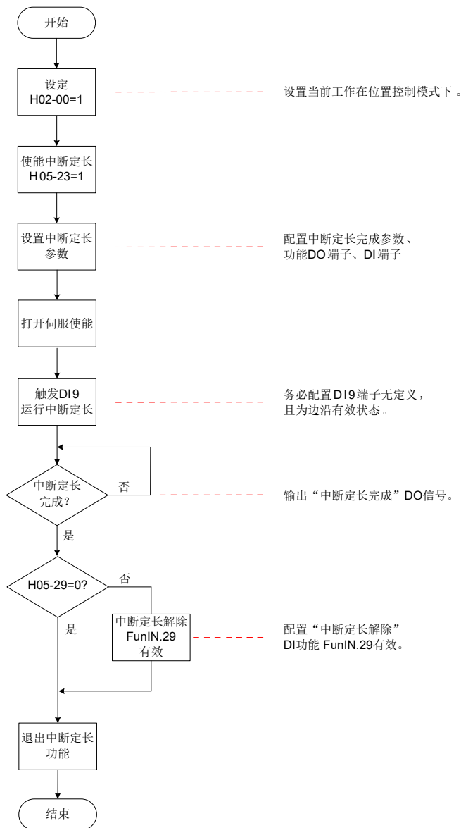
图 5-38 中断定长功能信号流程图
