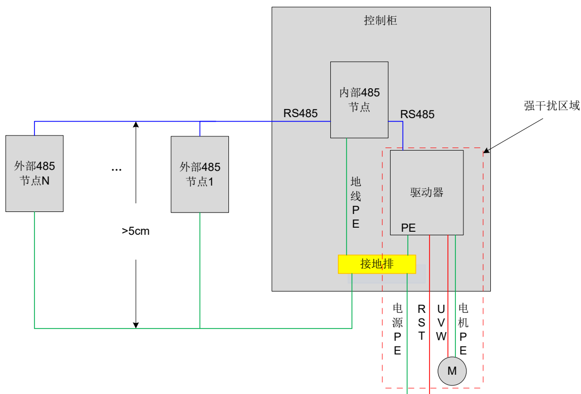
图 7-6 区域布置示意图
