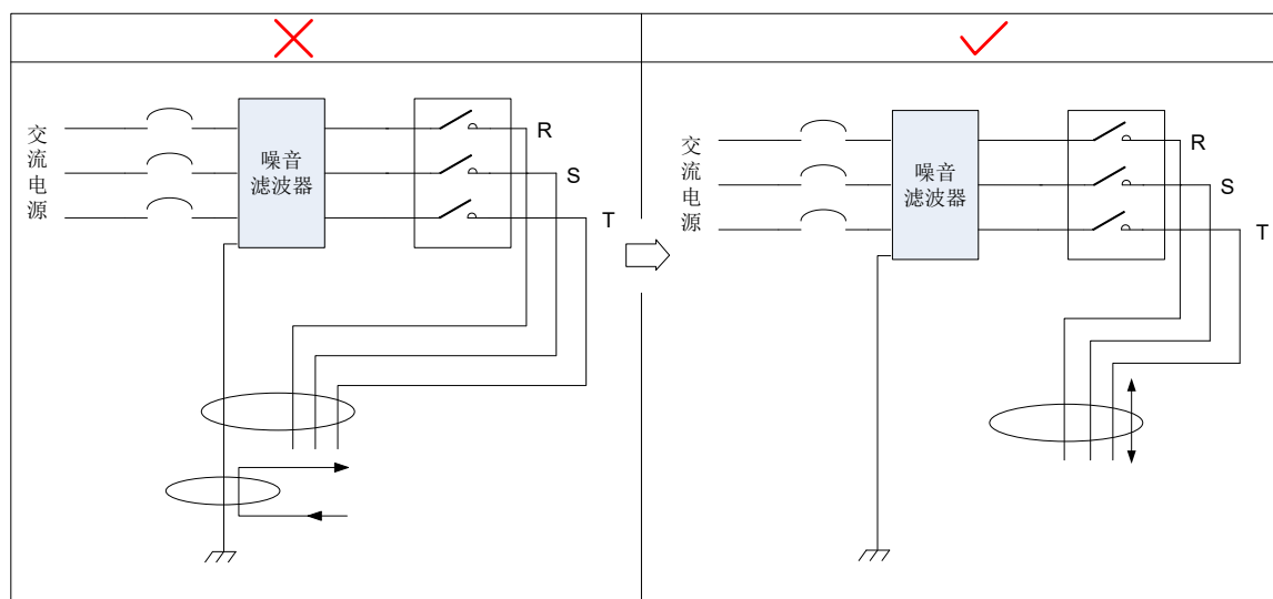
图 3-35 噪音滤波器地线与输出配线分离走线示意图
