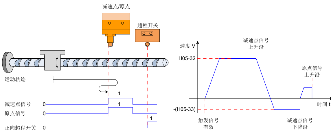
图 5-40 模式 0 原点回零电机运行曲线①与转速说明
