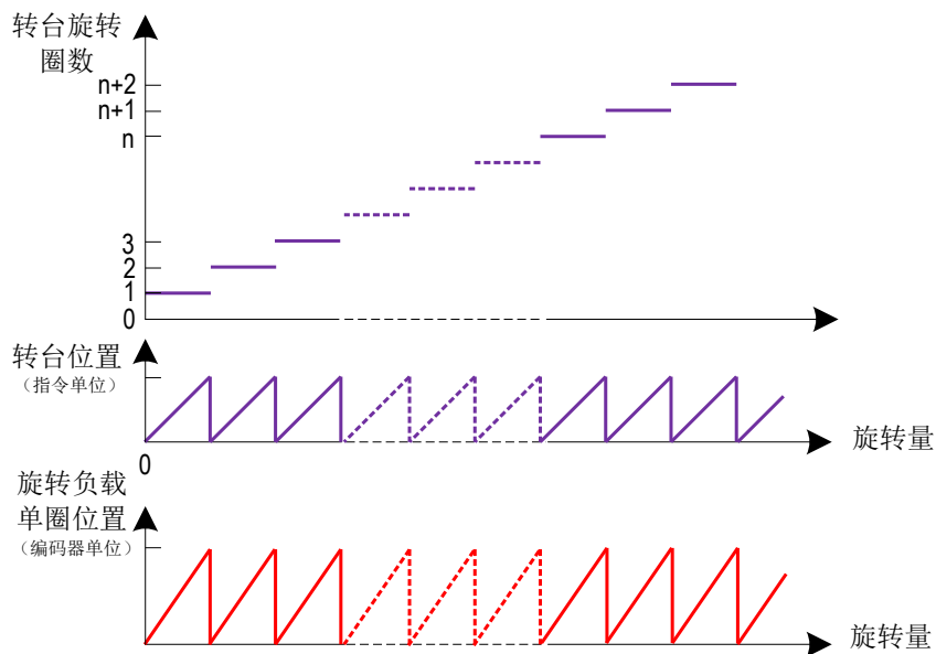
图 5-102 旋转负载单圈位置与转台位置对应关系示意图
