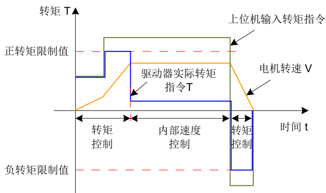
图 5-86 转矩给定与转矩限制
