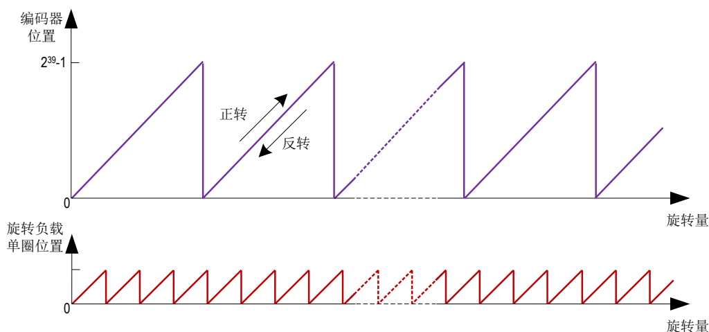
图 5-103 编码器反馈位置与旋转负载位置关系示意图
