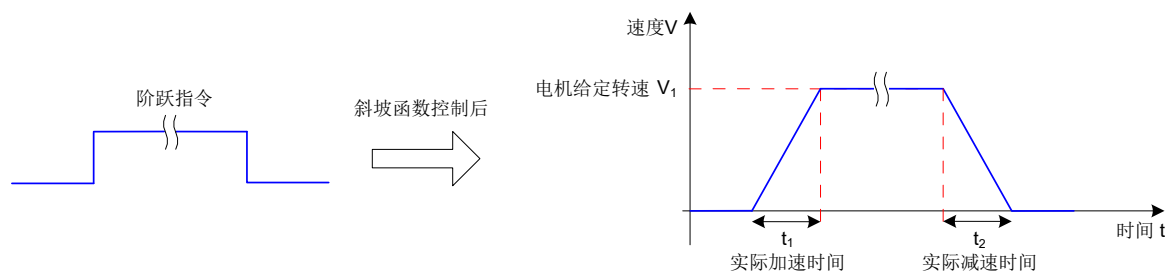
图 5-70 斜坡函数定义示意图
