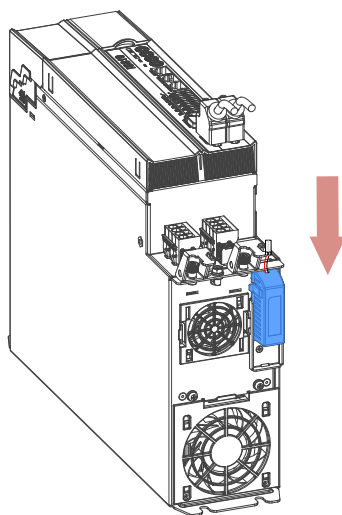
图 3-8 绝对值编码器电池盒安装示例图（SIZE2 机型，仰视图）
