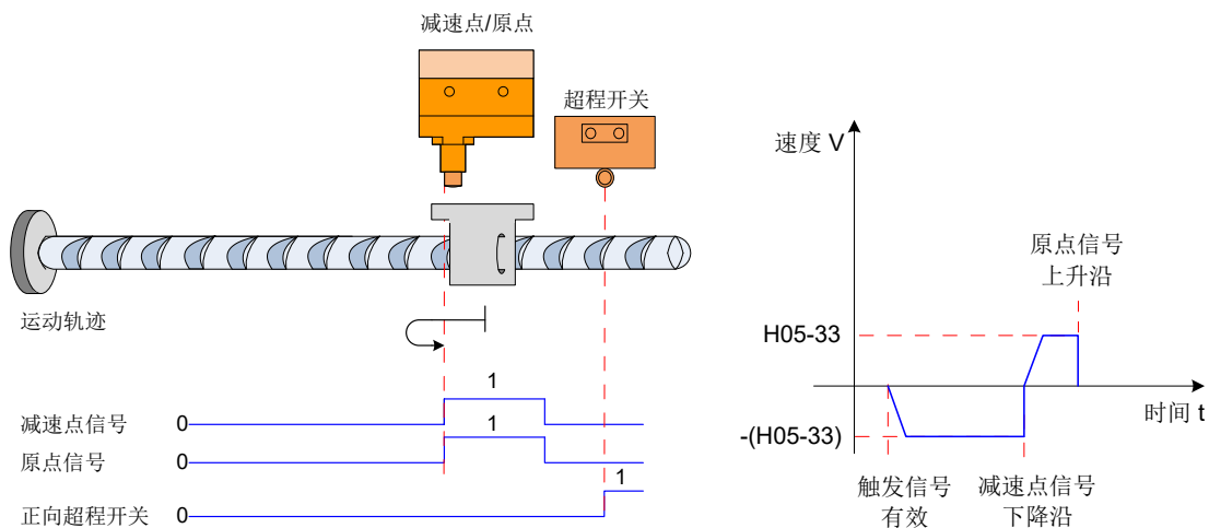
图 5-41 模式 0 原点回零电机运行曲线②与转速说明
