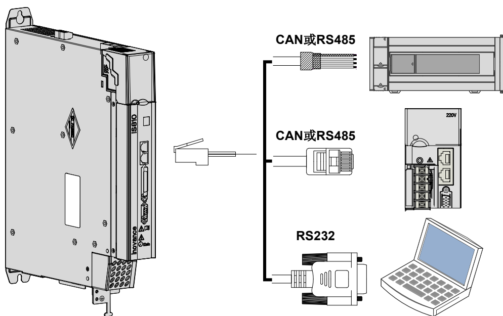
图 3-21 通信配线示意图
