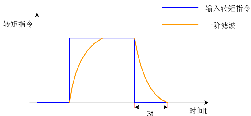
图 5-84 矩形转矩指令一阶滤波示意图
