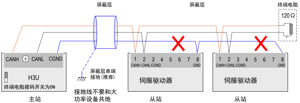
图 3-25 错误的 CAN 连接方法
