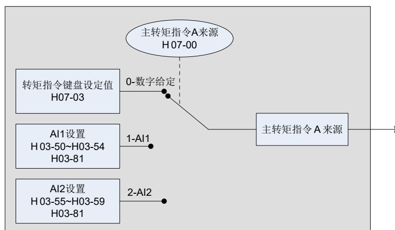
图 5-80 主转矩指令 A 来源说明
