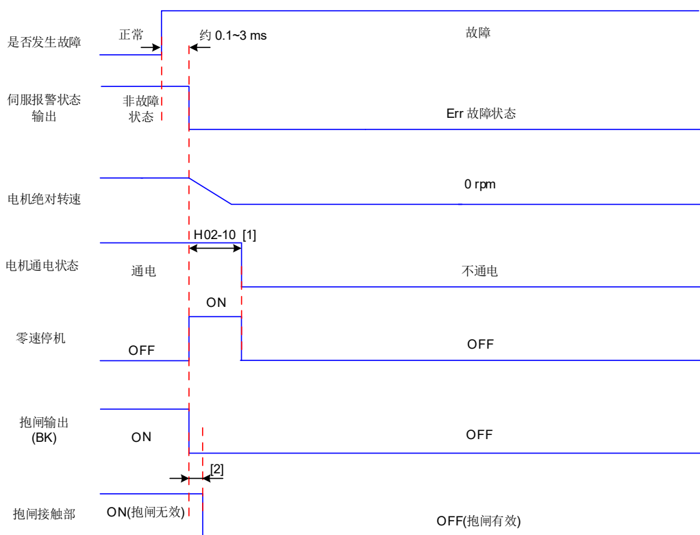
图 5-11 故障 2(带抱闸)时零速停机方式自由停机状态时序图
