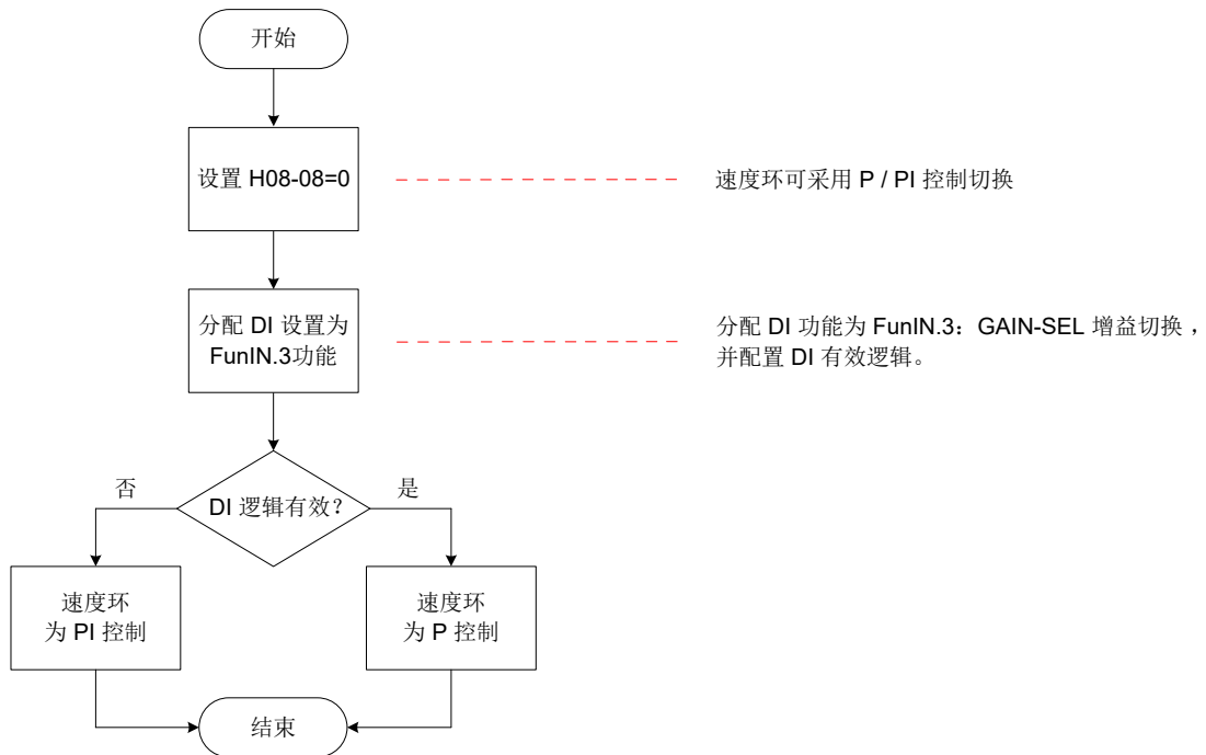
图 6-7 H08-08=0 增益切换流程图
