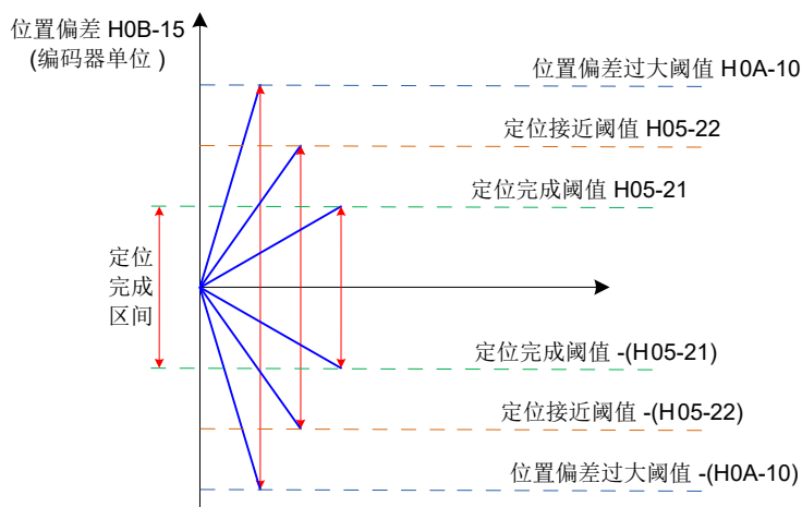
图 5-36 位置偏差相关信号
