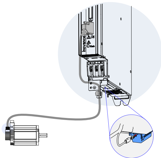
图 3-9 绝对值编码器信号接线及电池盒接线示例图
