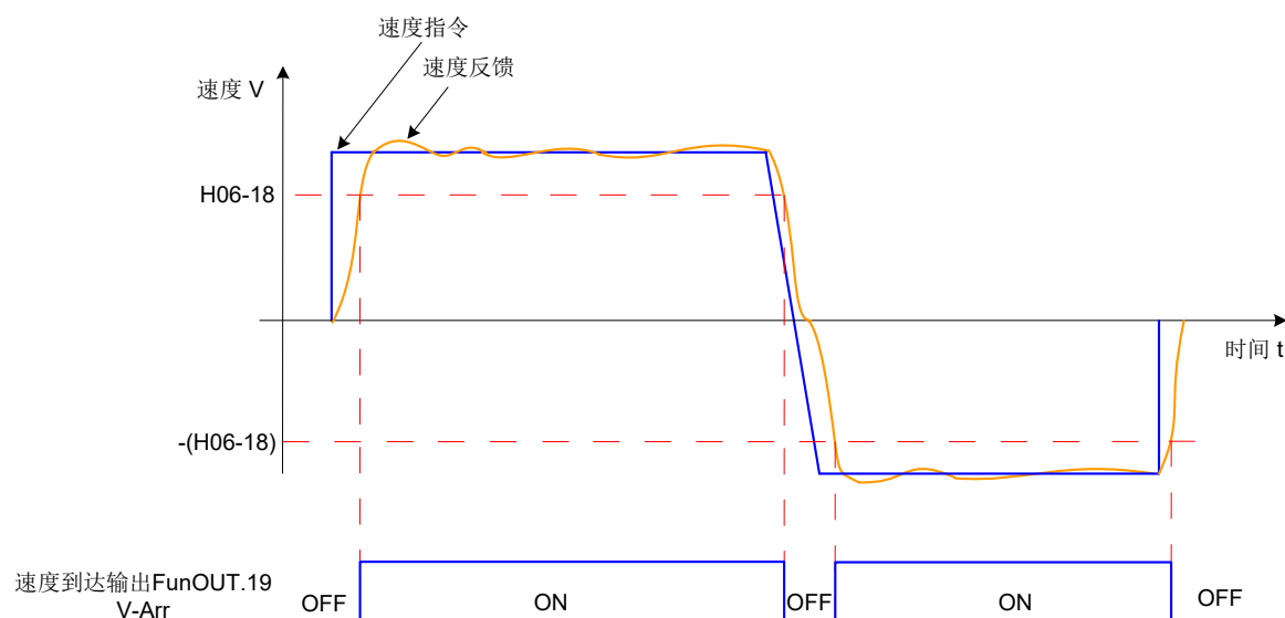
图 5-75 速度到达信号波形图
