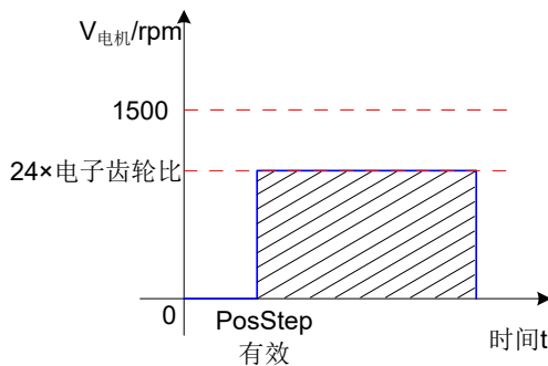
图 5-23 H05-00=1 时, 电机运行曲线
