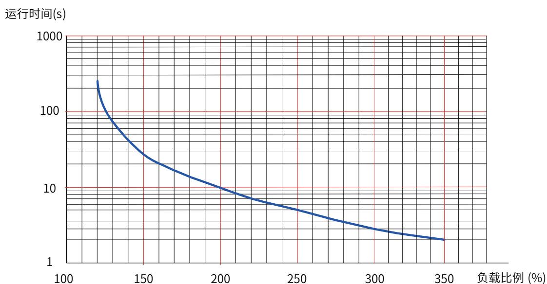
图 1-5 电机过载曲线
