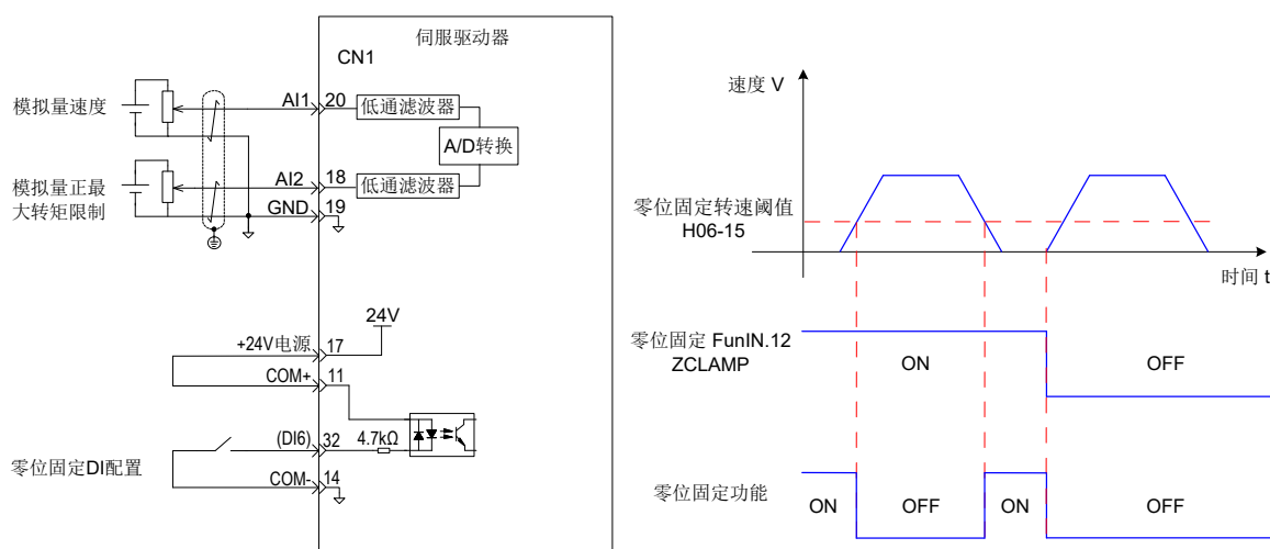
图 5-71 零位固定相关配线与波形图
