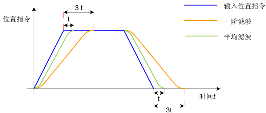
图 5-33 梯形位置指令一阶滤波与平均滤波示意图
