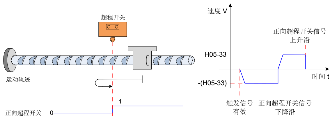
图 5-50 模式 6 原点回零电机运行曲线②与转速说明
