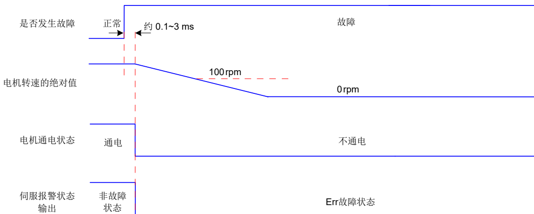
图 5-9 故障 2 时自由停机保持自由运行状态时序图
