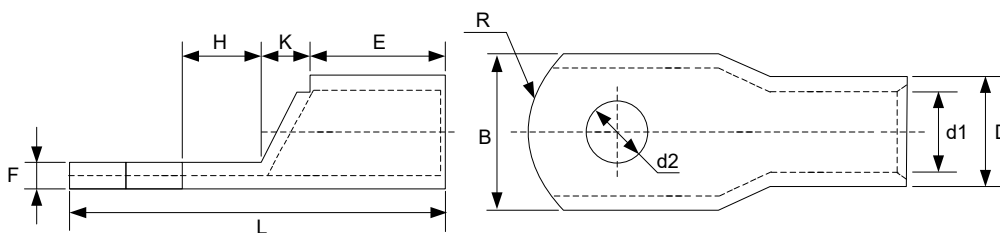
图 3-5 GTNR 系列线耳尺寸图
