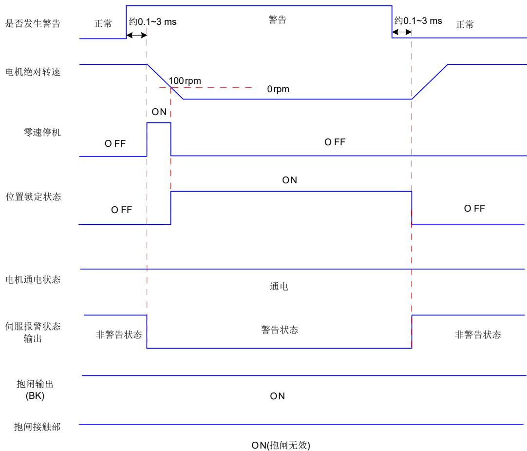
图 5-12 需停机类警告时序图
