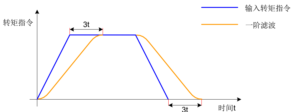
图 5-85 梯形转矩指令一阶滤波示意图
