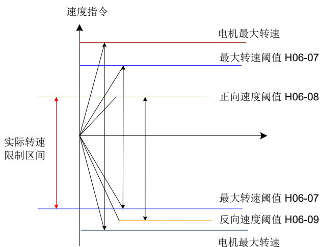
图 5-72 速度指令限幅举例说明
