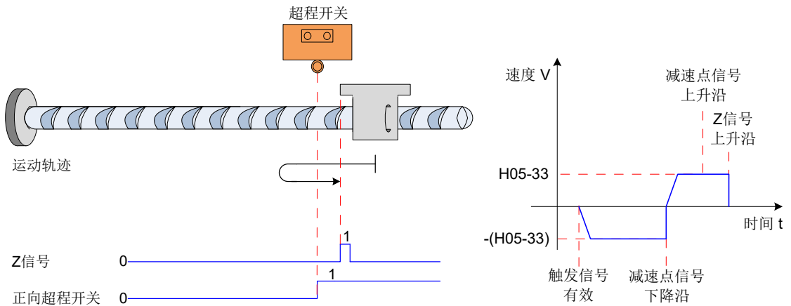
图 5-52 模式 8 原点回零电机运行曲线②与转速说明
