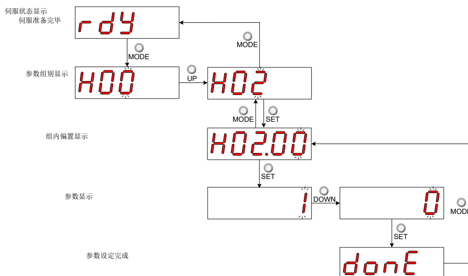
图 4-5 参数设定步骤示意图
