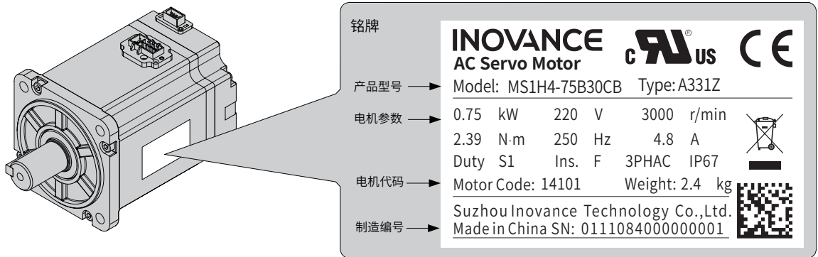
图 1-4 伺服电机型号与铭牌说明
