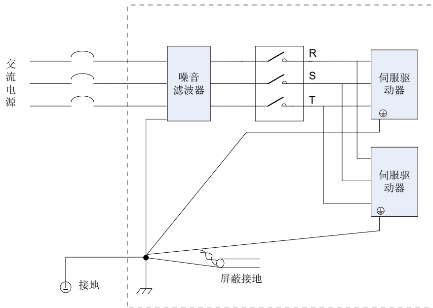
图 3-37 噪音滤波器地线处理示意图
