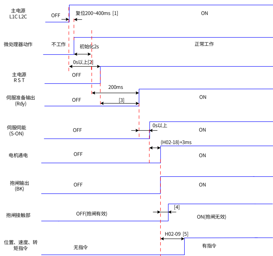
图 5-7 电源接通时序图
