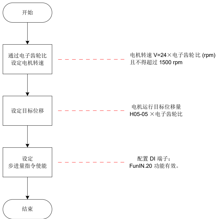
图 5-22 步进量指令来源设置流程
