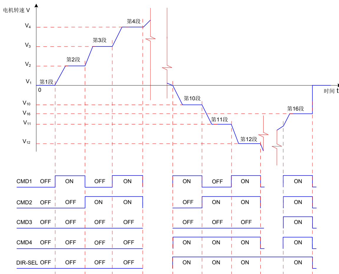
图 5-68 多段速度曲线举例
