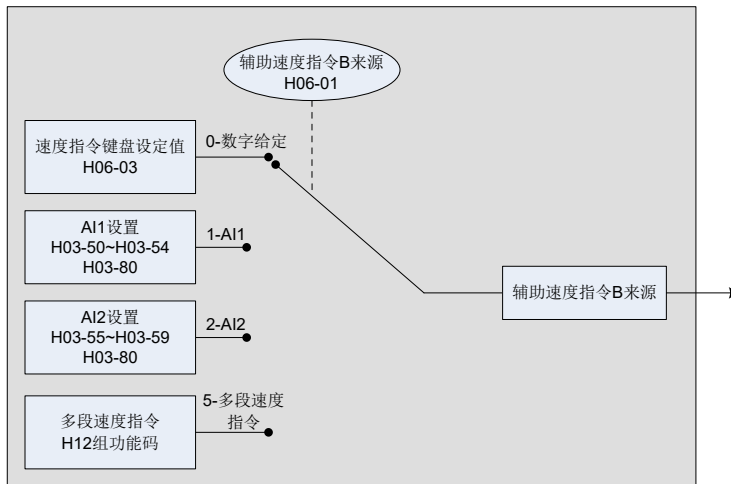
图 5-66 辅助速度指令 B 来源图
