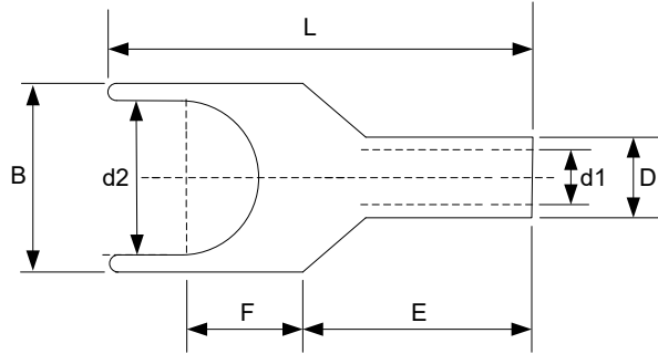
图 3-6 TNS 系列线耳尺寸图
