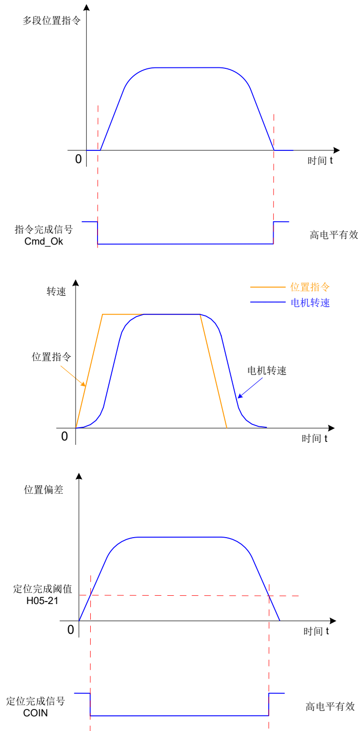
图 5-35 定位完成 / 接近功能说明
