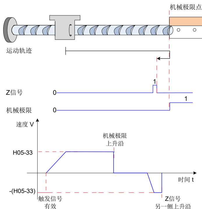
图 5-54 模式 12 原点回零电机运行曲线与转速说明
