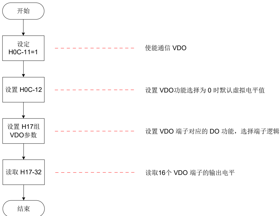
图 7-19 VDO 使用流程图
