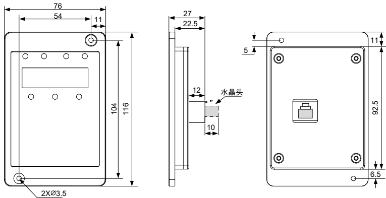
图 2-7 MD32NKE1 外引操作面板尺寸 (单位：mm)
