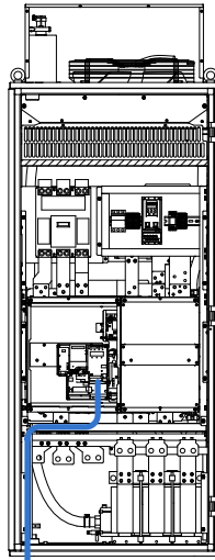
图 4-10 控制回路线缆布放示例 表 4-7 线缆选型指导
