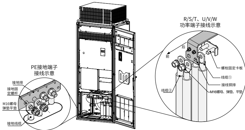
图 4-9 主回路端子和 PE 接地端子接线示例
