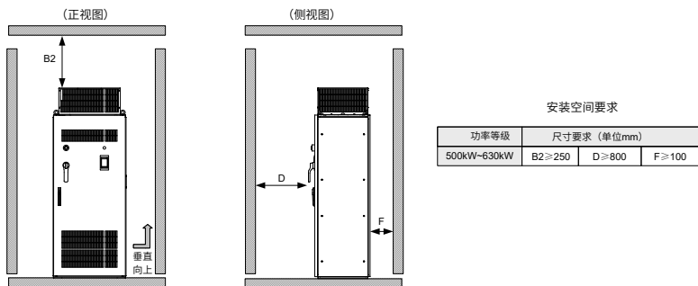
图 3-2 安装空间要求
