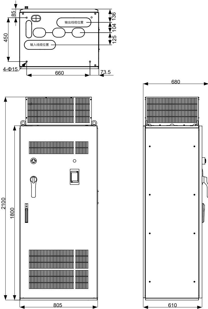
图 1-5 MD290T500G~MD290T630G、MD290T560P~MD290T800P (标准机柜) 安装尺寸示意图 (单位: mm)
