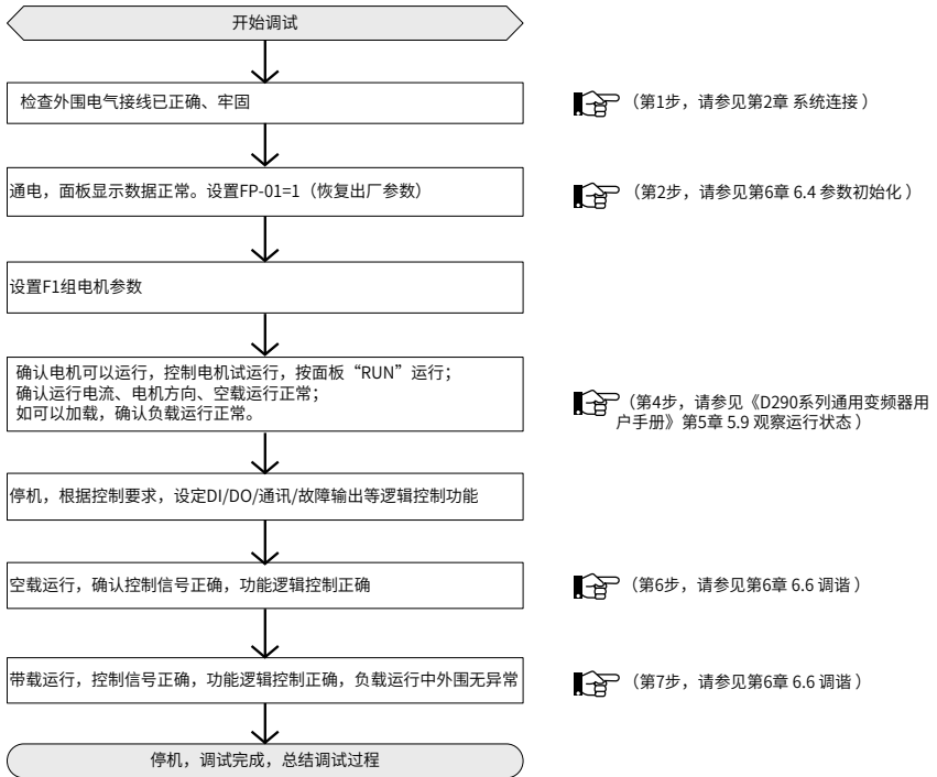
图 6-1 快速调试步骤指南
