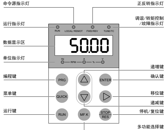
图 5-1 面板各部分名称
