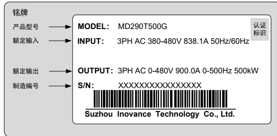
图 1-1 产品铭牌
