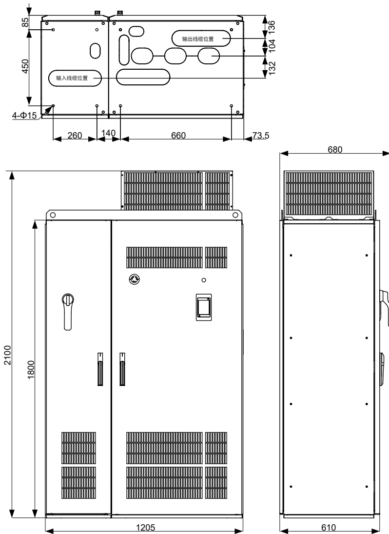
图 1-6 MD290T500G~MD290T630G、MD290T560P~MD290T800P (带辅助配电柜) 安装尺寸示意图 (单位: mm)
