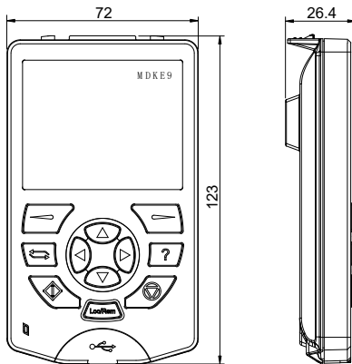
图 2-9 MDKE9 外引操作面板尺寸 (单位: mm)
