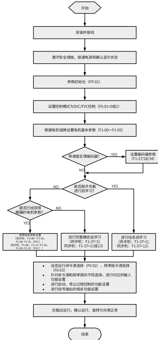
图2-3 变频器调试流程图 (SVC/FVC)
