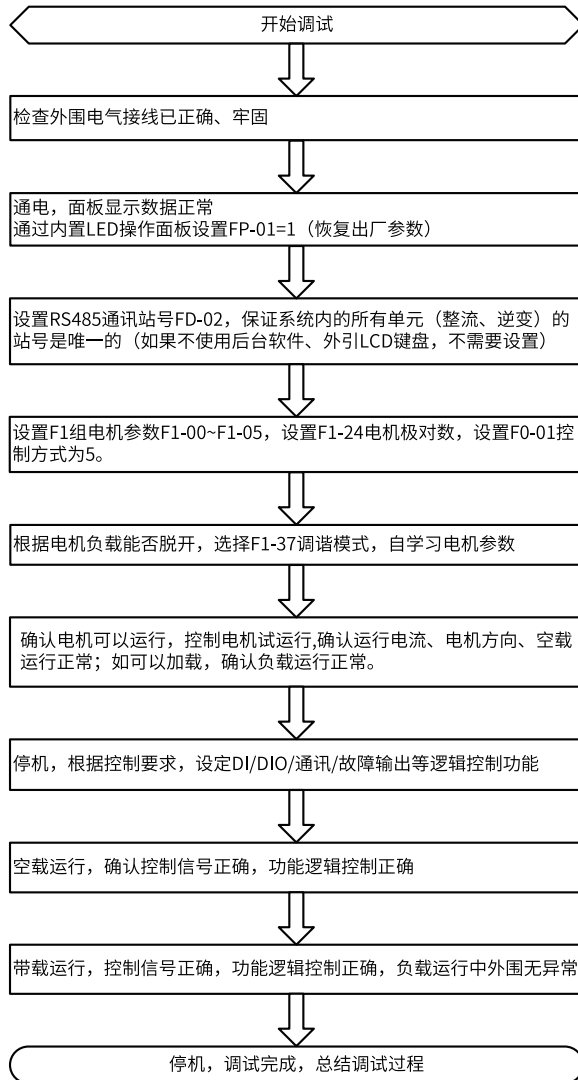
图2-6 调试流程图
