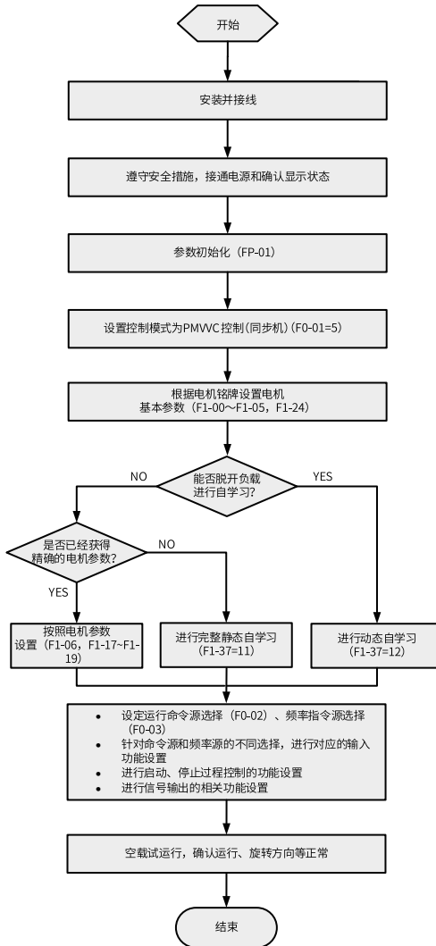
图2-4 变频器调试流程图 (PMWVC控制)
