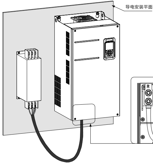
图9-1 EMC滤波器安装示意图
