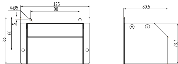
图1-9 T2机型导风罩尺寸 (单位: mm)
