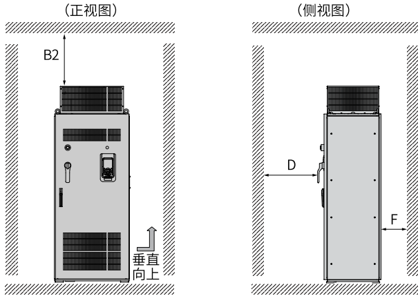
图1-15 安装空间要求
