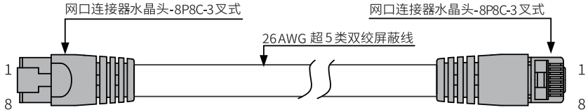
图8-67 EtherCAT网线制作要求
