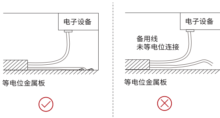
图8-57 多芯电缆有芯线剩余时的处理方法示意图
