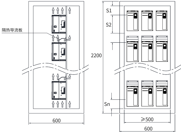
图4-1 多层安装最小保证空间 (单位: mm)
