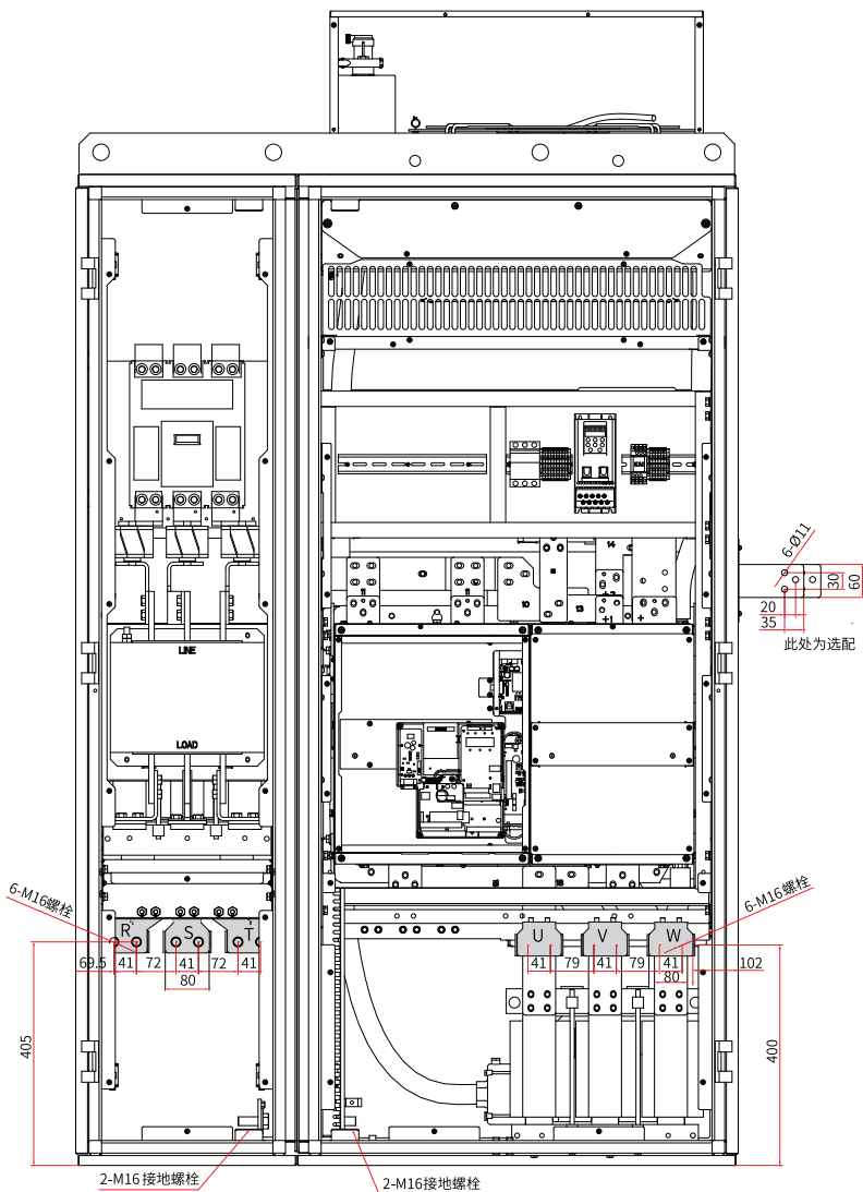
图8-27 T13机型主回路端子尺寸（带辅助配电柜）（三相380V-480V）
