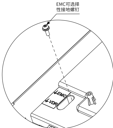
图8-31 断开EMC可选择性接地螺钉
