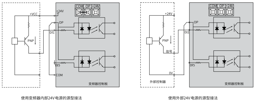
图8-41 源型接线方式
