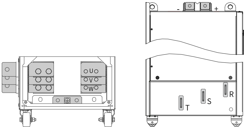
图8-7 T10~T12主回路端子分布图
