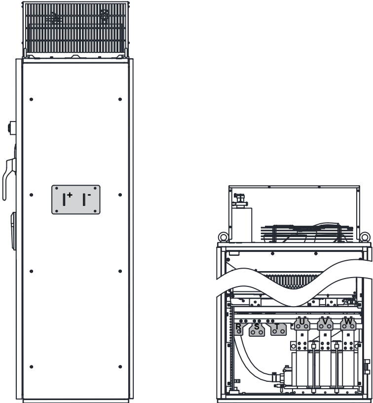
图8-8 T13主回路端子分布图
