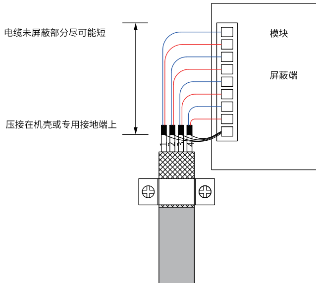
图8-60 屏蔽线处理要求示意图
