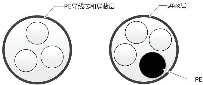
图8-28 推荐的动力线缆类型
