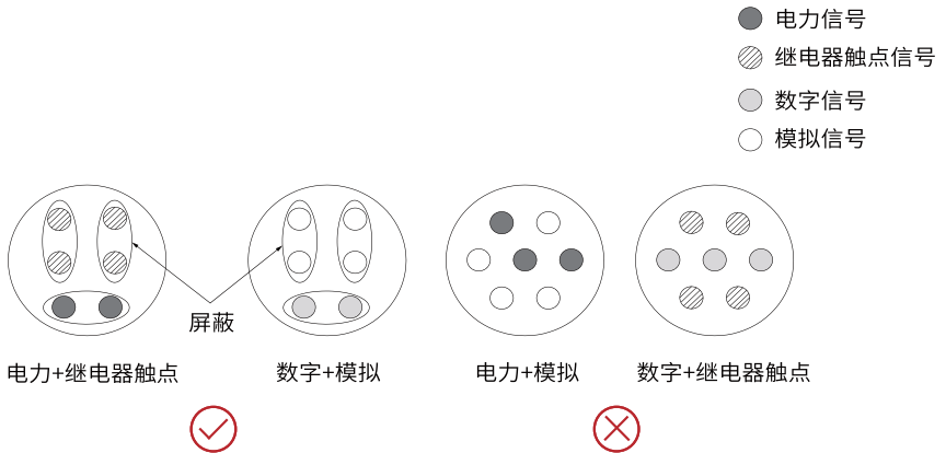
图8-56 多芯电缆布线示意图
