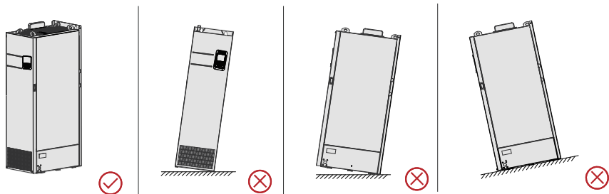
图1-17 安装方向示意图 (T10~T12)
