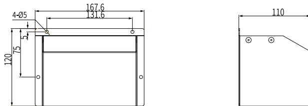
图1-12 T5机型导风罩尺寸 (单位: mm)
