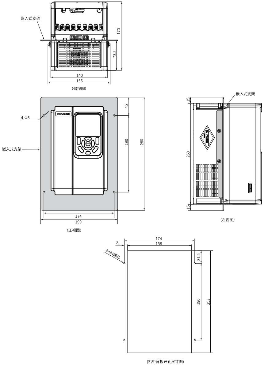
图1-21 MD500-AZJ-A1T3中部安装支架及开孔尺寸 (mm)
