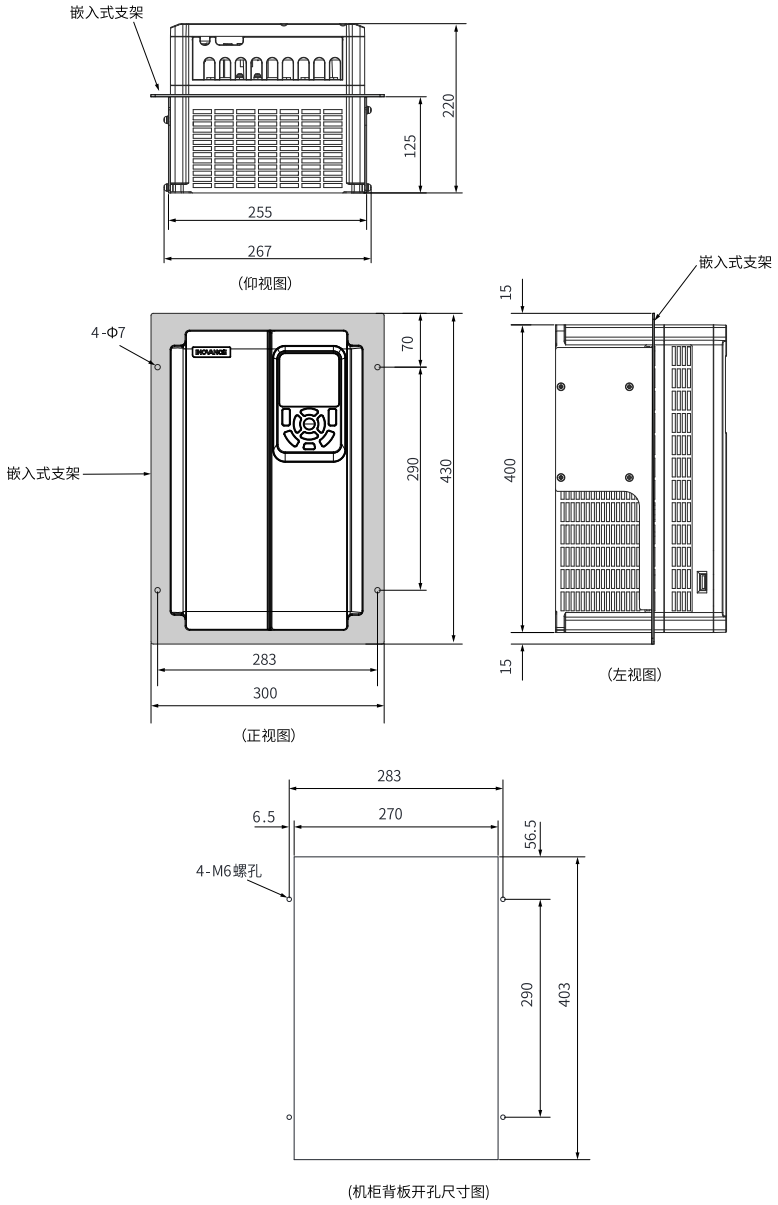
图1-24 MD500-AZJ-A1T6嵌入式安装支架及开孔尺寸 (mm)
