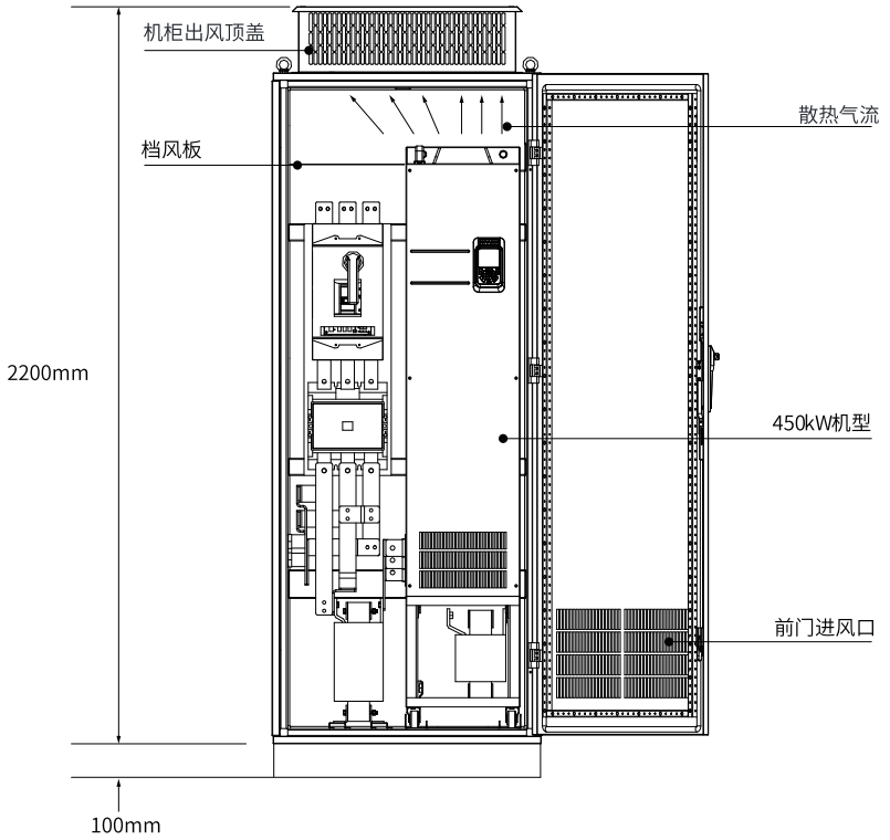
图5-1 直排风机柜示意图
