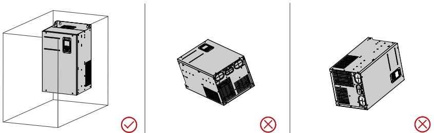
图1-16 安装方向示意图 (T1~T9)
