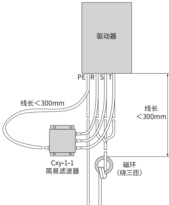
图10-2 输入侧加装简易滤波器、磁环示意图
