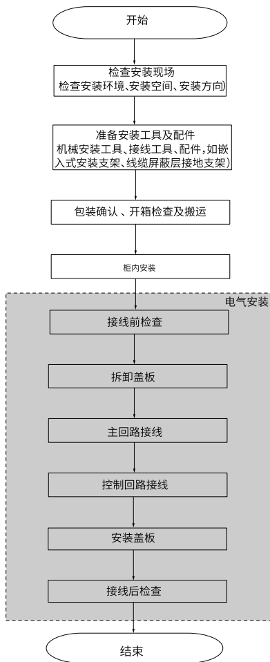
图1-2 安装总流程 (T10~T12机型)
