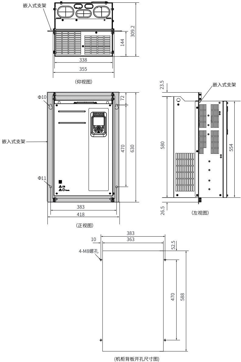
图1-26 MD500-AZJ-A1T8嵌入式安装支架及开孔尺寸 (mm)
