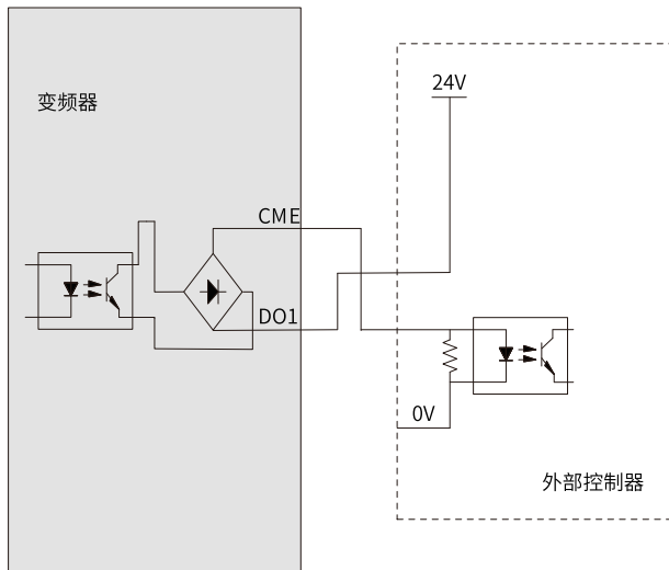
图8-46 数字输出端子接外部控制器2
