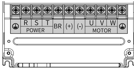
图8-5 T5~T8机型主回路端子分布图
