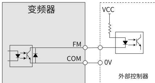
图8-47 高速数字输出端子接线示意图
