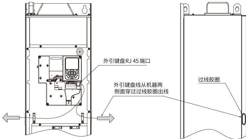
图8-50 外引操作面板线缆走线示意图
