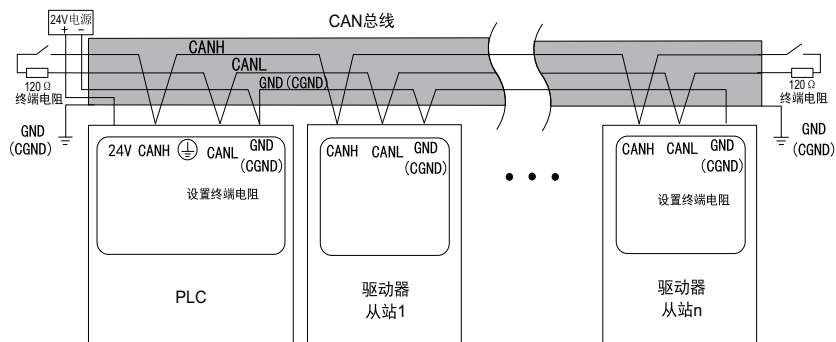
图8-66 CAN总线连接拓扑结构
