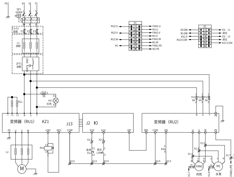
图8-2 柜内电气图 (T13机型)
