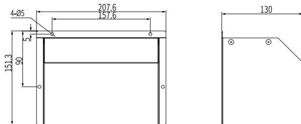
图1-13 T6机型导风罩尺寸 (单位: mm)
