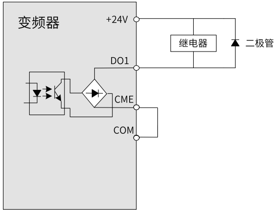
图8-42 数字输出端子接继电器示意图
