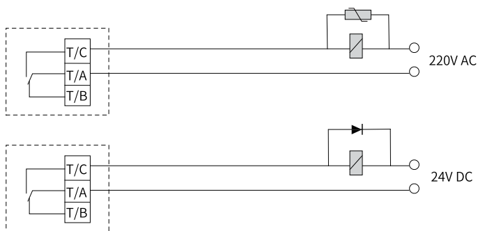
图8-48 继电器输出端子抗干扰处理
