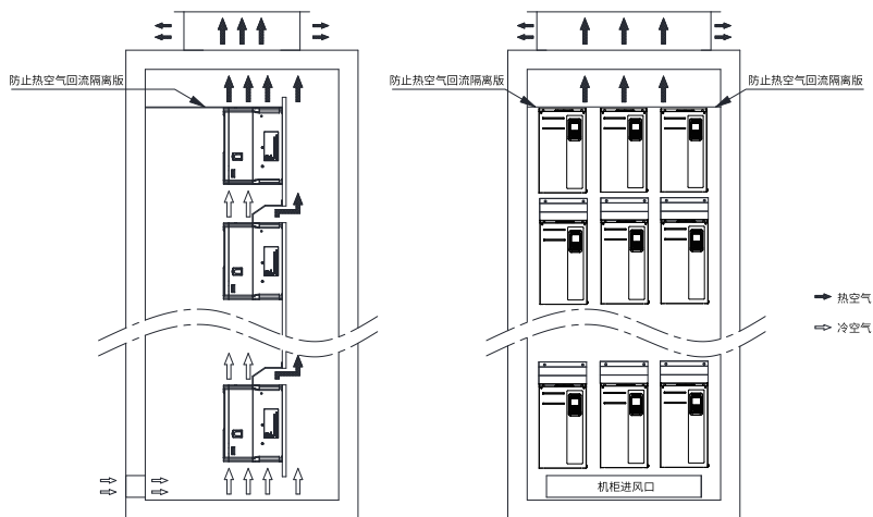
图4-5 被动排风机柜内热空气回流示意图 (有隔离装置)
