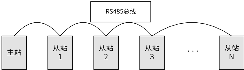
图8-64 菊花链连接方式
