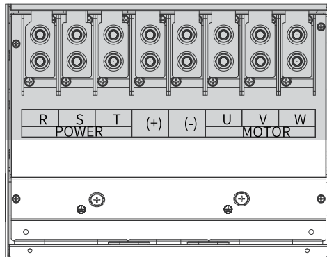
图8-6 T9机型主回路端子分布图
