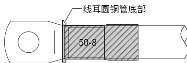
图8-34 线缆导体加套管热缩示意图
