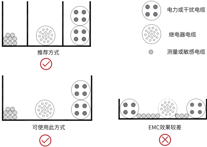
图8-59 多类电缆铺设方法示意图
