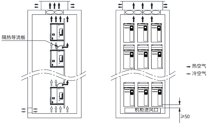
图4-3 机柜进风口开孔位置示意图
