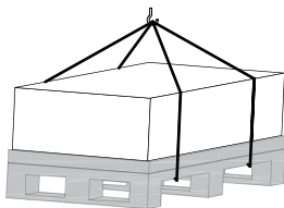
图3-1 设备起吊示意图
