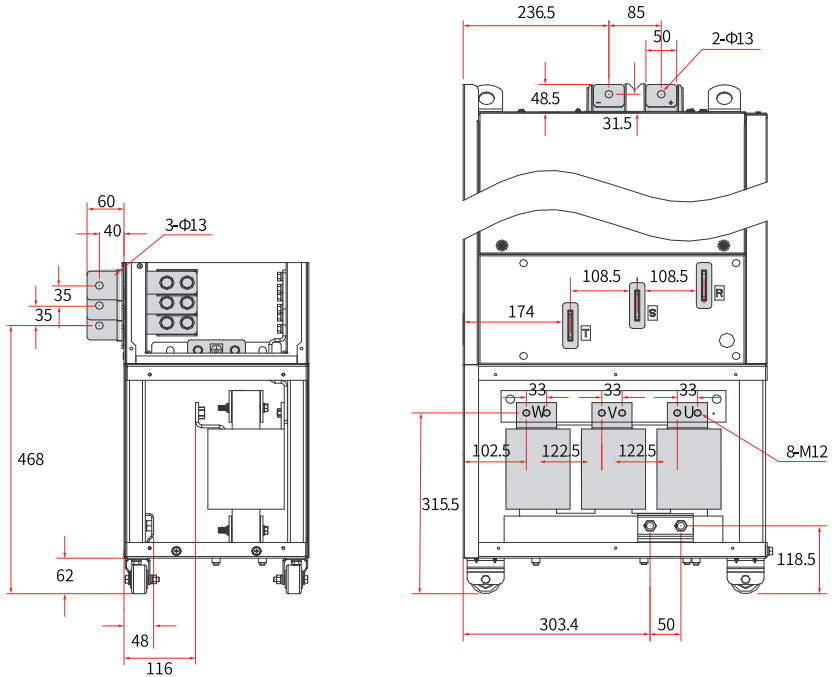
图8-18 T10机型主回路端子尺寸（带输出电抗器）（mm）
