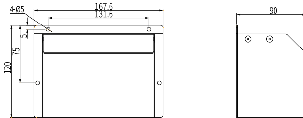
图1-11 T4机型导风罩尺寸 (单位: mm)
