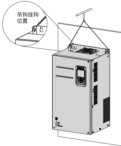
图3-12 起吊示意图
