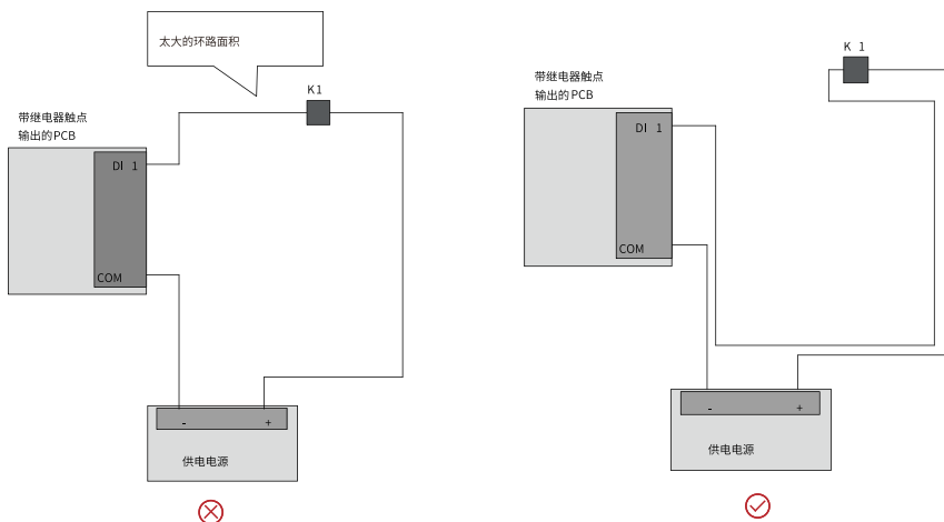
图8-58 避免布线环路过大示意图
