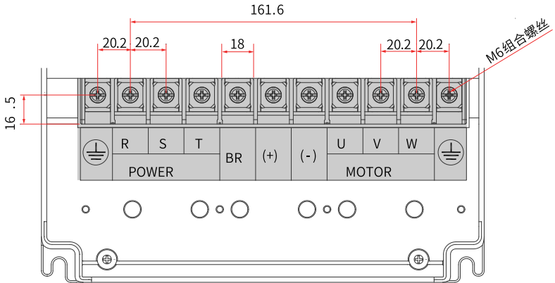
图8-13 T6机型主回路端子尺寸 (mm)
