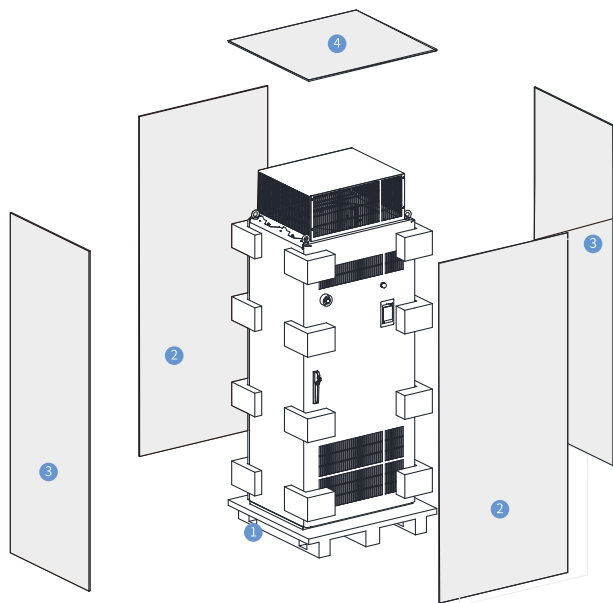
图3-16 包装拆卸示意图
