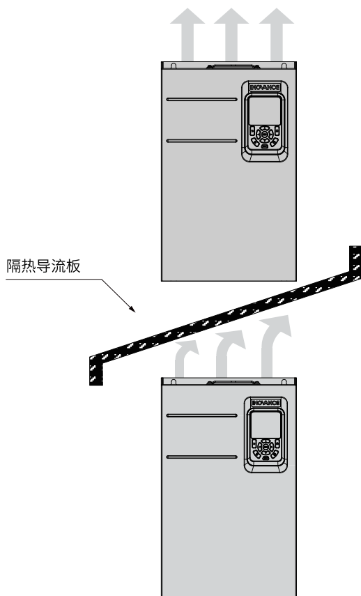
图1-6 上下排安装要求
