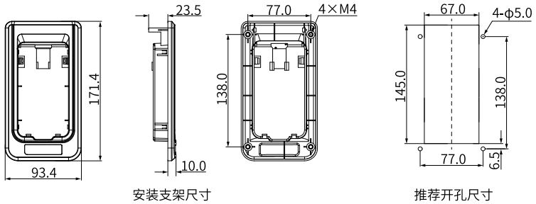
图9-4 MDKE-10键盘底座安装支架尺寸及开孔尺寸（单位：mm）
