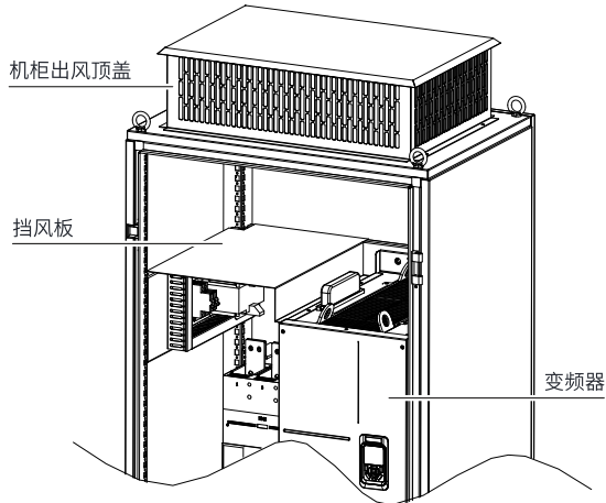
图5-3 机柜挡风板示意图
