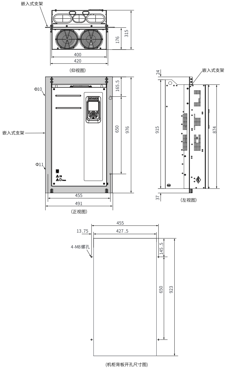
图1-27 MD500-AZJ-A1T9嵌入式安装支架及开孔尺寸 (mm)
