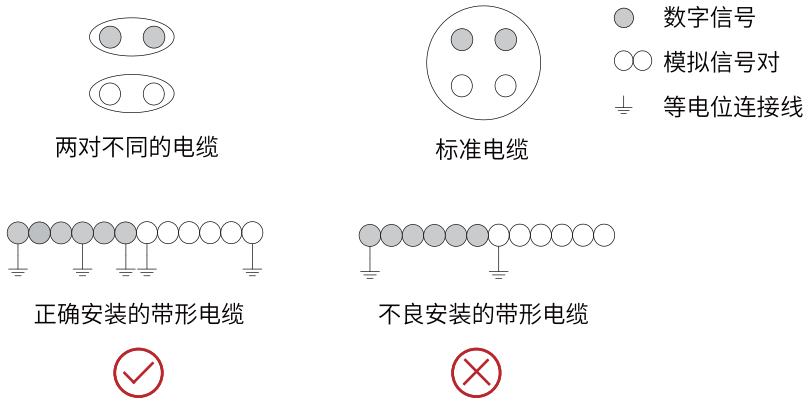
图8-55 不同类型信号电缆布线示意图
