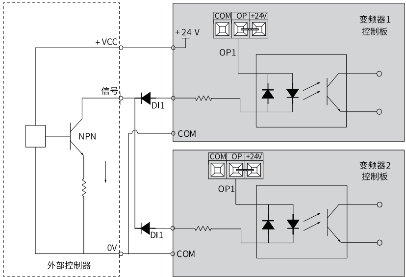
图8-40 多台变频器DI端子并接漏型接线方式
