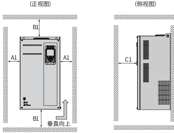
图1-4 单台机器 (T1~T9) 安装空间
