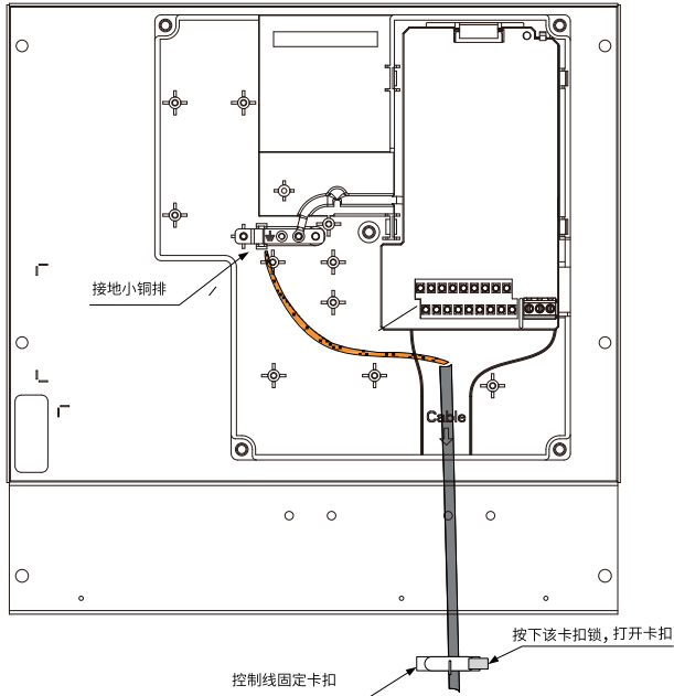
图8-52 模拟量端子的屏蔽层接地示意图
