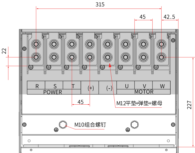
图8-16 T9机型主回路端子尺寸 (mm)
