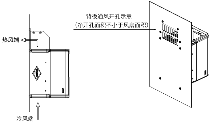
图1-7 导风罩整机装备图
