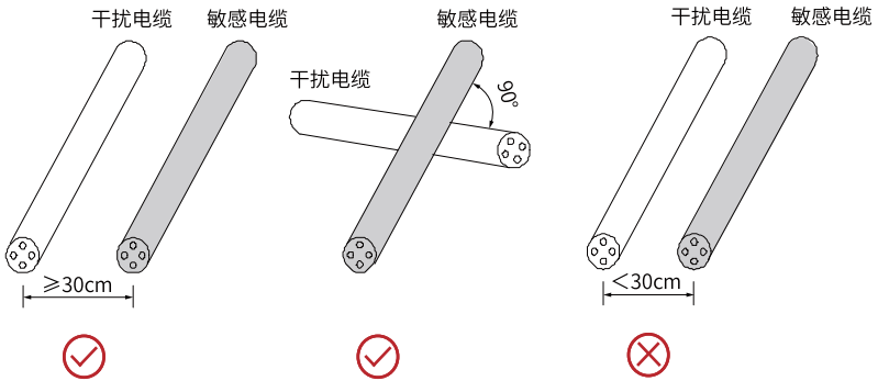
图8-54 干扰电缆与敏感电缆布线示意图
