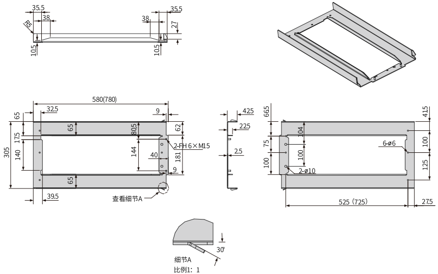
图1-28 T10底部安装支架尺寸
