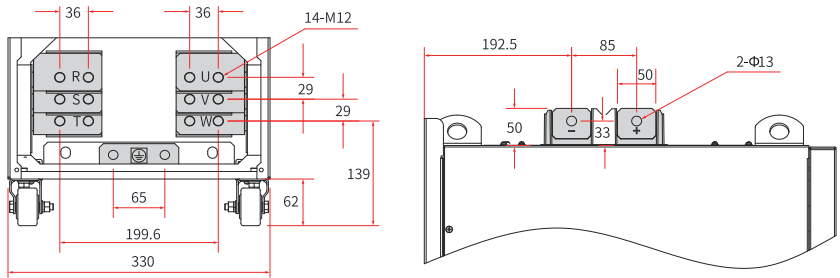
图8-22 T11机型主回路端子尺寸（不带侧出铜排，不带输出电抗器）（mm）
