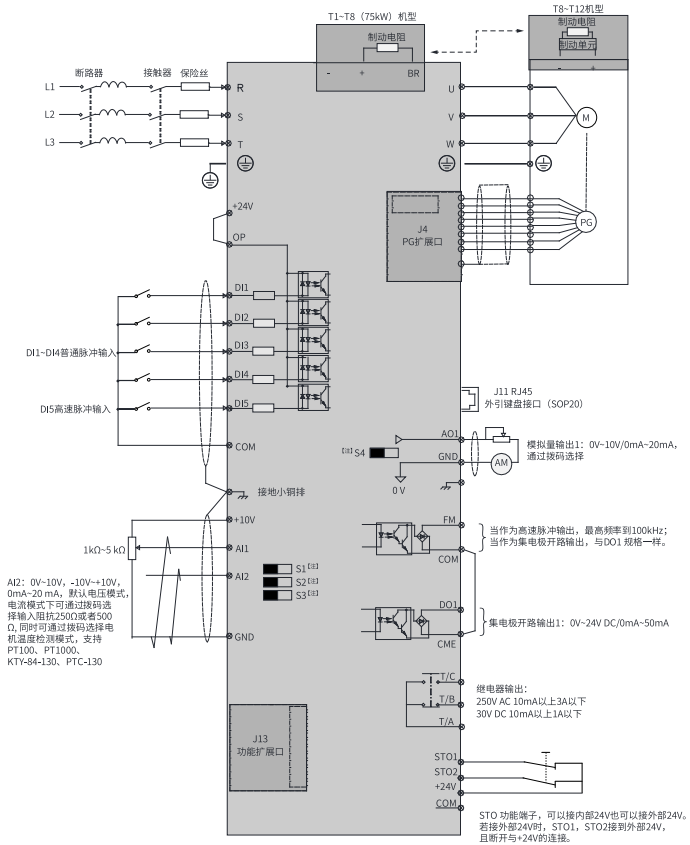
图8-1 标准接线图 (T1-T12)
