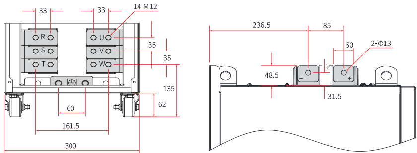
图8-19 T10机型主回路端子尺寸（不带侧出铜排，不带输出电抗器）（mm）
