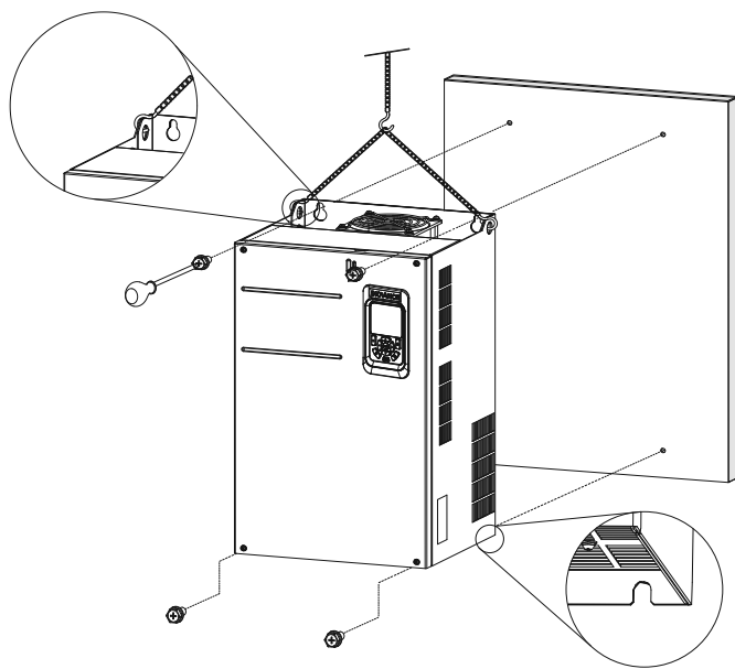
图4-9 T7~T9机型壁挂式安装示意图
