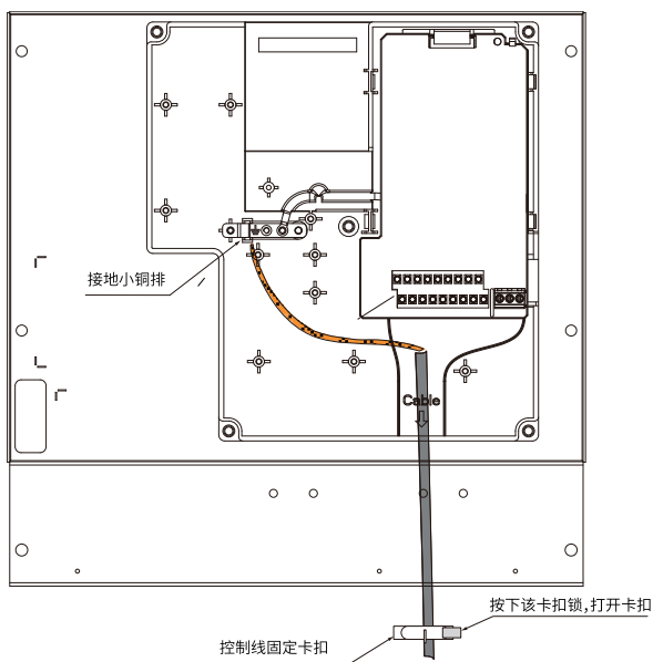
图8-37 模拟量端子的屏蔽层接地示意图
