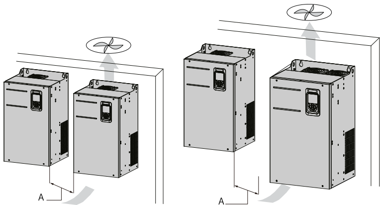
图1-5 多台机器 (T1~T9) 并排安装
