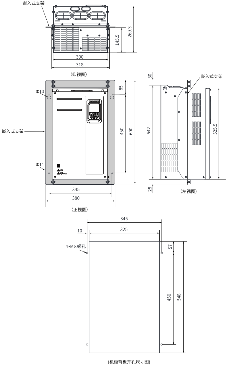
图1-25 MD500-AZJ-A1T7嵌入式安装支架及开孔尺寸 (mm)
