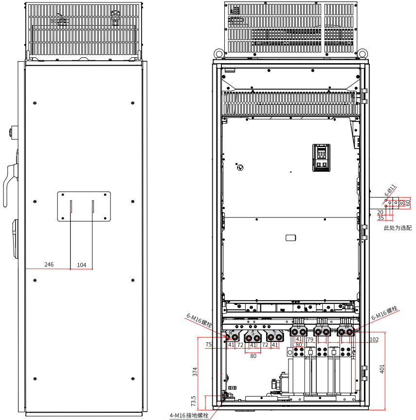
图8-26 T13机型主回路端子尺寸（不带辅助配电柜）（三相380V-480V）
