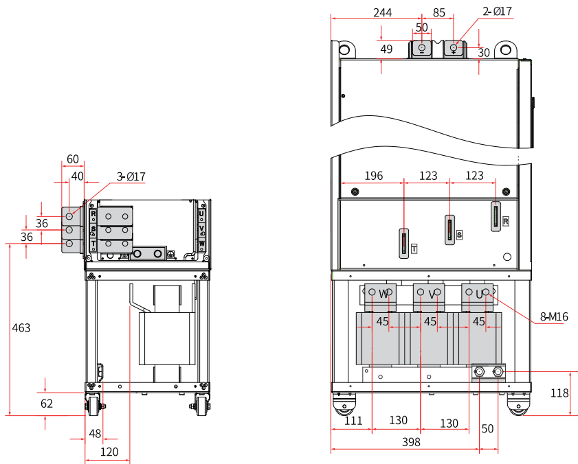
图8-24 T12机型主回路端子尺寸（带输出电抗器）（mm）
