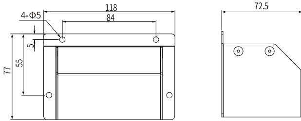
图1-8 T1机型导风罩尺寸 (单位: mm)
