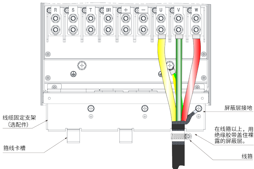
图8-32 屏蔽层接线示意图
