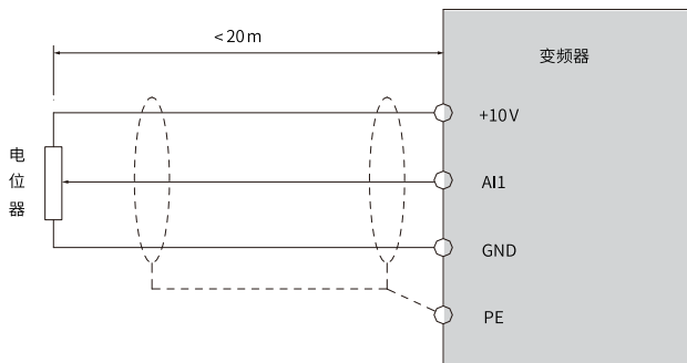
图8-36 模拟量输入端子接线示意图
