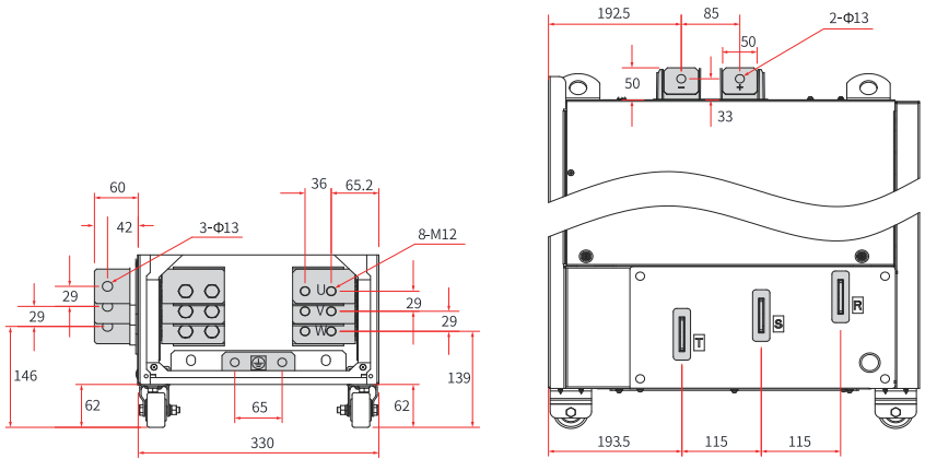
图8-20 T11机型主回路端子尺寸（不带输出电抗器）（mm）
