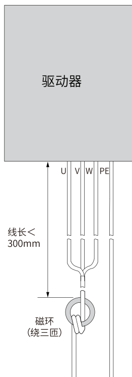
图9-2 磁环安装示意图
