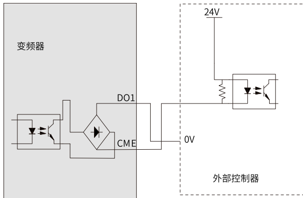
图8-44 数字输出端子接外部控制器2
