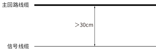
图8-30 线缆布线图
