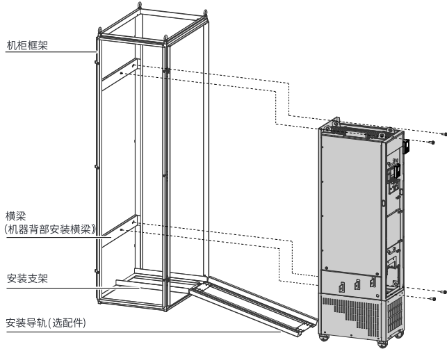
图5-12 固定到安装横梁示意图
