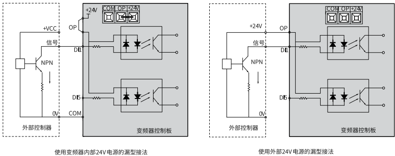
图8-39 漏型接线方式
