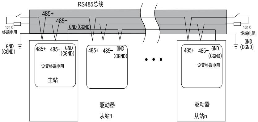
图8-65 RS485总线连接拓扑结构
