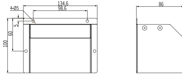
图1-10 T3机型导风罩尺寸 (单位: mm)
