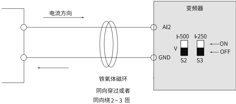
图8-38 模拟量AI2/AI3输入端子处理接线图
