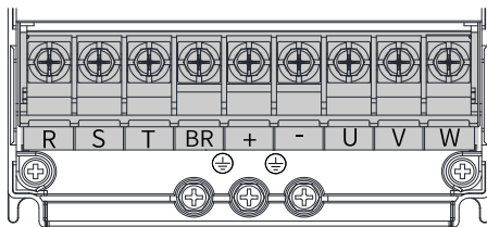
图8-3 T1~T4机型主回路端子分布图（三相）
