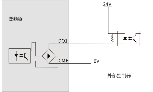
图8-43 数字输出端子接外部控制器1
