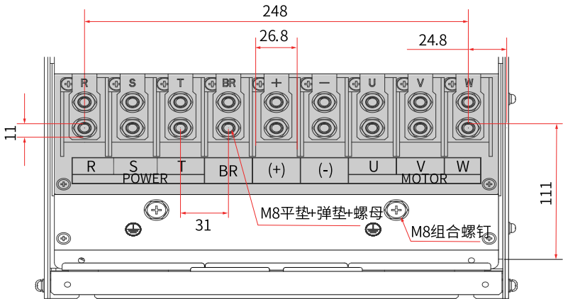
图8-14 T7机型主回路端子尺寸 (mm)
