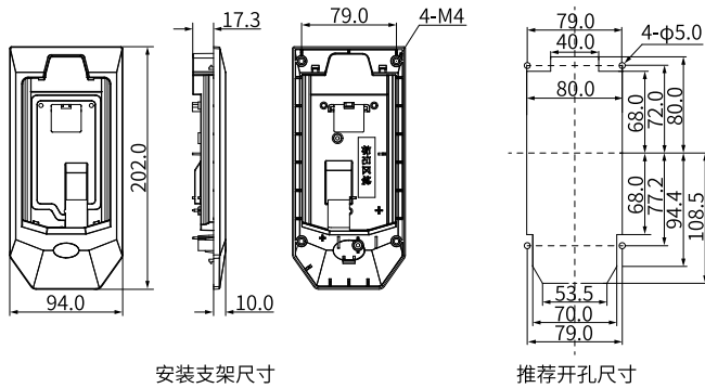
图9-5 SOP-20-810 键盘安装底座支架尺寸及开孔尺寸（单位：mm）
