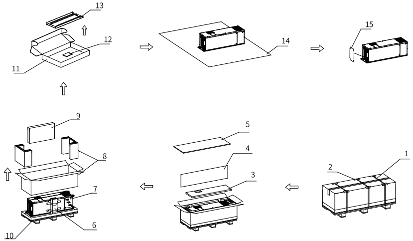
图3-7 T10机型包装清单
