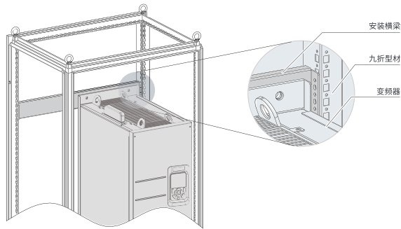
图5-6 T11~T12机型机柜3D示意图
