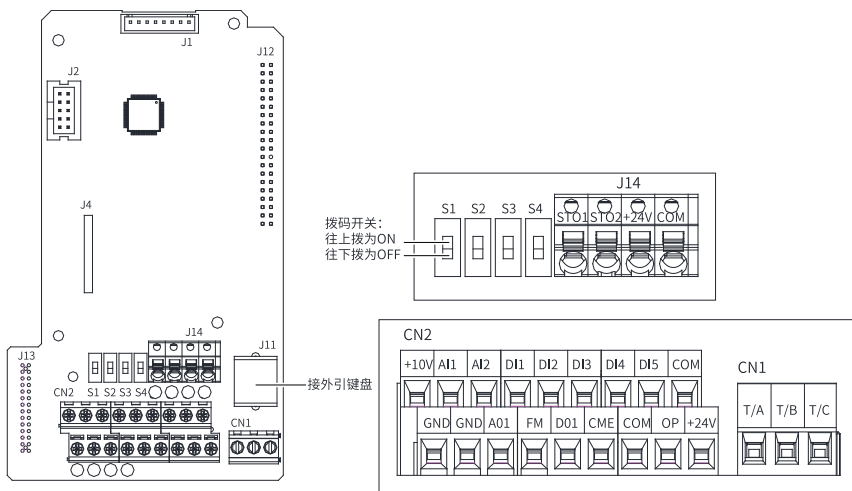
图8-35 控制回路端子分布图
