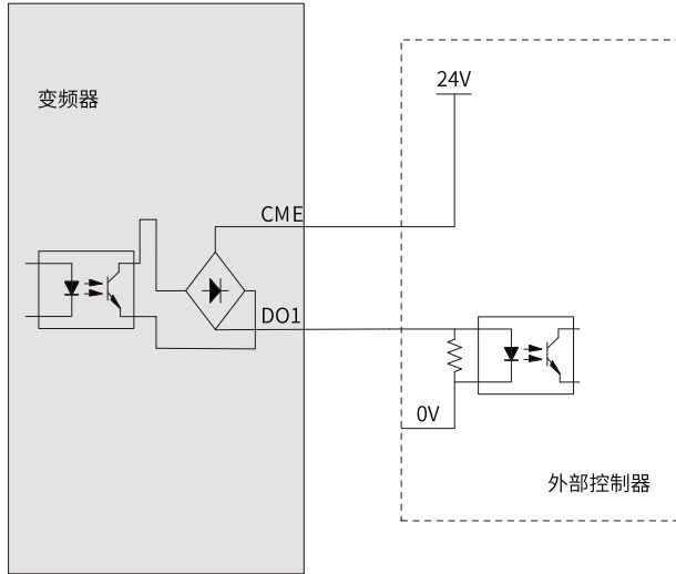
图8-45 数字输出端子接外部控制器3
