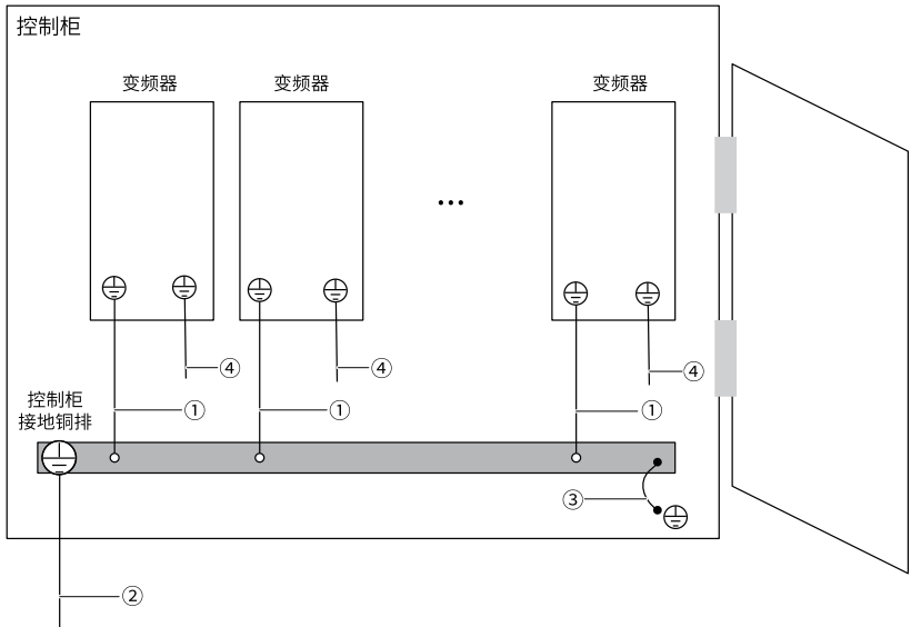
图8-62 多机并联接地示意图
