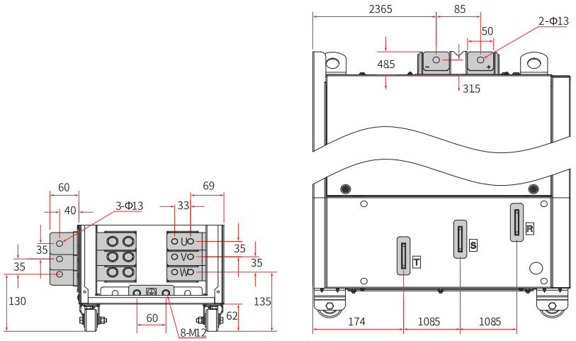
图8-17 T10机型主回路端子尺寸（不带输出电抗器）（mm）
