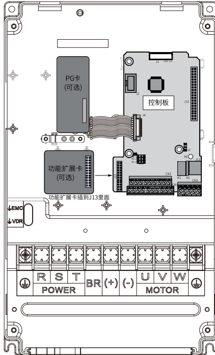
图4-10 控制板位置
