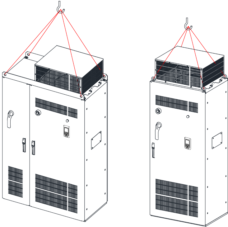
图3-15 包装拆封后搬运示意图
