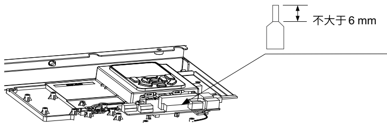
图8-49 控制线管状端子要求
