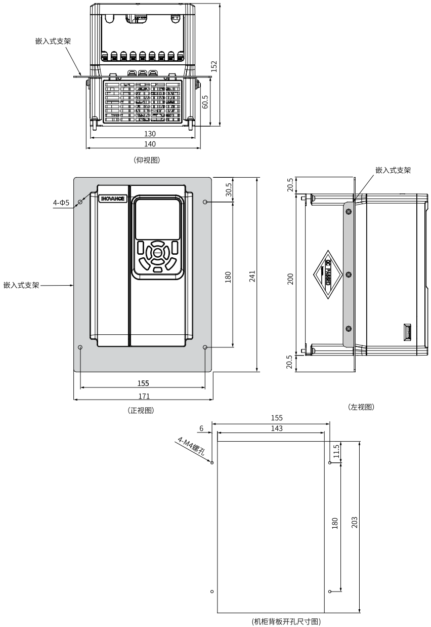
图1-19 MD500-AZJ-A1T1中部安装支架及开孔尺寸 (mm)
