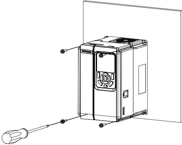
图4-8 T1~T6机型壁挂式安装示意图
