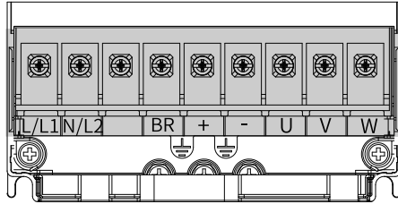
图8-4 T2机型主回路端子分布图（单相）
