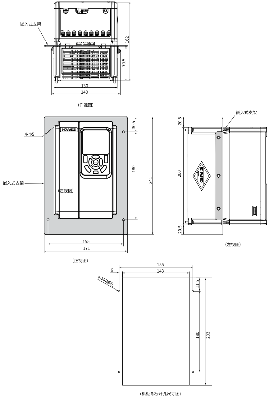
图1-20 MD500-AZJ-A1T2中部安装支架及开孔尺寸 (mm)
