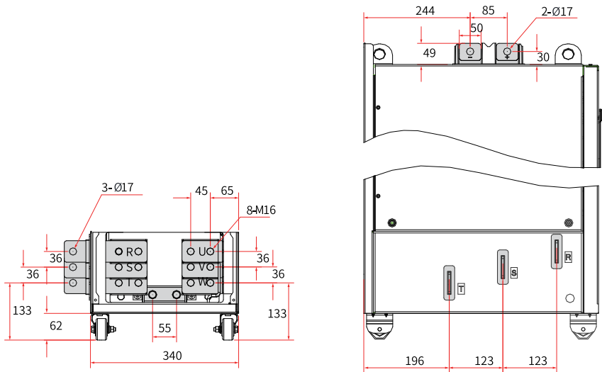
图8-23 T12机型主回路端子尺寸（不带输出电抗器）（mm）
