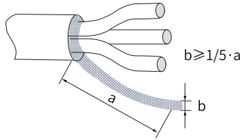
图8-33 电机线缆“屏蔽层”引出示意图
