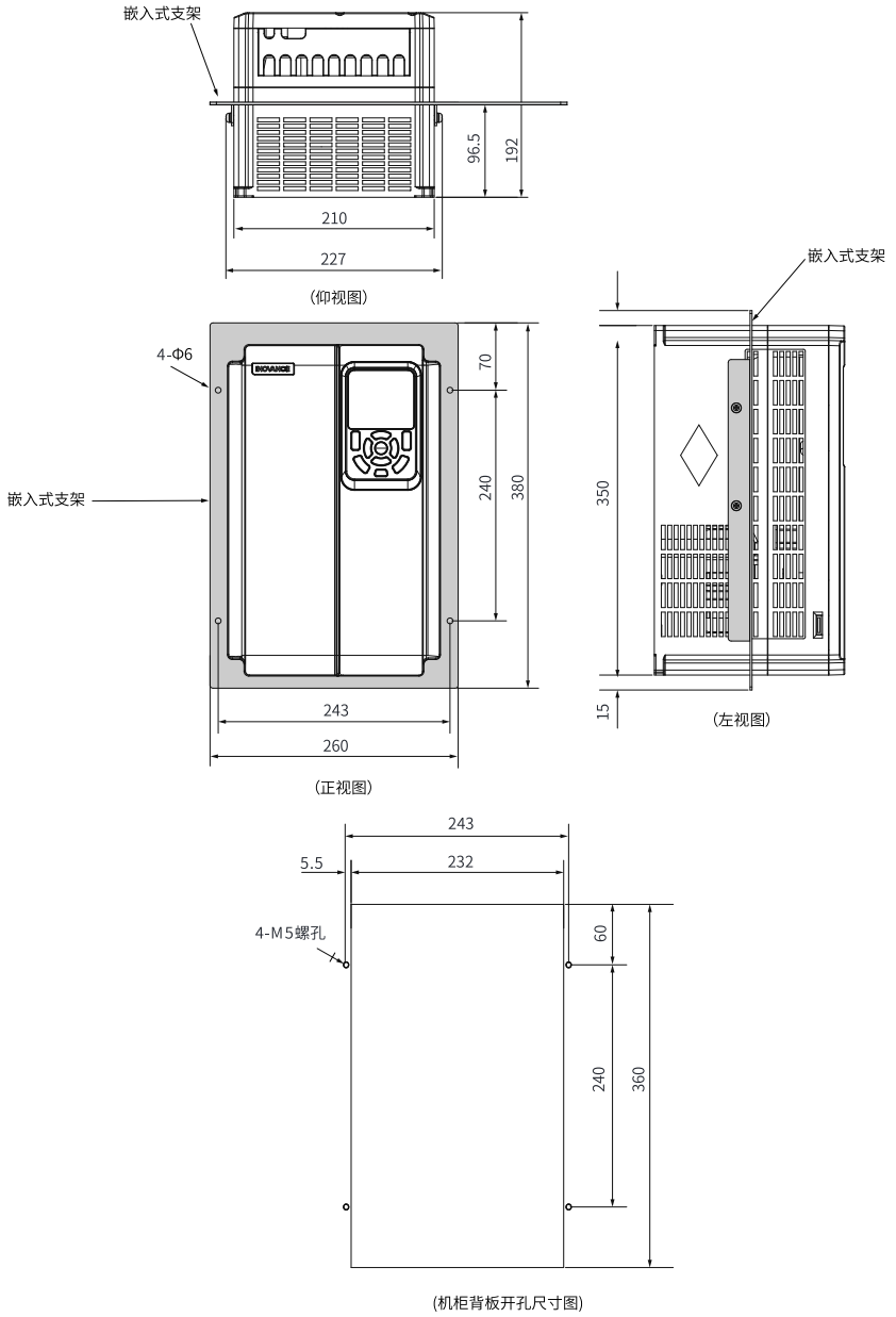
图1-23 MD500-AZJ-A1T5嵌入式安装支架及开孔尺寸 (mm)
