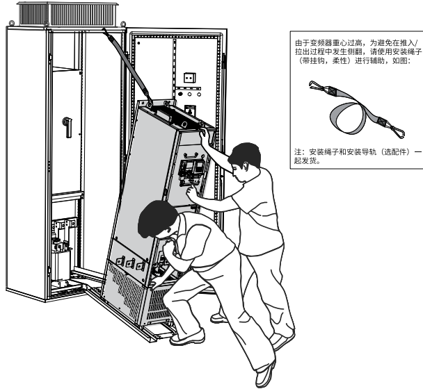
图5-11 推入机柜示意图
