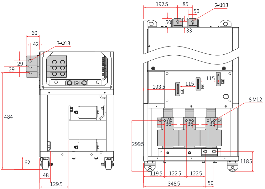
图8-21 T11机型主回路端子尺寸（带输出电抗器）（mm）
