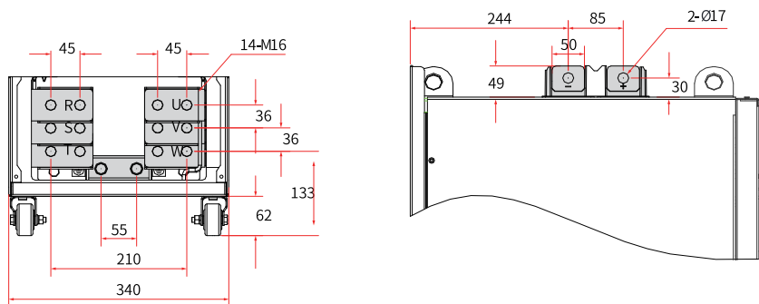
图8-25 T12机型主回路端子尺寸（不带侧出铜排，不带输出电抗器）（mm）
