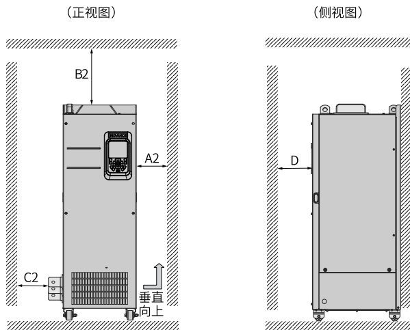
图1-14 安装空间要求
