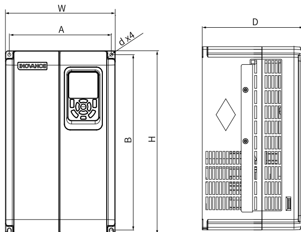
图2-2 T5~T6外型尺寸及安装尺寸示意图
