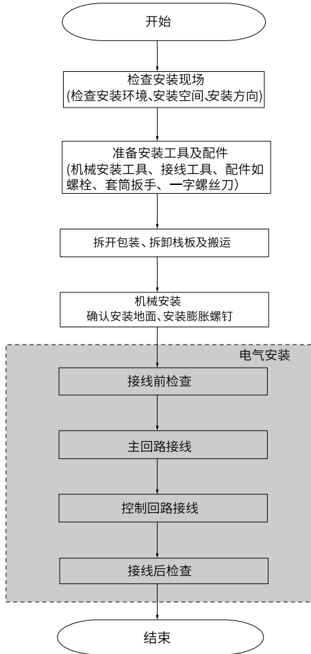
图1-3 安装总流程（T13机型）
