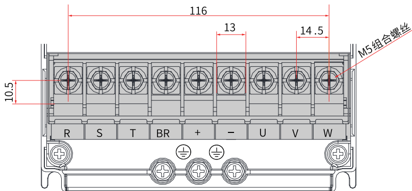
图8-10 T3机型主回路端子尺寸 (mm)
