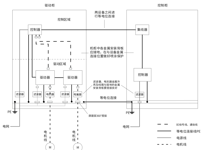
图8-63 推荐的机柜系统接线
