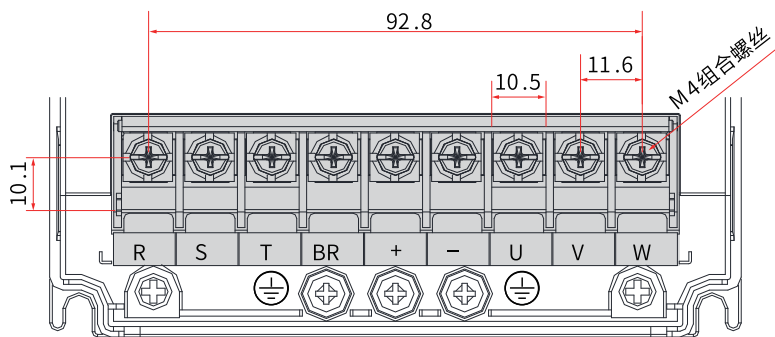
图8-9 T1~T2机型主回路端子尺寸 (mm)
