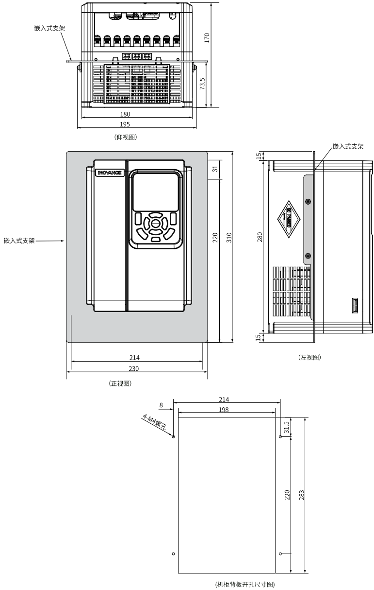
图1-22 MD500-AZJ-A1T4中部安装支架及开孔尺寸 (mm)
