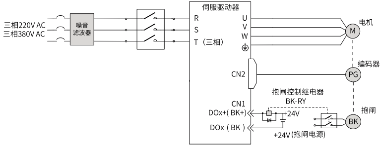
图3-7 抱闸接线示意图
