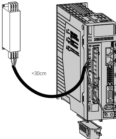
图2-2 EMC滤波器连接示意图
