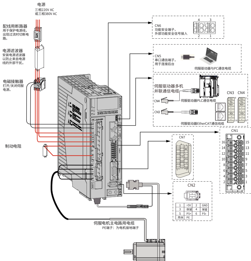
图1-2 三相220V或三相380V系统配线图举例
