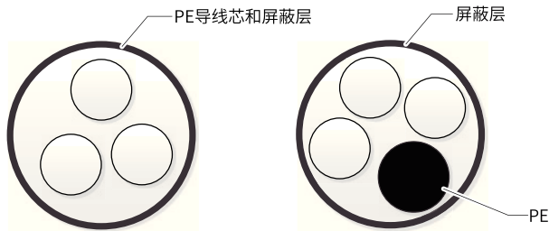
图2-6 推荐的动力线缆类型
