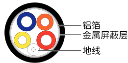
图3-13 推荐线缆示意图
