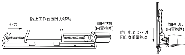
图3-6 抱闸应用示意图
