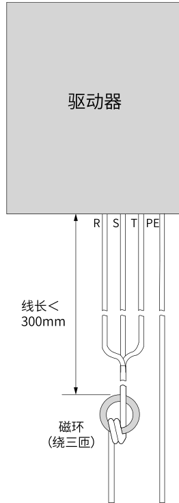
图5-1 输入侧加磁环
