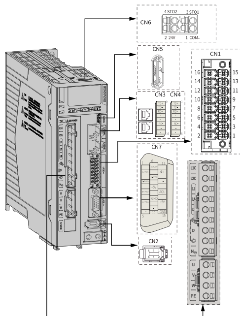
图3-1 伺服驱动器端子引脚分布示意图
