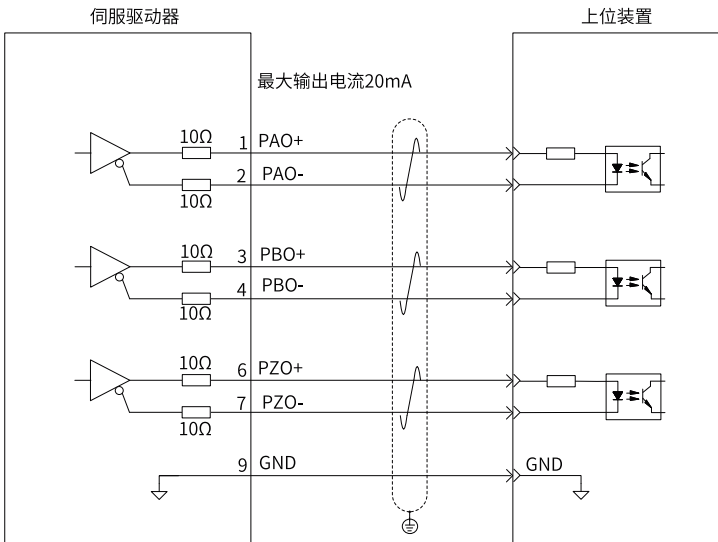
图3-15 光耦接收电路示例图
