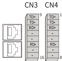
图3-11 伺服驱动器通信端子引脚分布示意图
