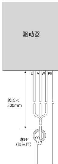
图2-3 磁环的连接示意图
