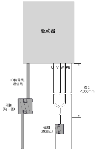
图2-4 磁扣的连接示意图
