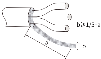
图2-8 电机线缆屏蔽层引出示意图
