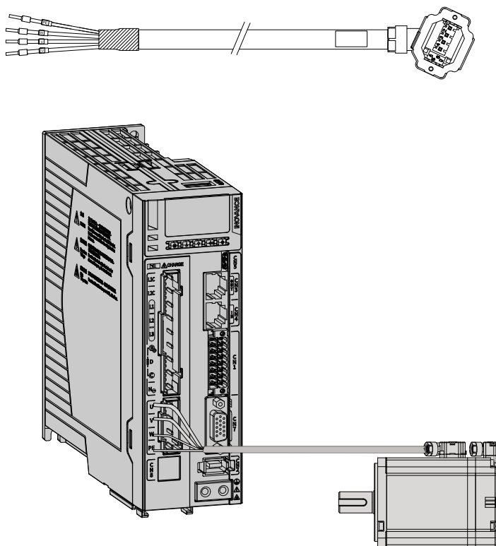
图3-4 伺服驱动器输出与伺服电机连接示意图
