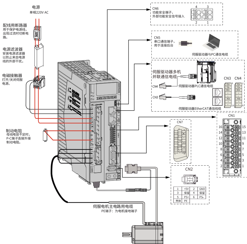
图1-1 单相220V系统配线图举例
