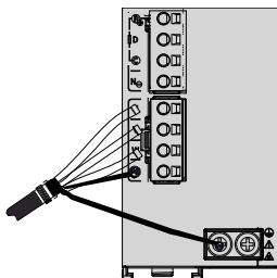
图2-7 屏蔽层搭接示意图
