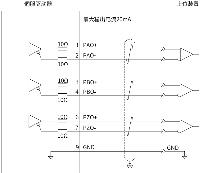
图3-14 差分接收电路示例图
