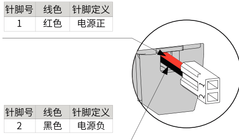
图3-10 绝对值编码器电池外引线说明
