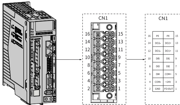
图3-5 伺服驱动器控制端子（CN1）引脚分布示意图
