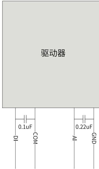
图5-2 IO信号线上加大滤波
