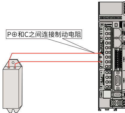
图3-16 外接制动电阻连接示意图
