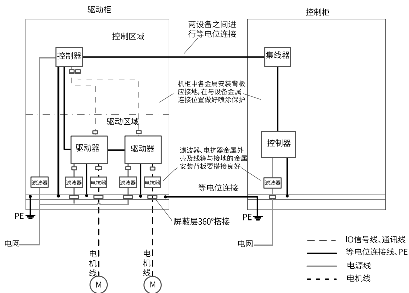
图2-11 推荐的控制柜系统接线
