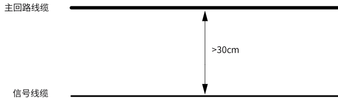
图2-10 线缆布线图
