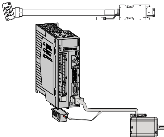
图3-9 绝对值编码器信号 [1] 接线示例图
