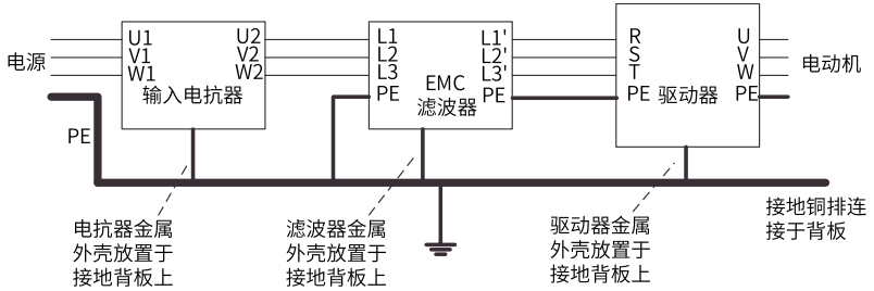
图2-1 交流输入电抗器连接示意图
