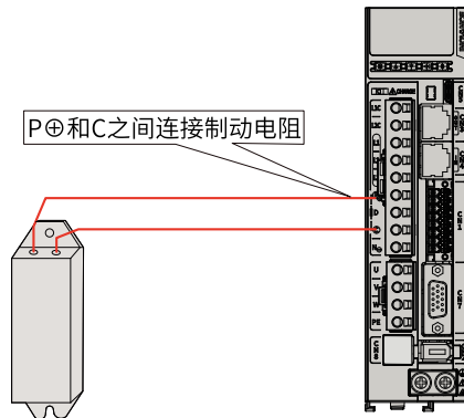
图2-5 外接制动电阻连接示意图
