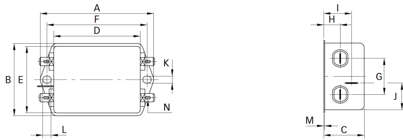
图4-3 FN2090系列滤波器尺寸图(单位: mm)
